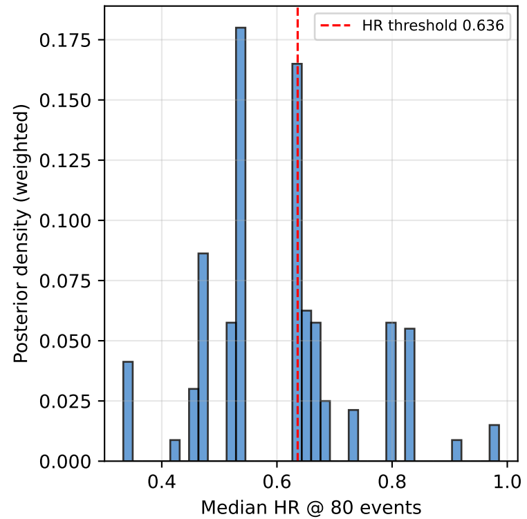
Final-HR posterior
