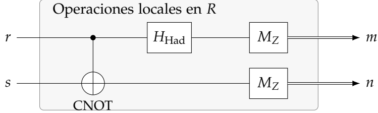
Figura 3: Circuito de la medición de Bell sobre r, s . El tiempo avanza hacia la derecha. M_Z denota una medición en la base computacional; las líneas dobles transportan los resultados clásicos. Los qubits de Alice y Bob no intervienen en estas compuertas.
