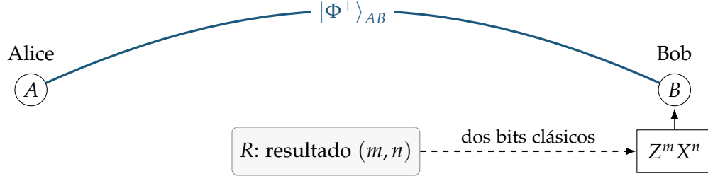
Figura 4: Situación final, después de comunicar el resultado y aplicar la corrección. La línea gruesa representa el nuevo par entrelazado AB ; la flecha discontinua representa el mensaje clásico. Los dos enlaces iniciales se han consumido.
