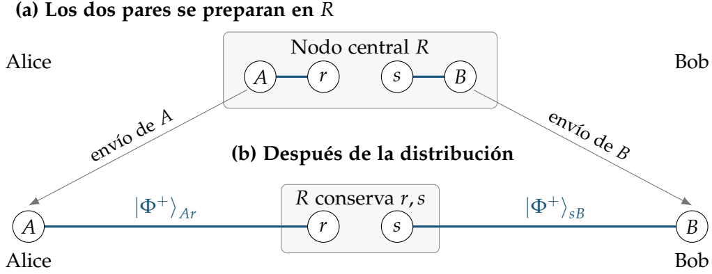
Figura 2: Preparación y envío desde la estación central. Las líneas gruesas representan pares entrelazados; las flechas grises representan el transporte de qubits. Las líneas de entrelazamiento no son trayectorias de partículas.
