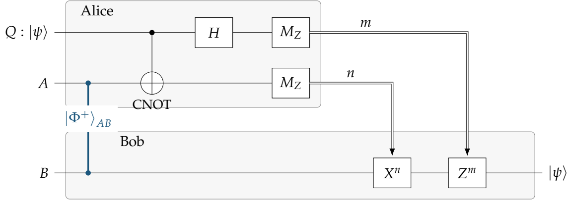
Figura 1: Circuito de teleportación con recurso |\Phi^+\rangle_{AB} . El tiempo avanza hacia la derecha; M_Z mide en la base computacional. El segmento azul izquierdo indica el par compartido, no una compuerta entre los laboratorios. Las líneas dobles llevan los bits clásicos que controlan las correcciones de Bob: primero X^n , después Z^m .
