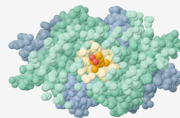
Tetrámero de TTR con tiroxina (naranja) en el canal · PDB 1ICT
