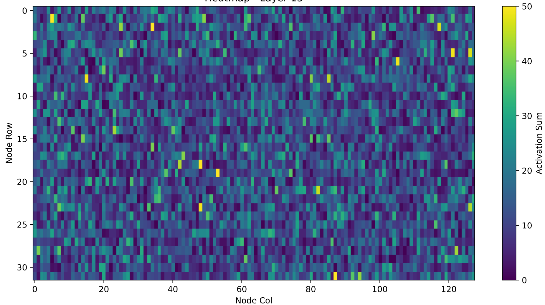
Heatmap - Layer 13
