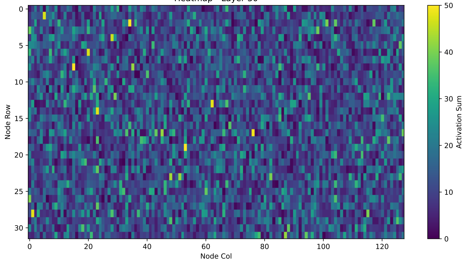
Heatmap - Layer 30
