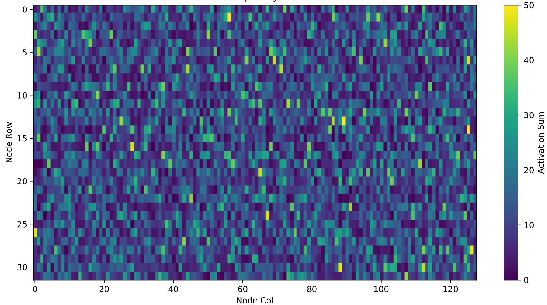
Heatmap - Layer 32
