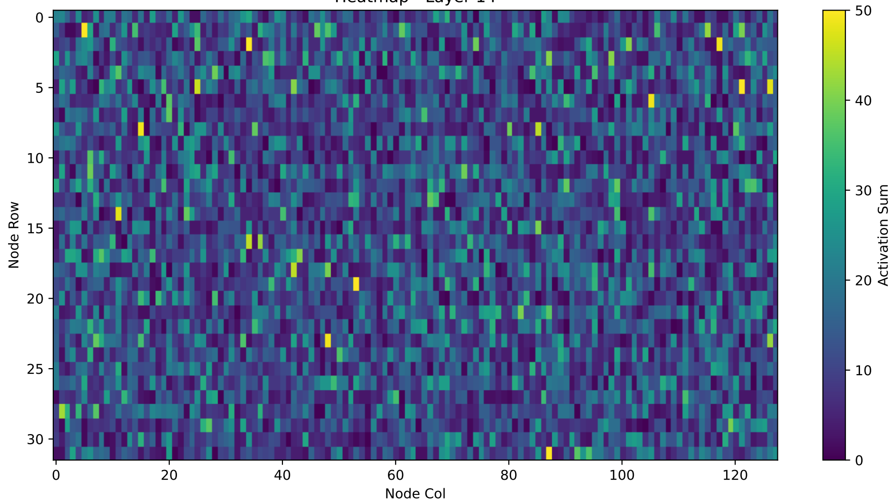
Heatmap - Layer 14
