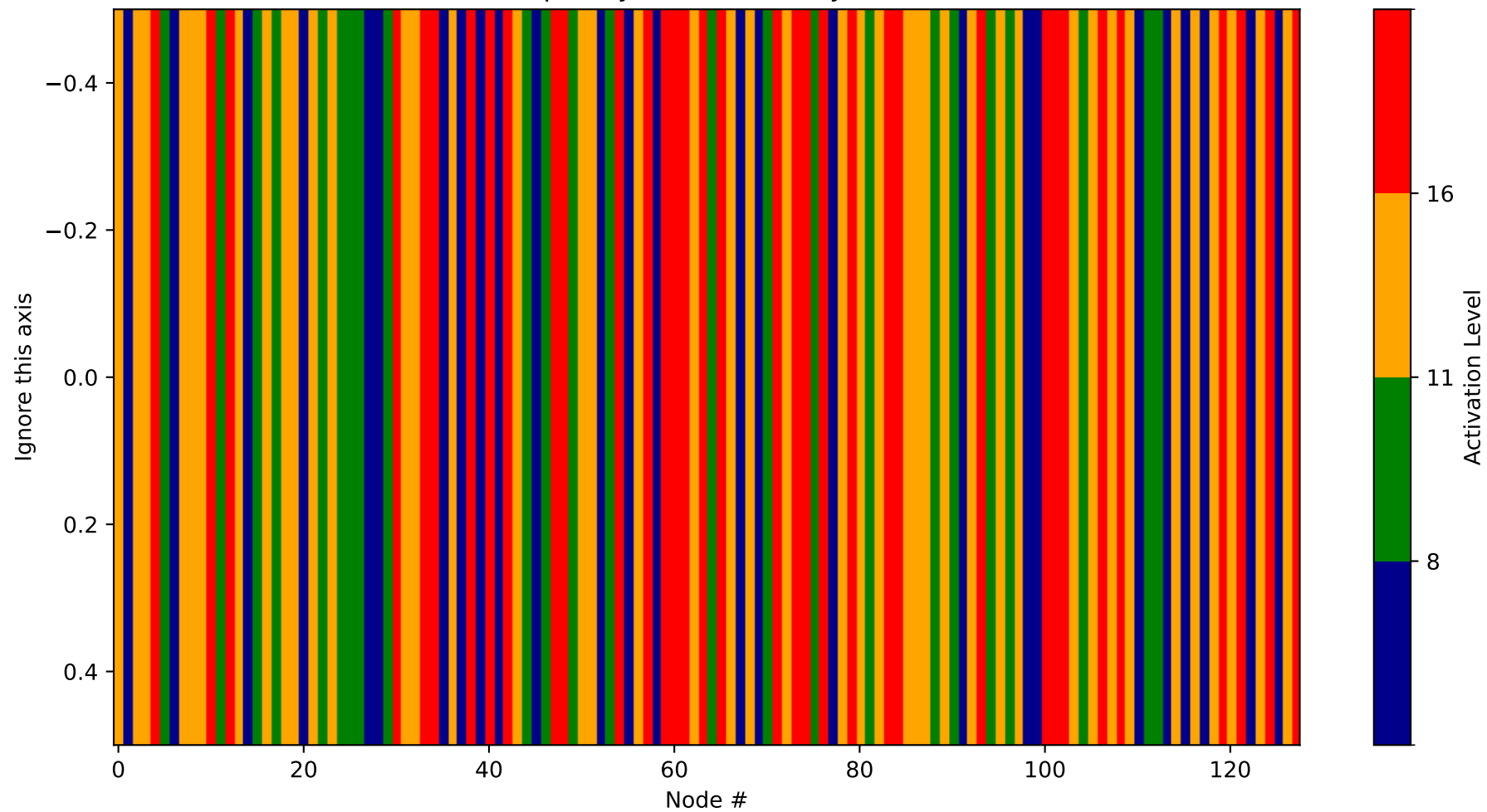
Heatmap - Layer 2 (Probability 256-384)
