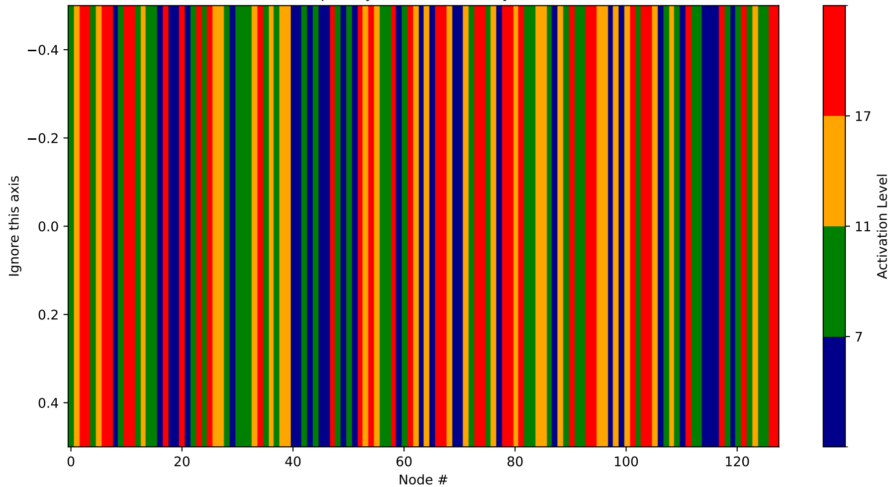
Heatmap - Layer 27 (Probability 256-384)
