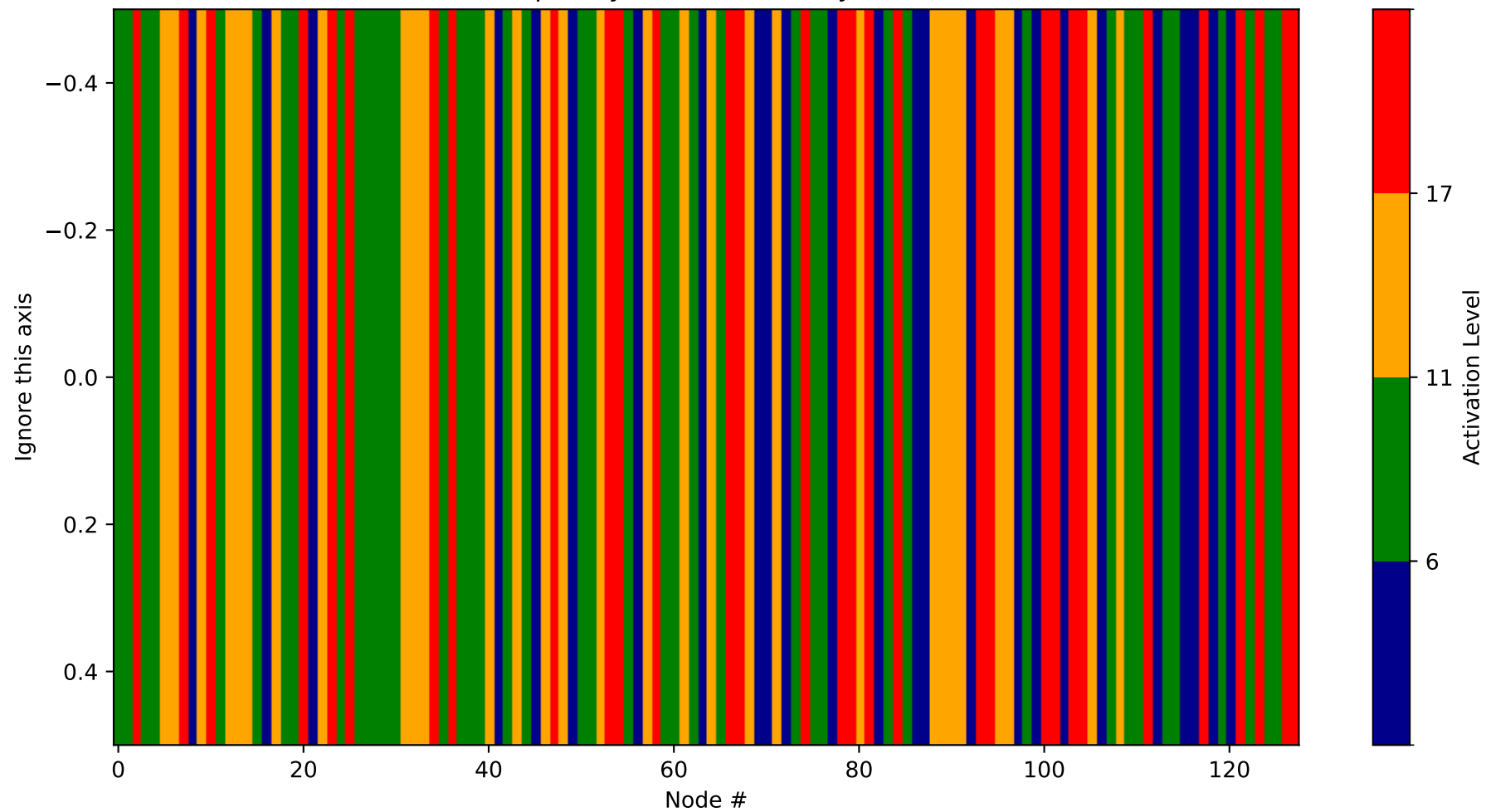
Heatmap - Layer 29 (Probability 256-384)
