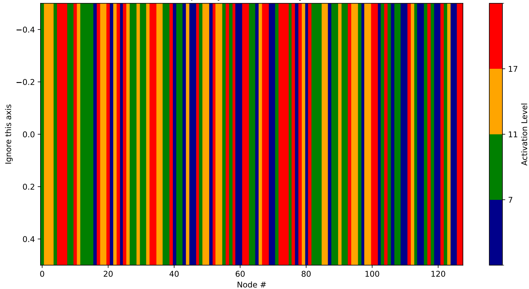
Heatmap - Layer 24 (Probability 256-384)
