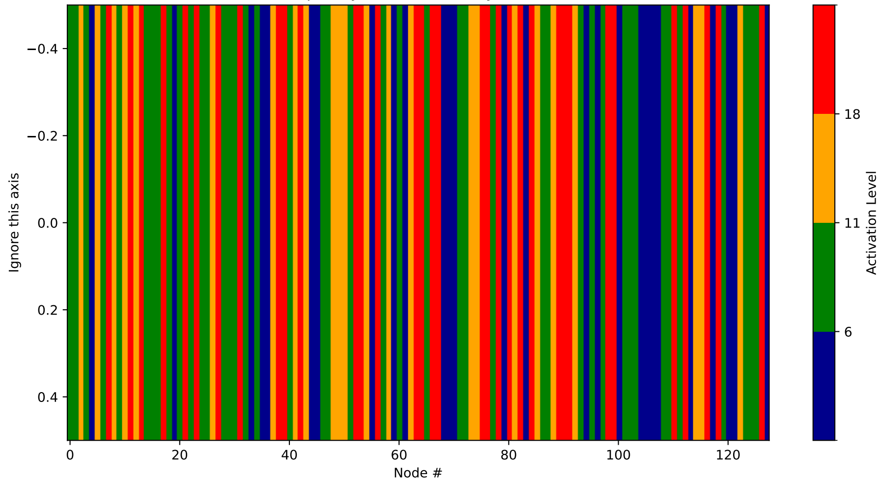
Heatmap - Layer 14 (Probability 1664-1792)
