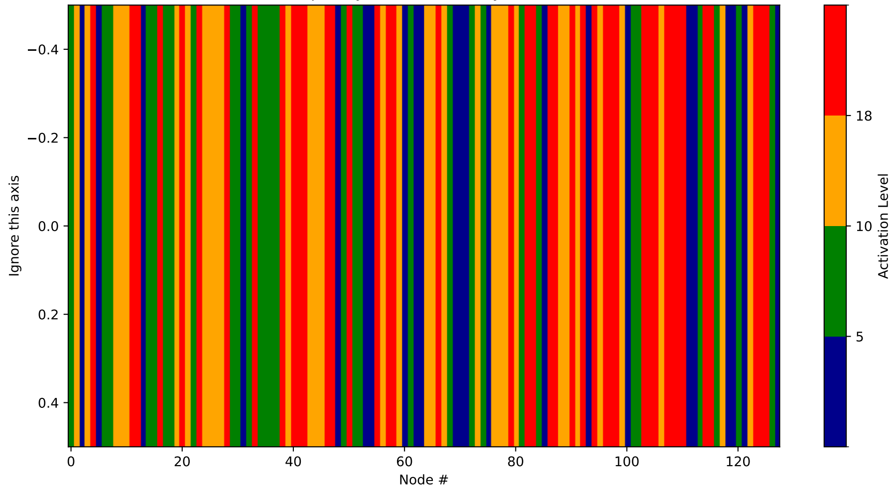
Heatmap - Layer 31 (Probability 3456-3584)
