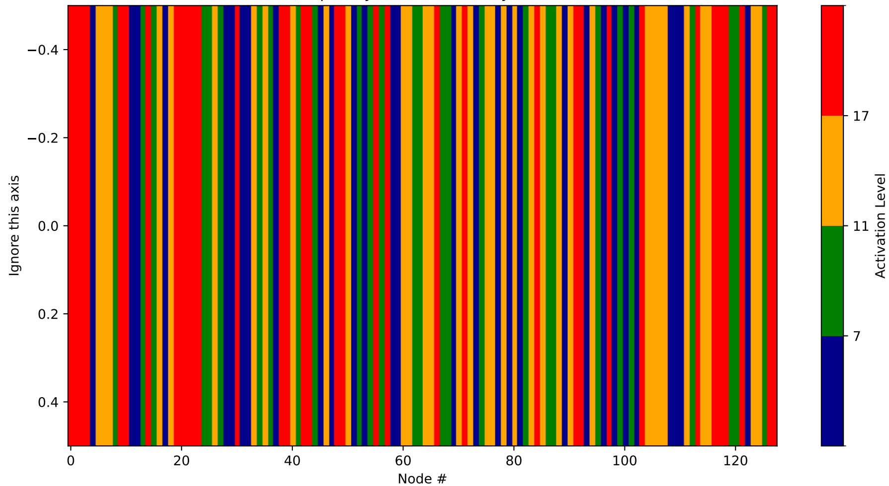
Heatmap - Layer 26 (Probability 640-768)
