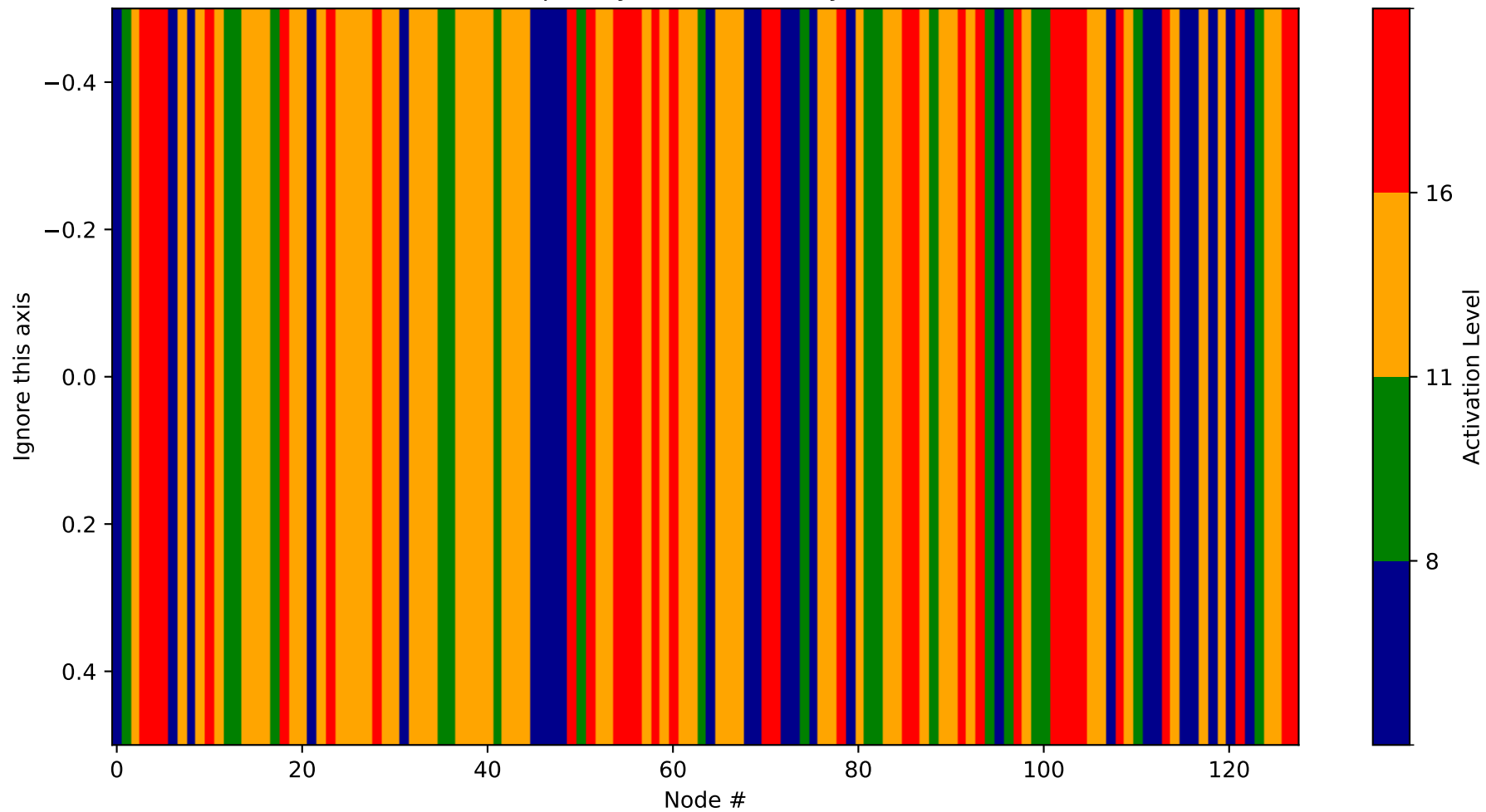
Heatmap - Layer 2 (Probability 640-768)
