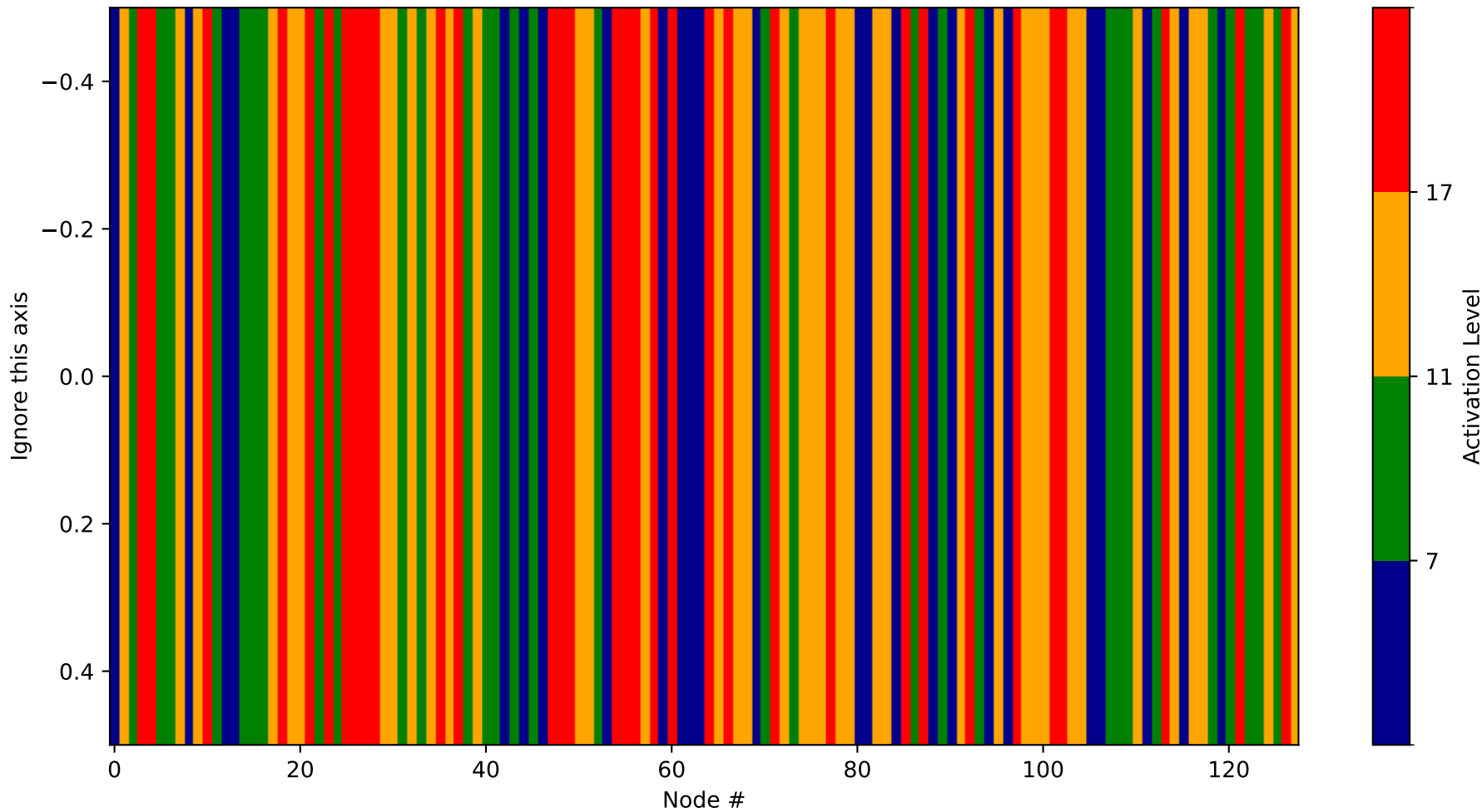
Heatmap - Layer 5 (Probability 640-768)
