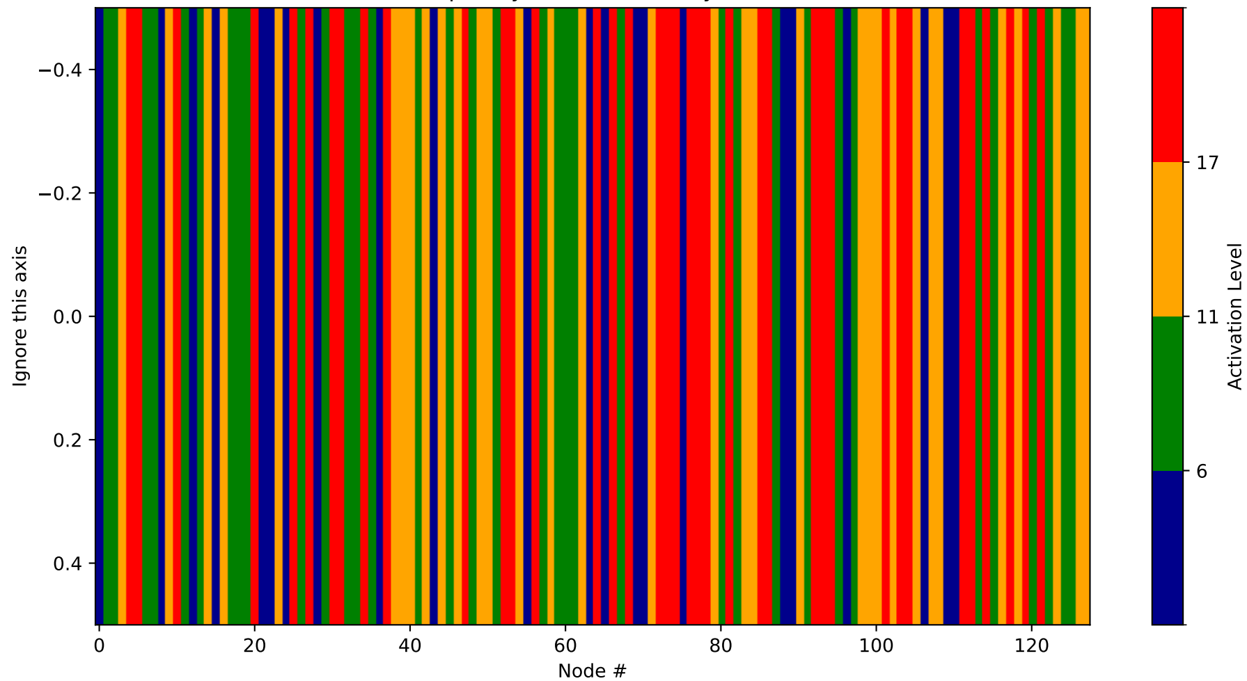
Heatmap - Layer 16 (Probability 256-384)
