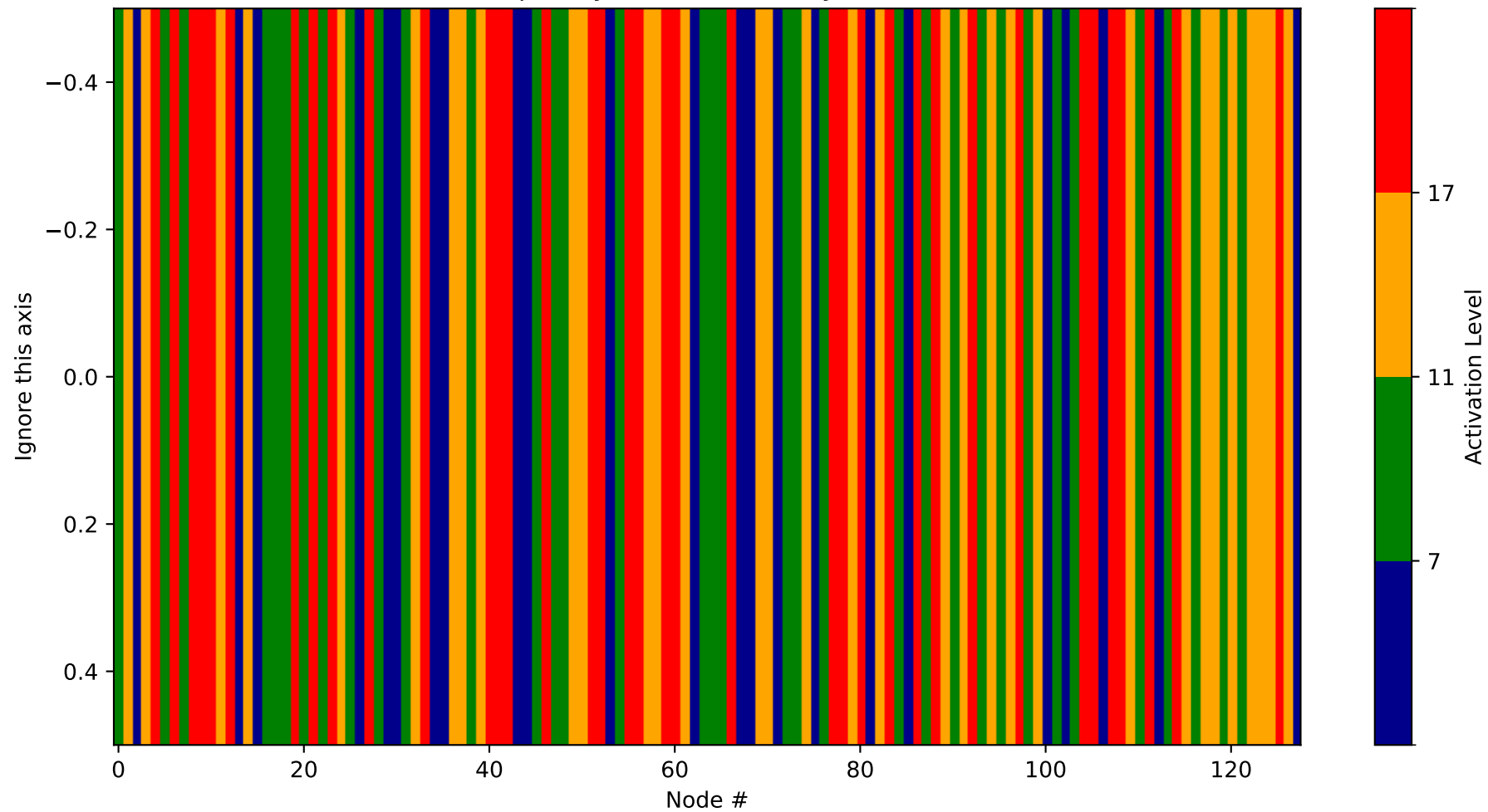
Heatmap - Layer 28 (Probability 3456-3584)
