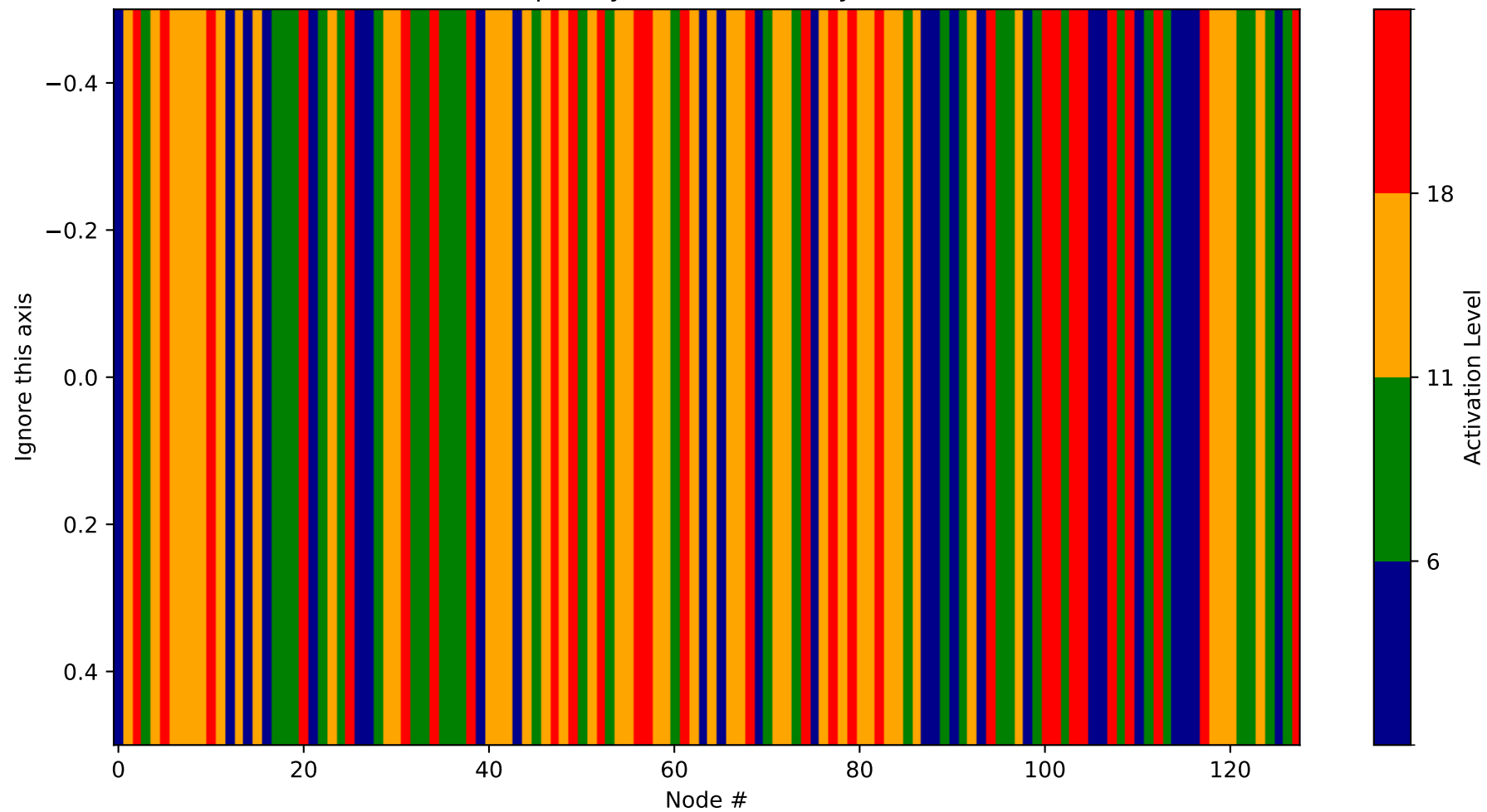
Heatmap - Layer 12 (Probability 256-384)
