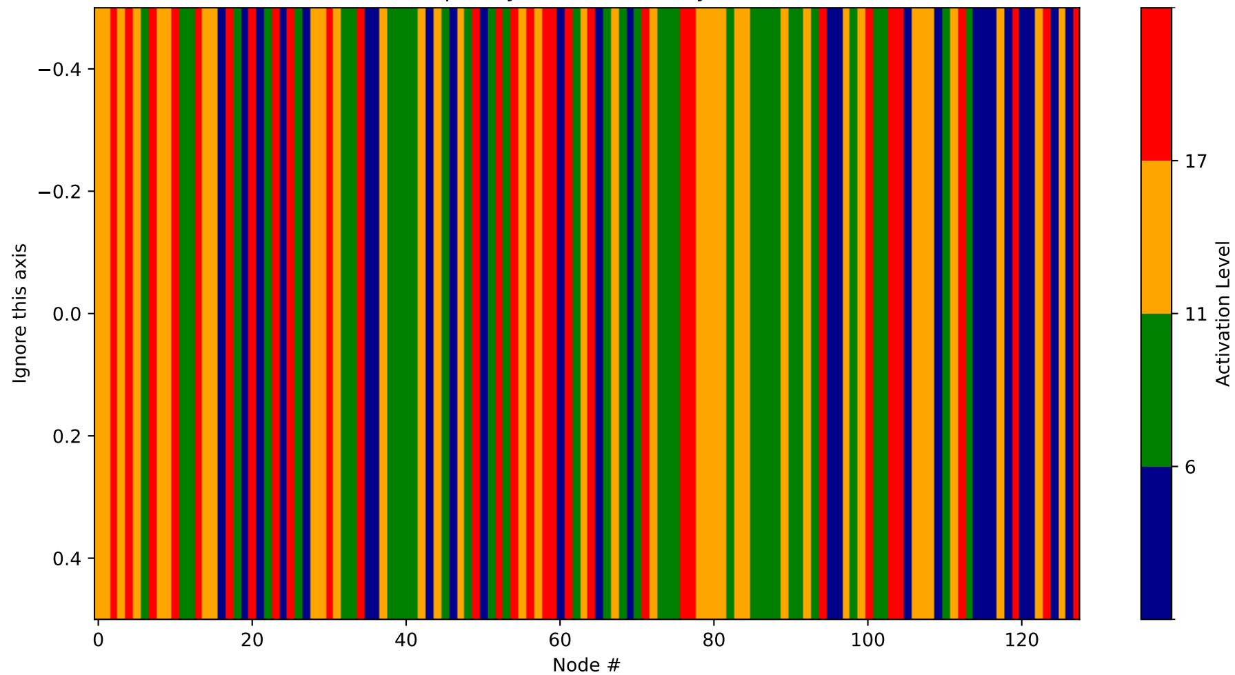
Heatmap - Layer 10 (Probability 256-384)
