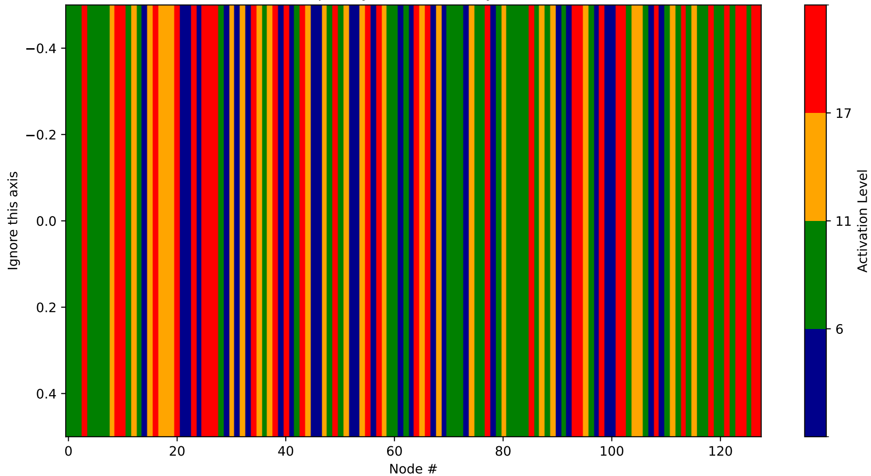
Heatmap - Layer 9 (Probability 640-768)
