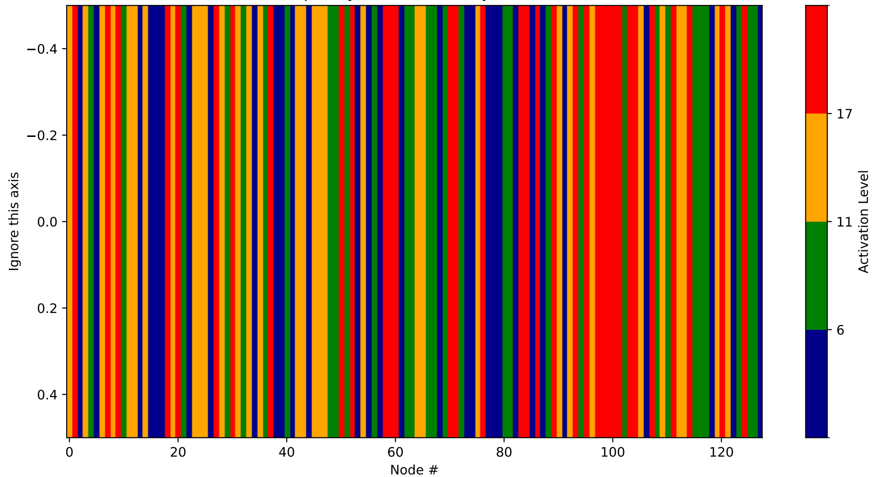
Heatmap - Layer 16 (Probability 3456-3584)
