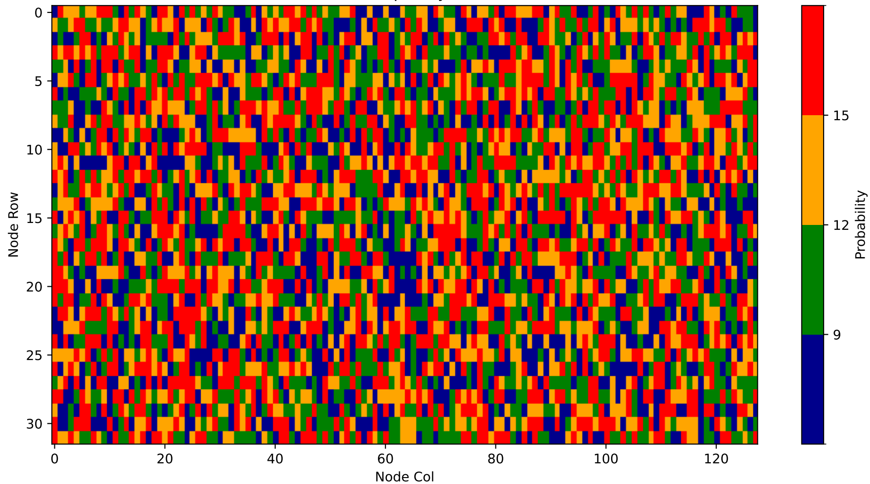
Heatmap - Layer 3
