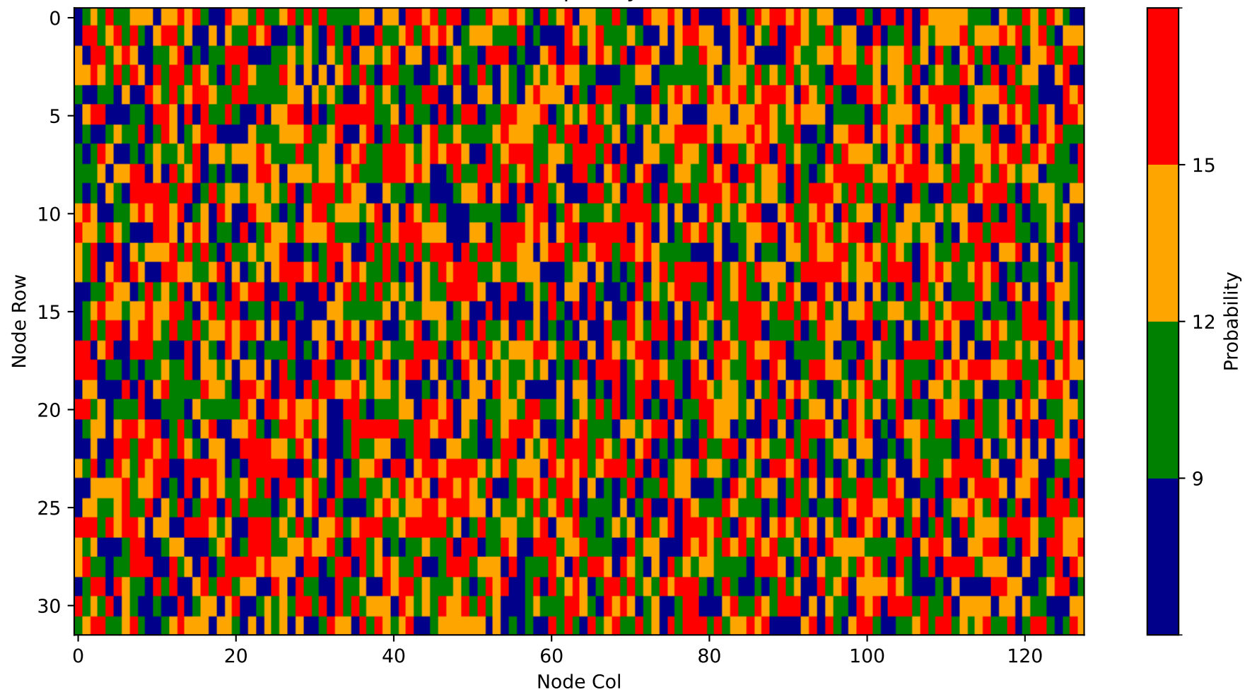
Heatmap - Layer 1
