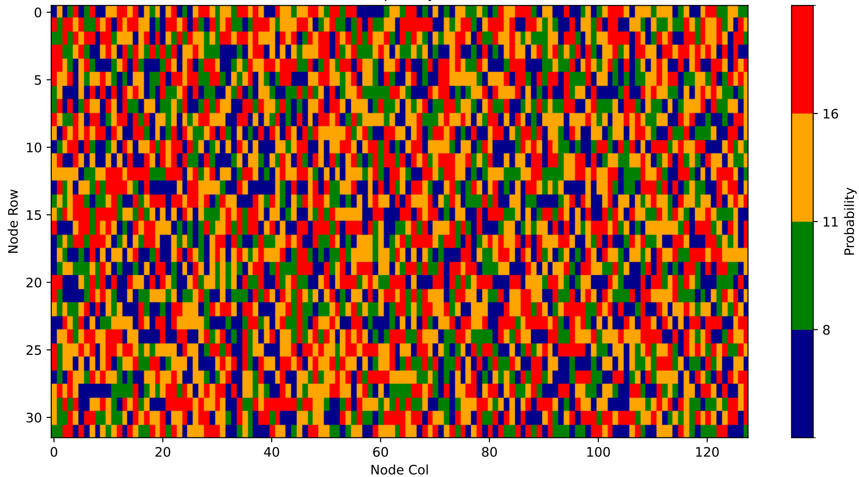
Heatmap - Layer 24
