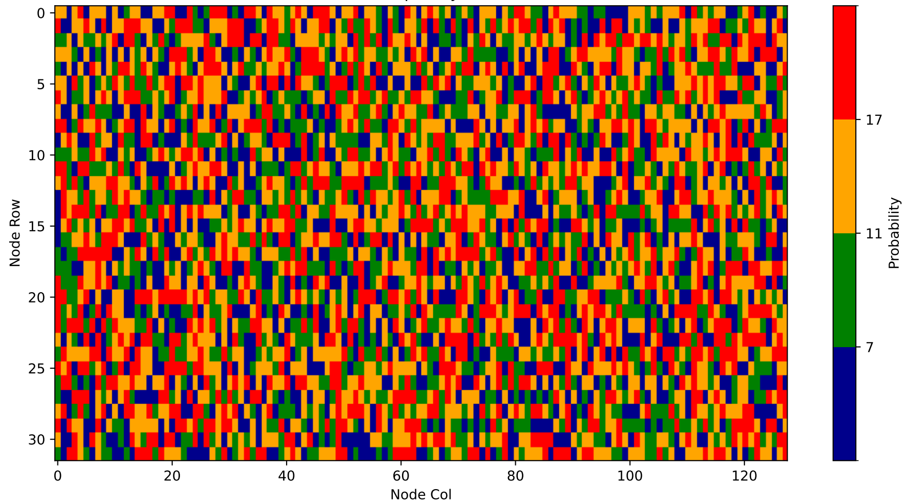
Heatmap - Layer 15
