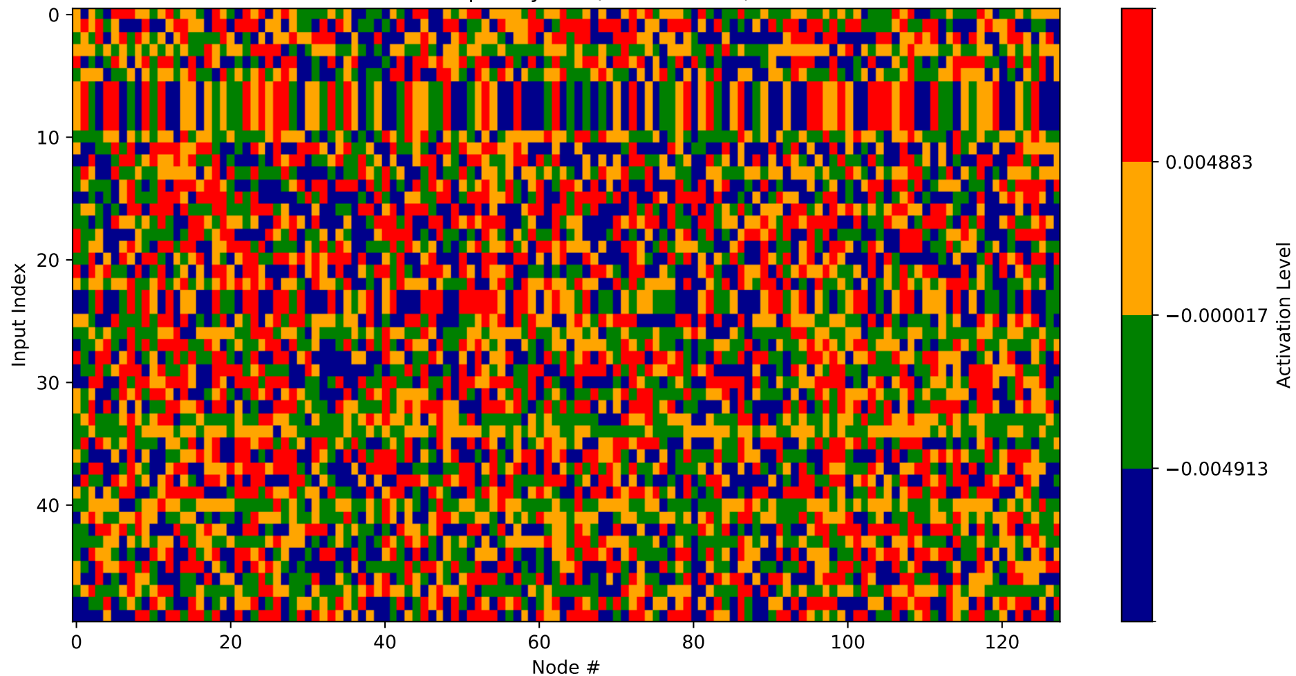
Heatmap - Layer 0 (Nodes 0-128)
