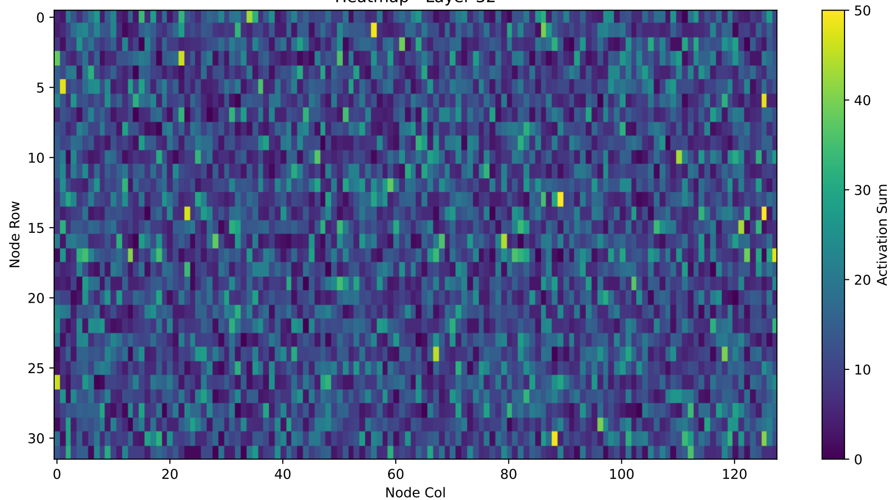
Heatmap - Layer 32
