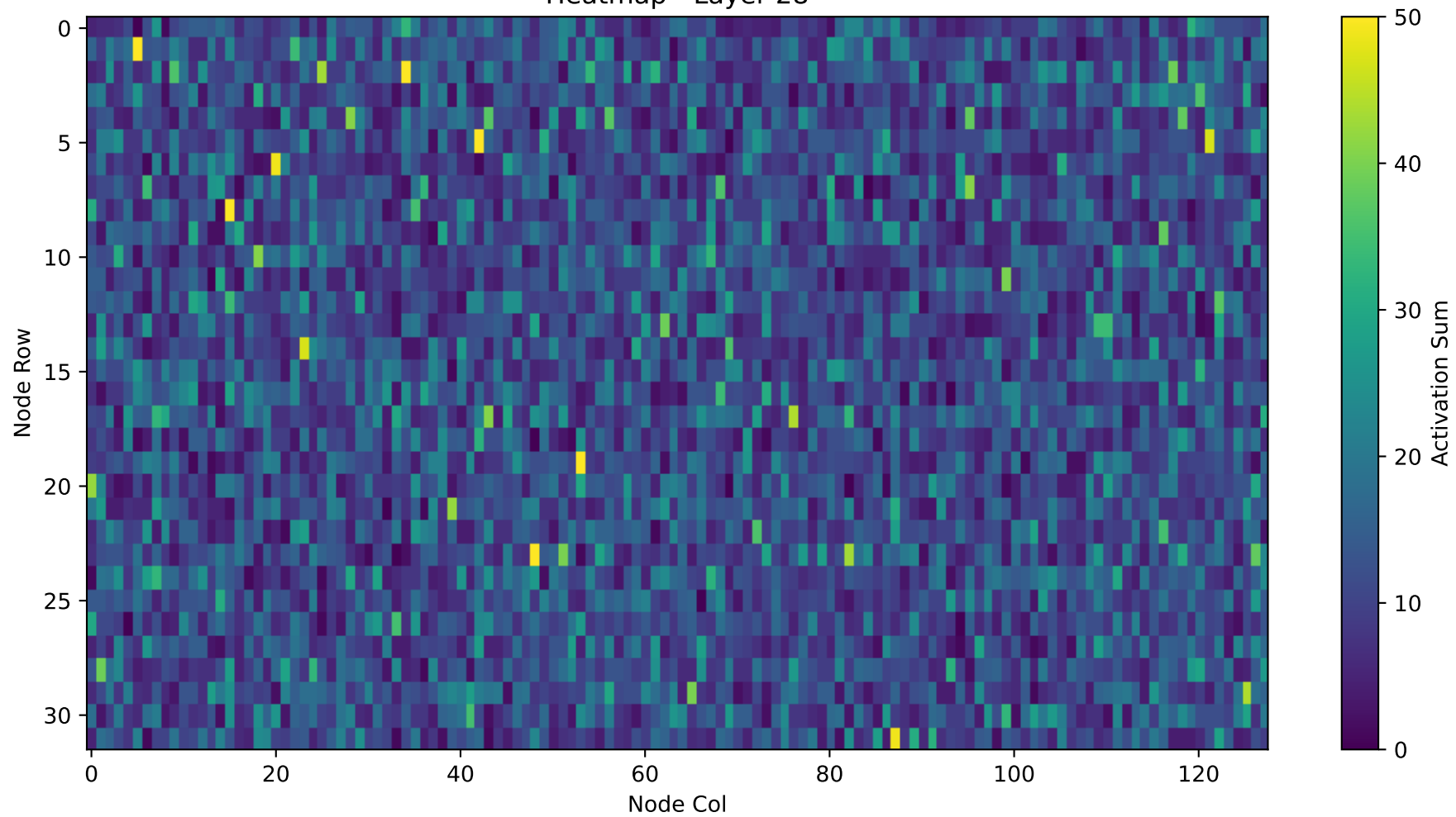
Heatmap - Layer 28
