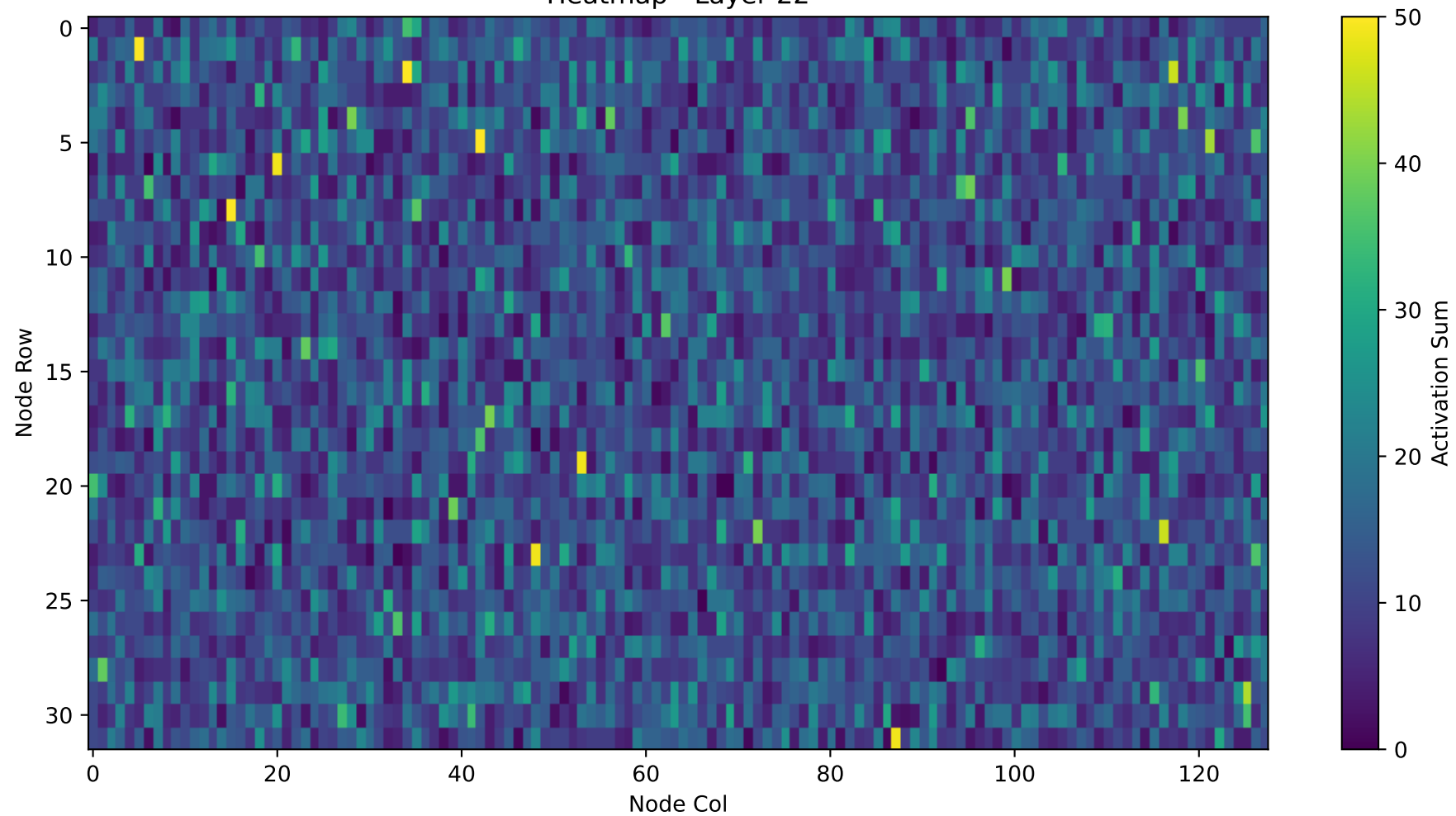
Heatmap - Layer 22
