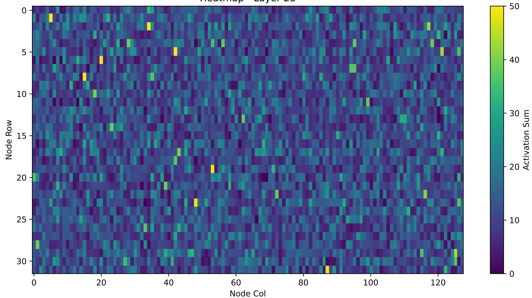
Heatmap - Layer 23
