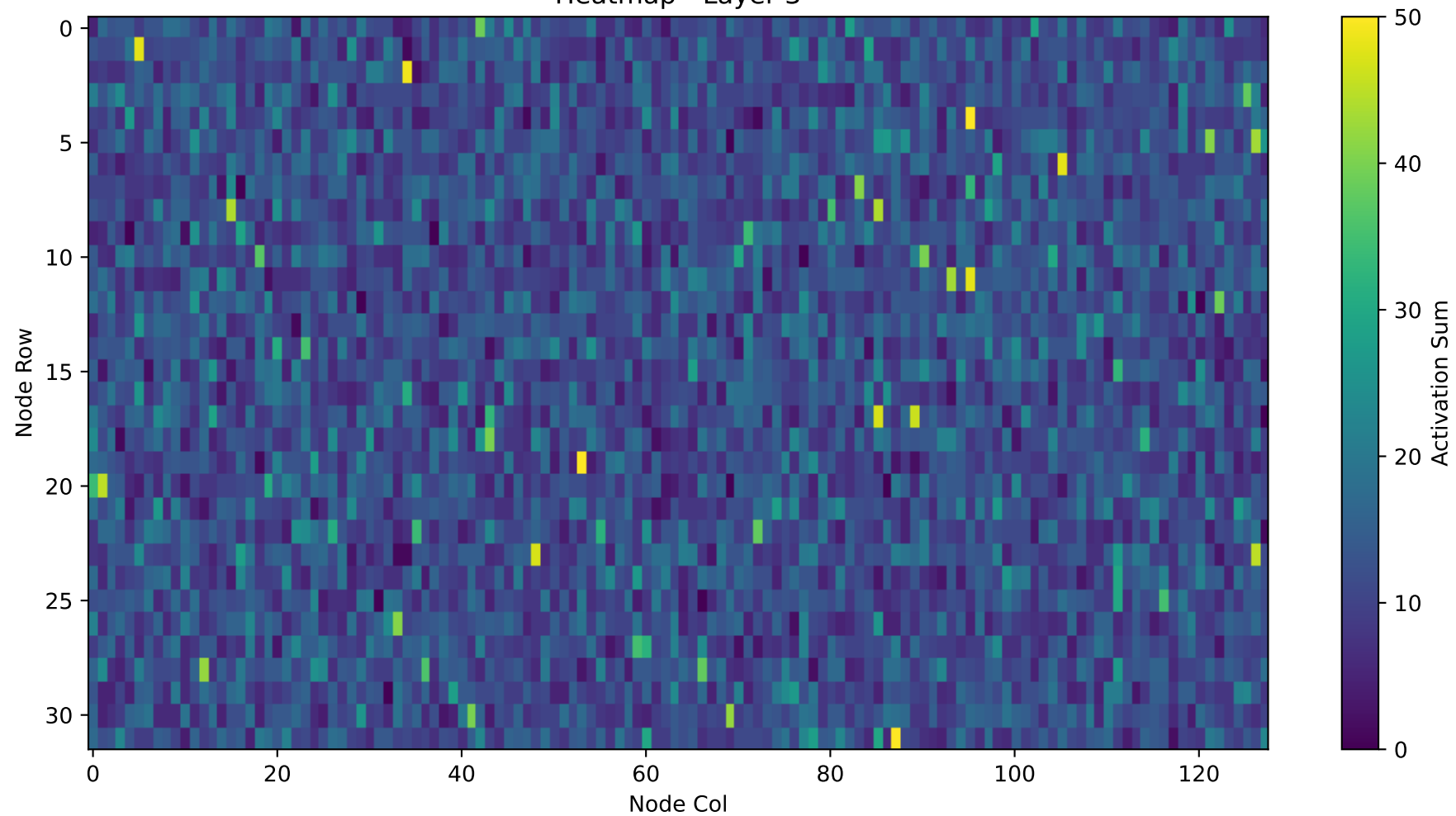
Heatmap - Layer 3
