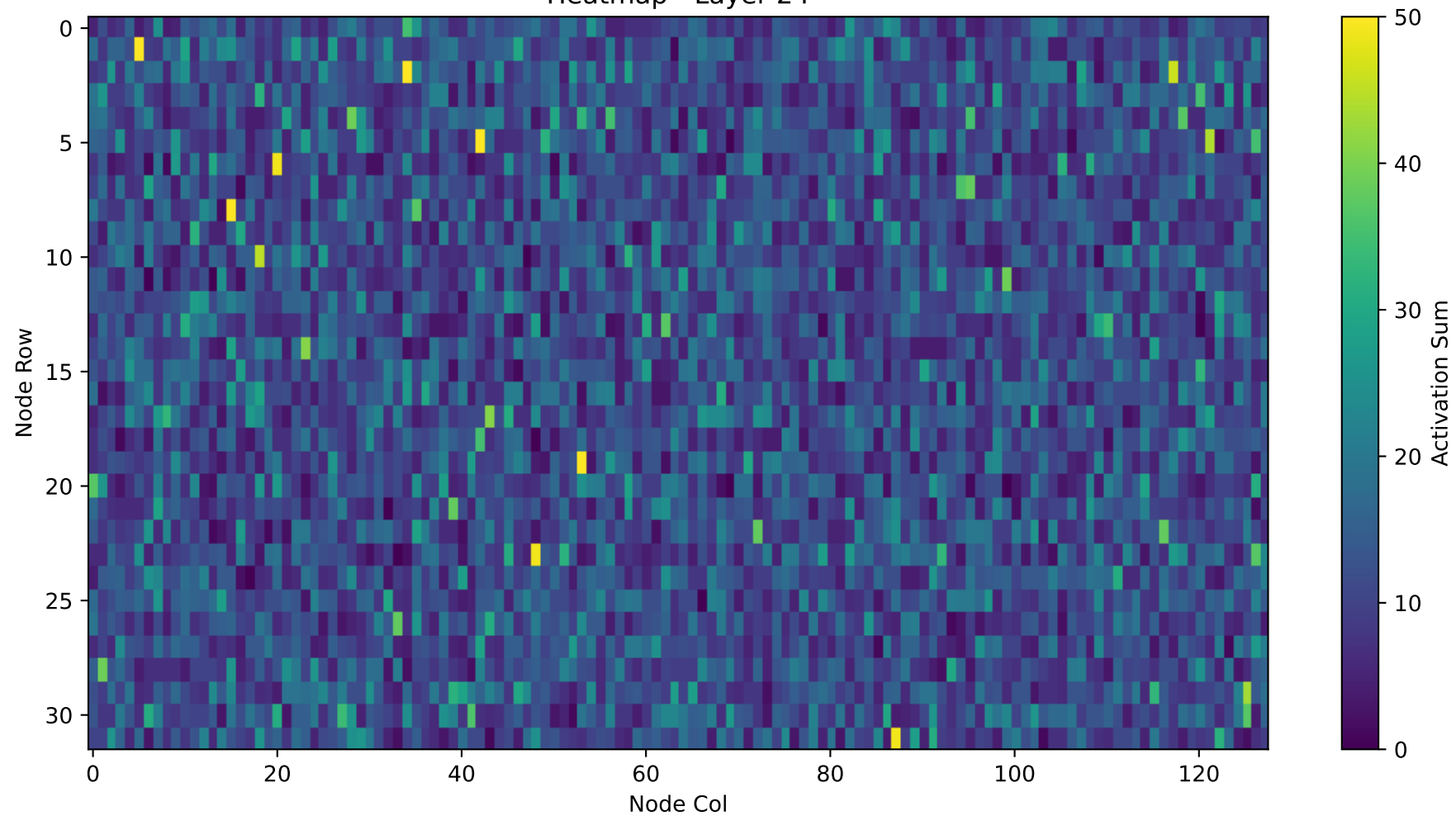
Heatmap - Layer 24
