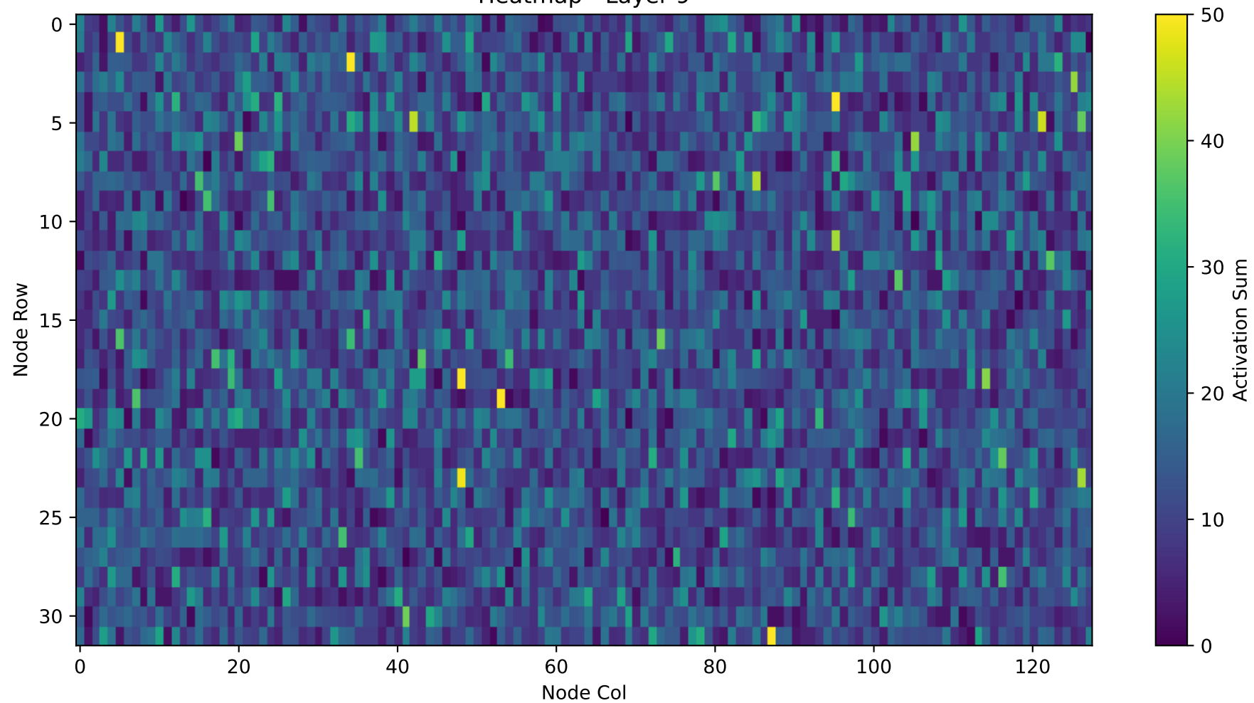
Heatmap - Layer 9
