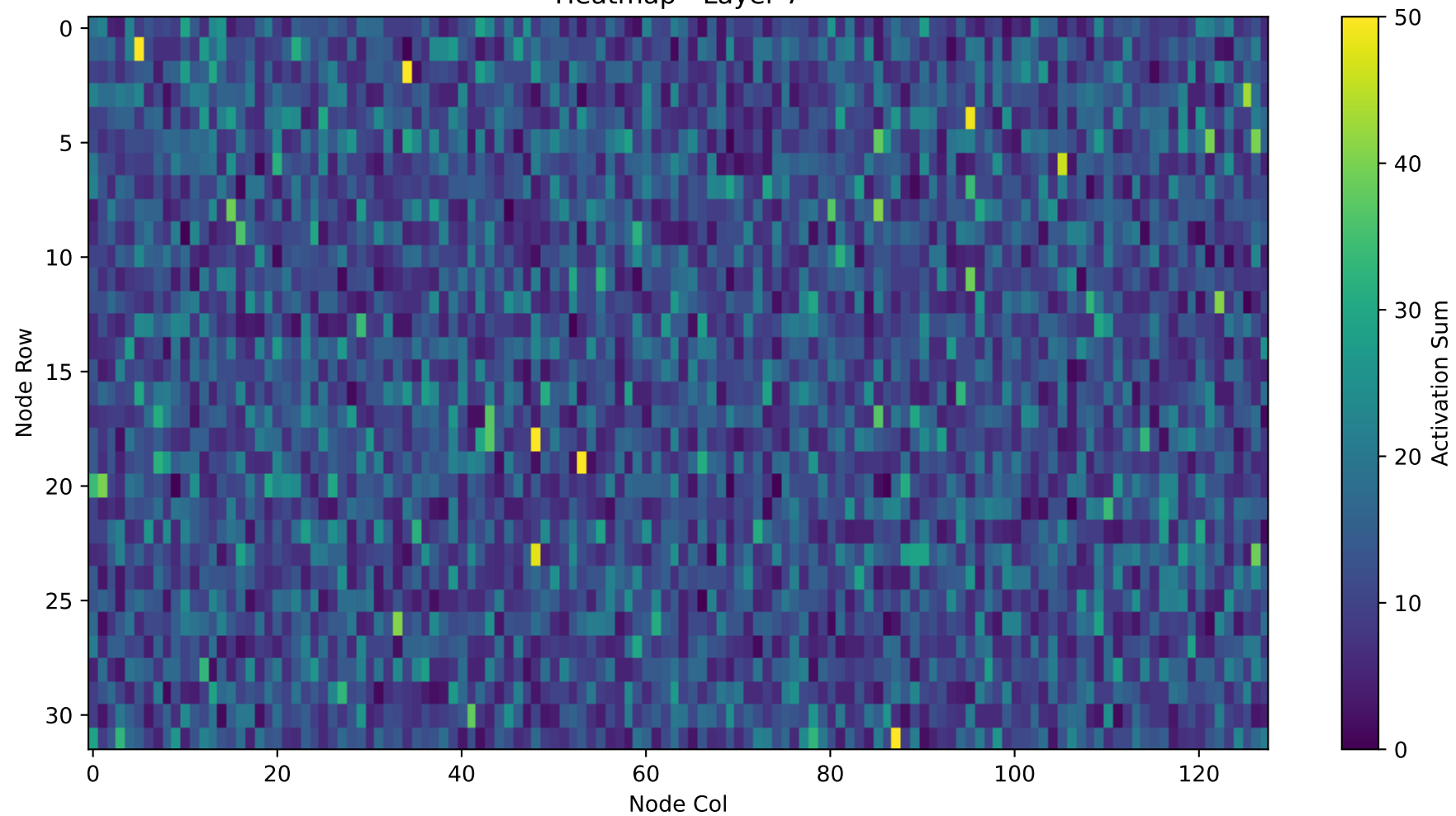
Heatmap - Layer 7
