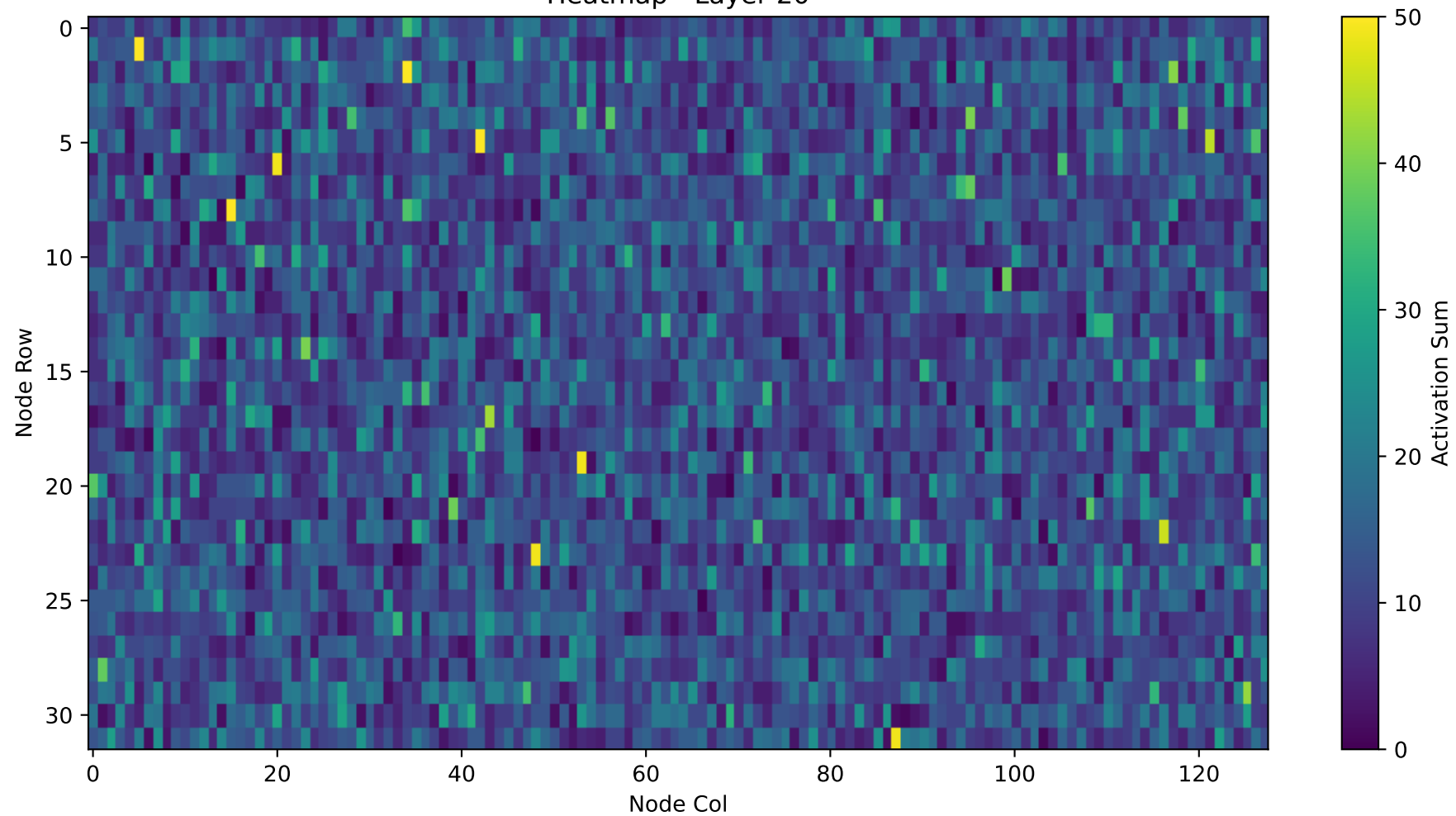
Heatmap - Layer 20
