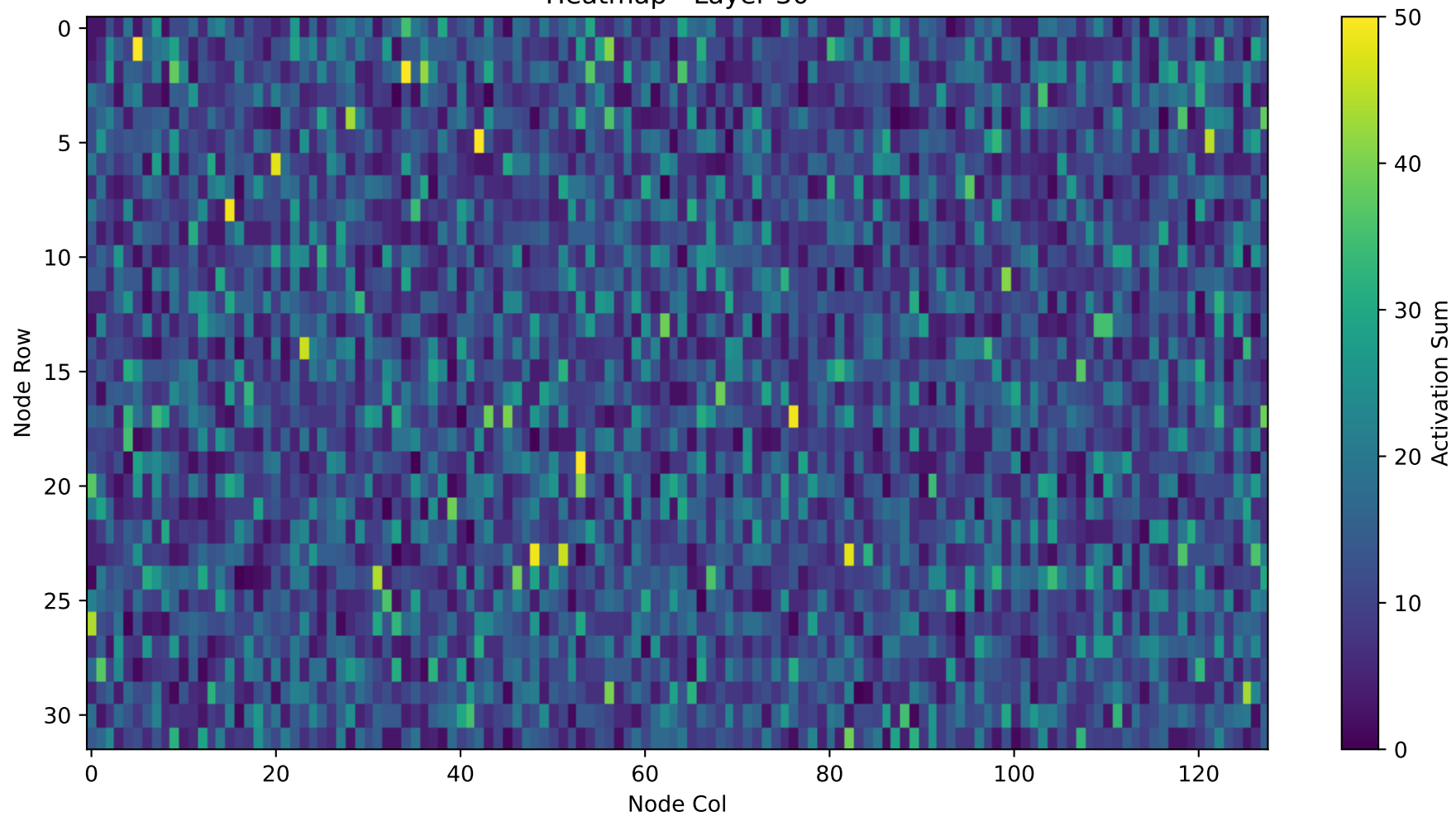
Heatmap - Layer 30
