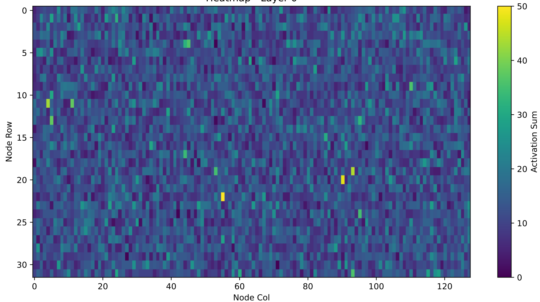
Heatmap - Layer 0
