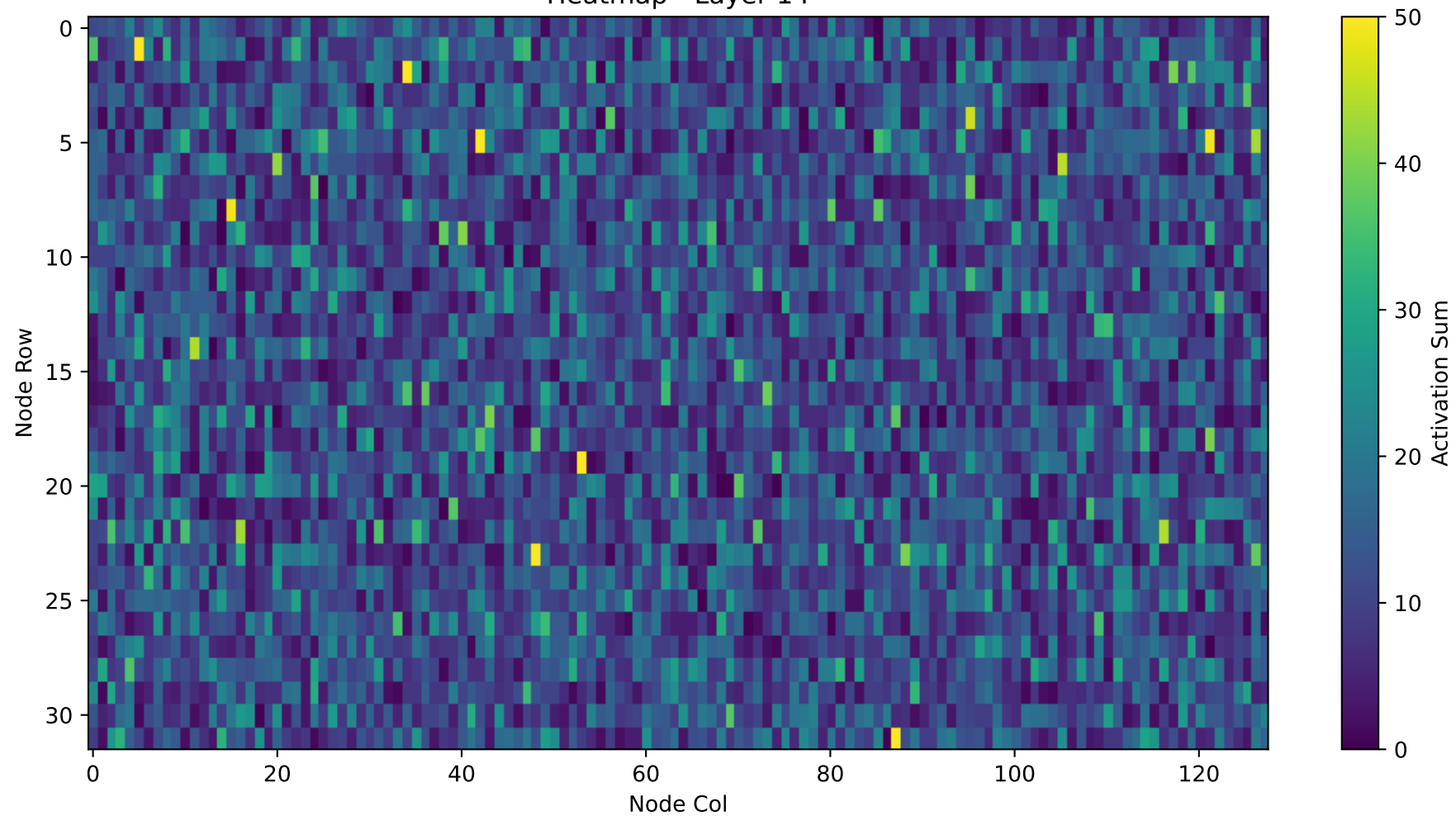
Heatmap - Layer 14
