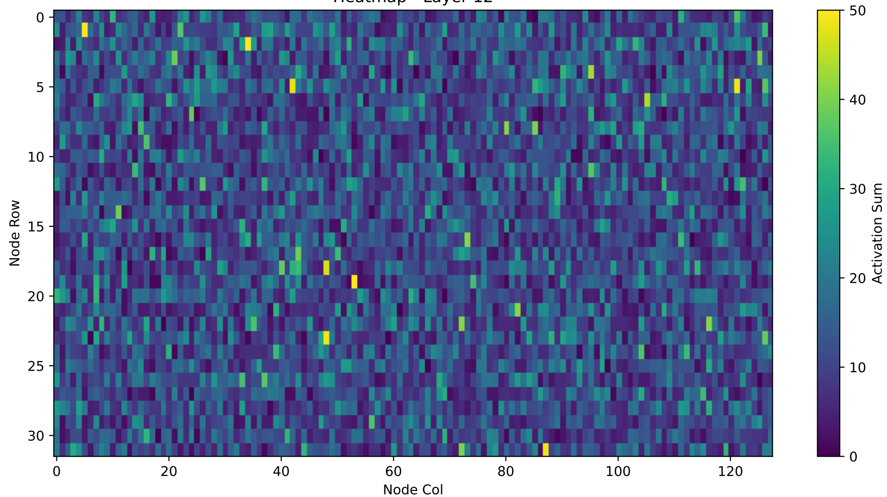
Heatmap - Layer 12
