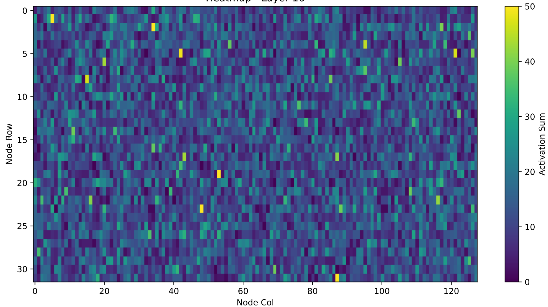
Heatmap - Layer 16
