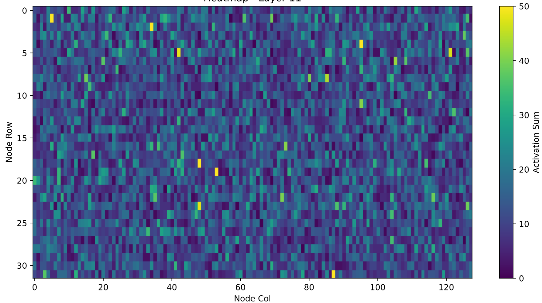
Heatmap - Layer 11
