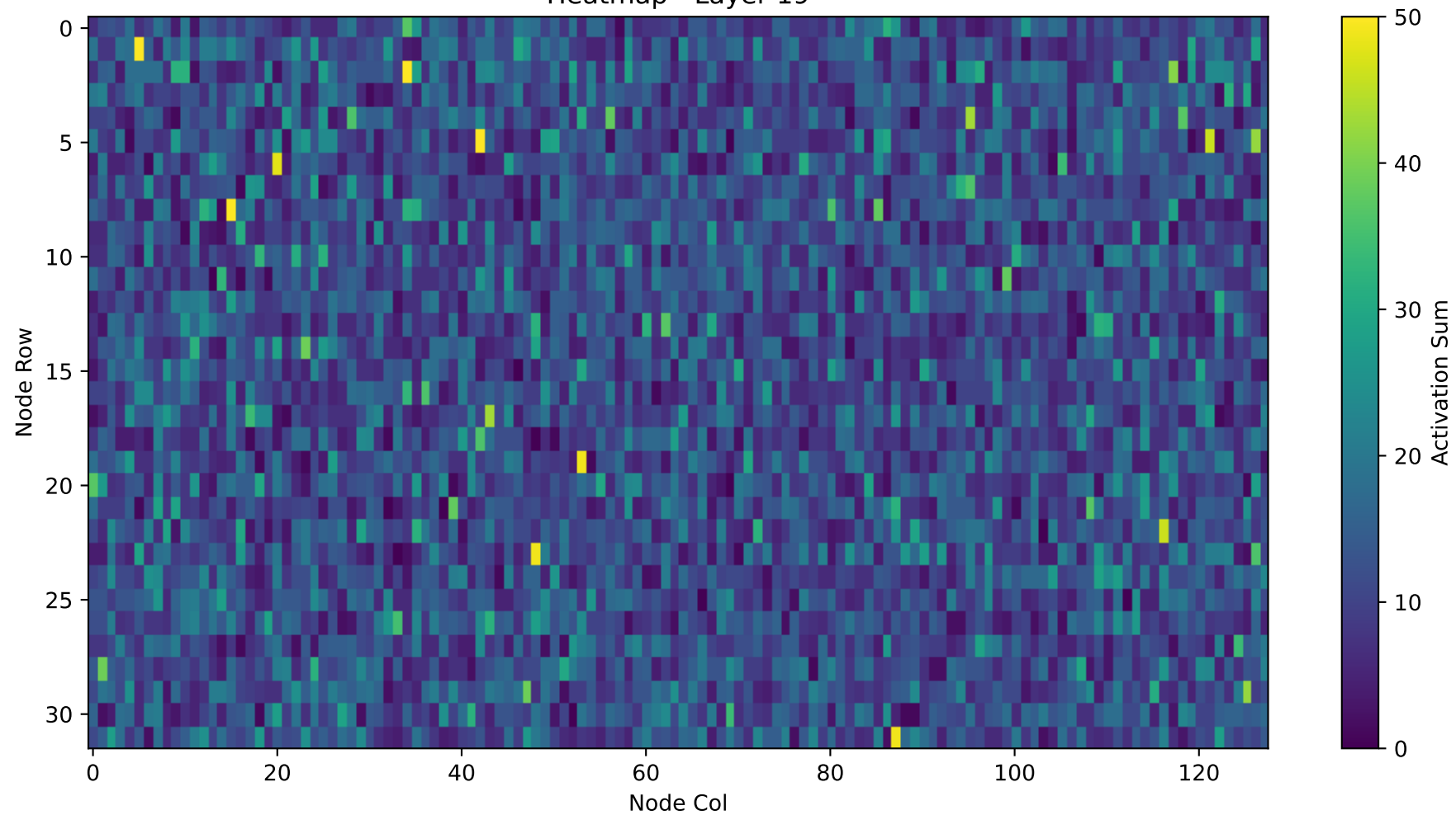
Heatmap - Layer 19
