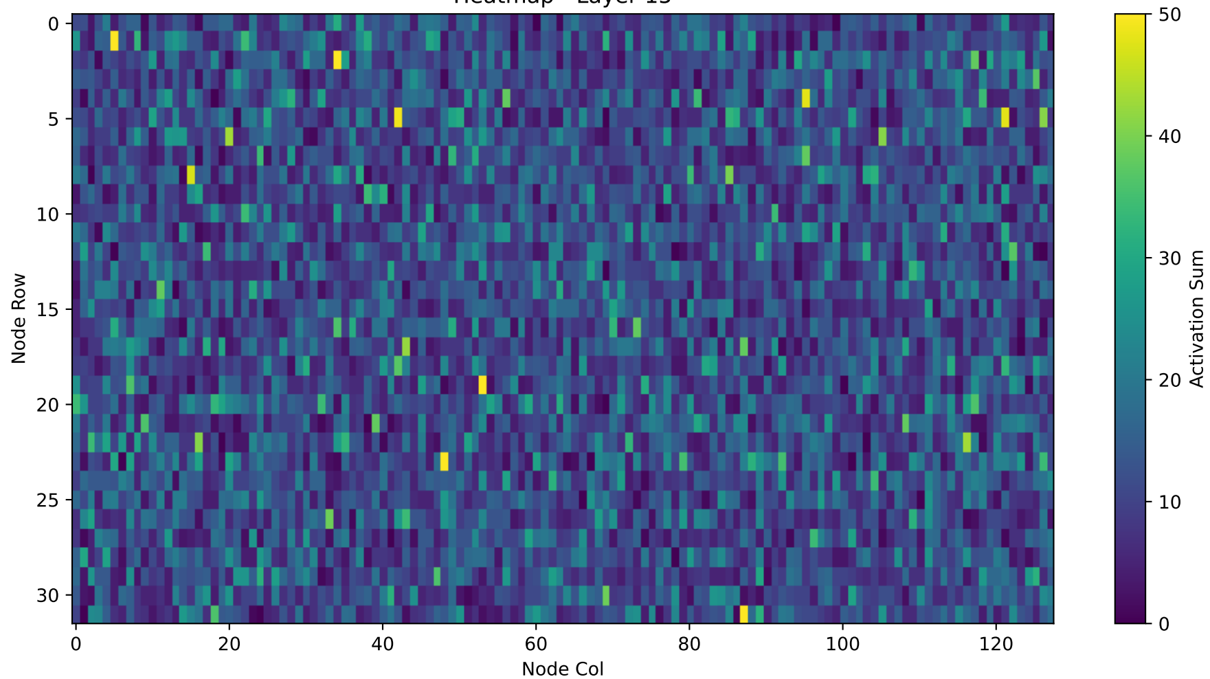
Heatmap - Layer 15
