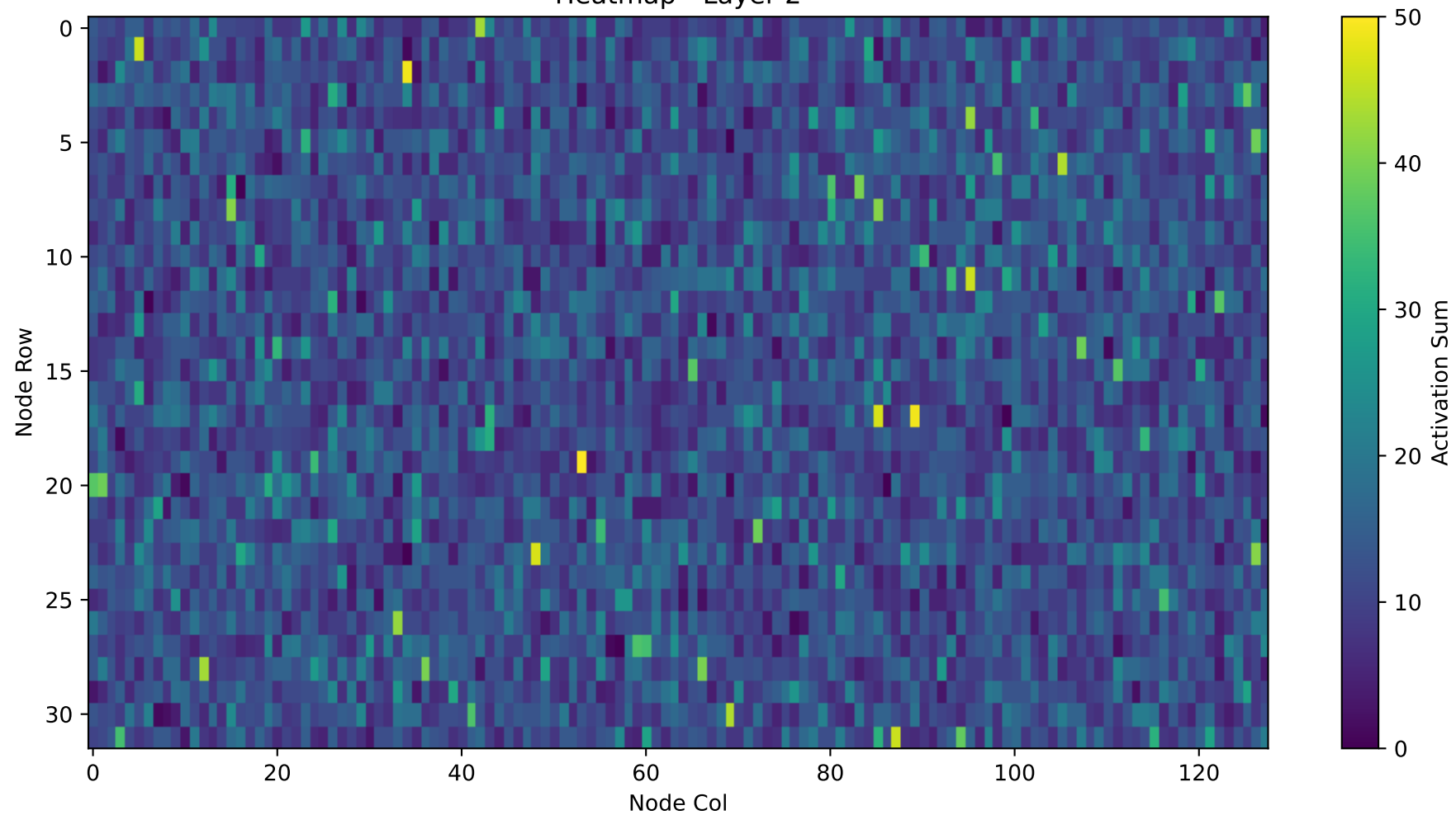
Heatmap - Layer 2
