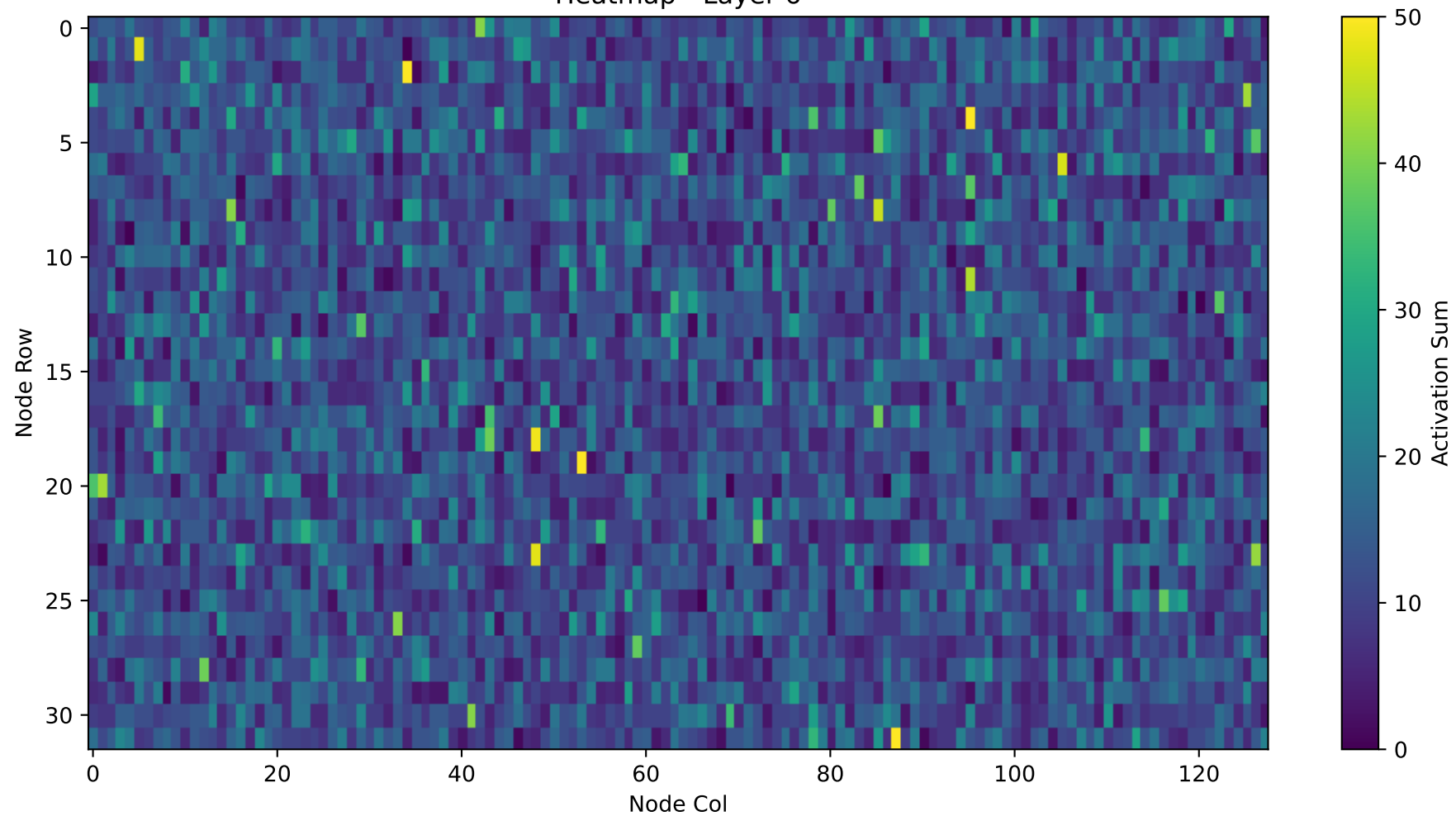
Heatmap - Layer 6
