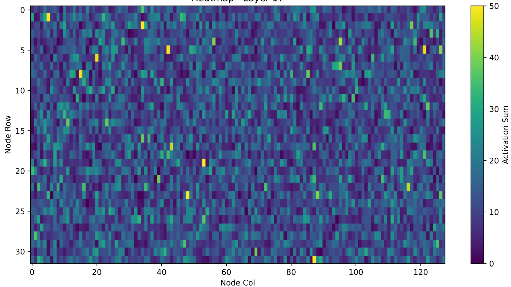
Heatmap - Layer 17
