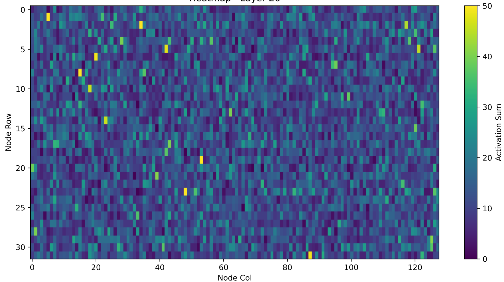
Heatmap - Layer 26
