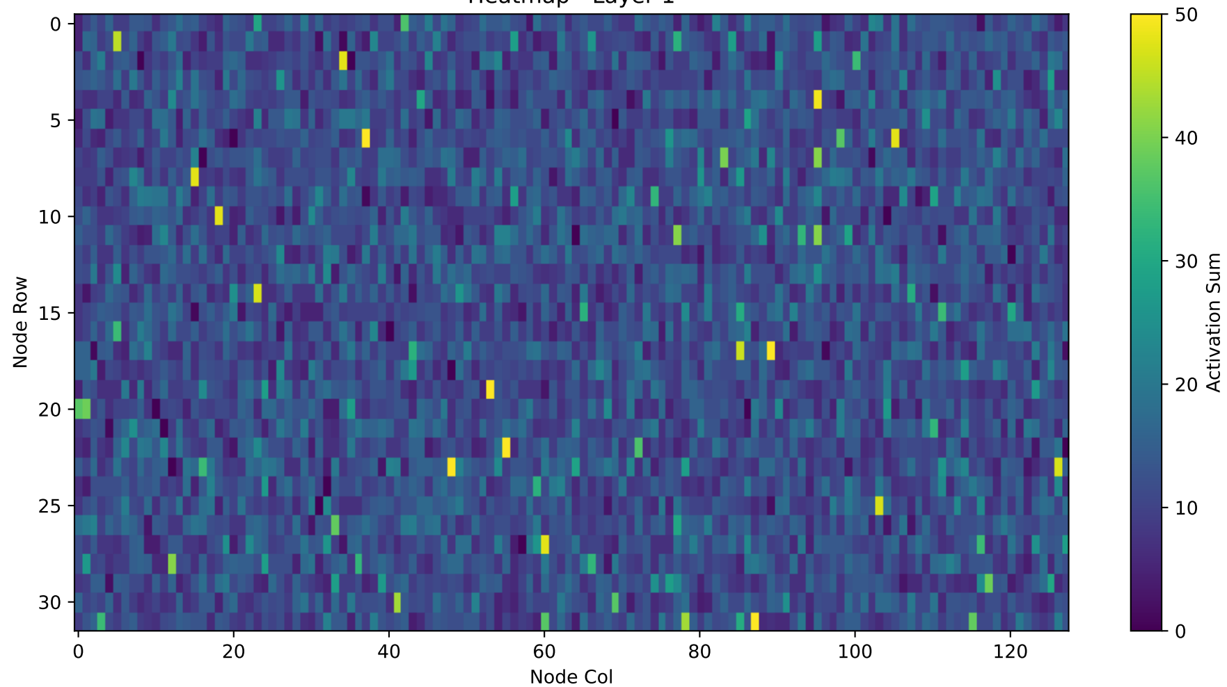
Heatmap - Layer 1
