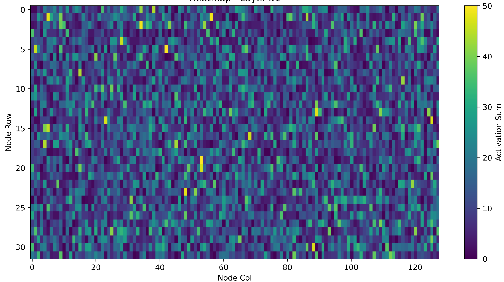
Heatmap - Layer 31
