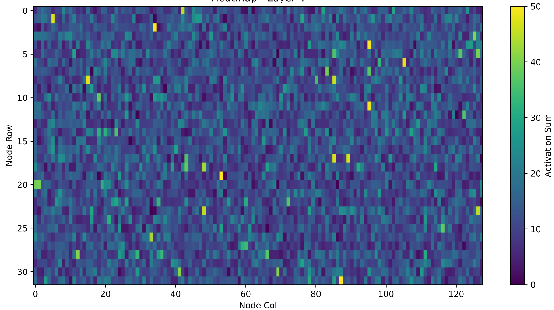
Heatmap - Layer 4
