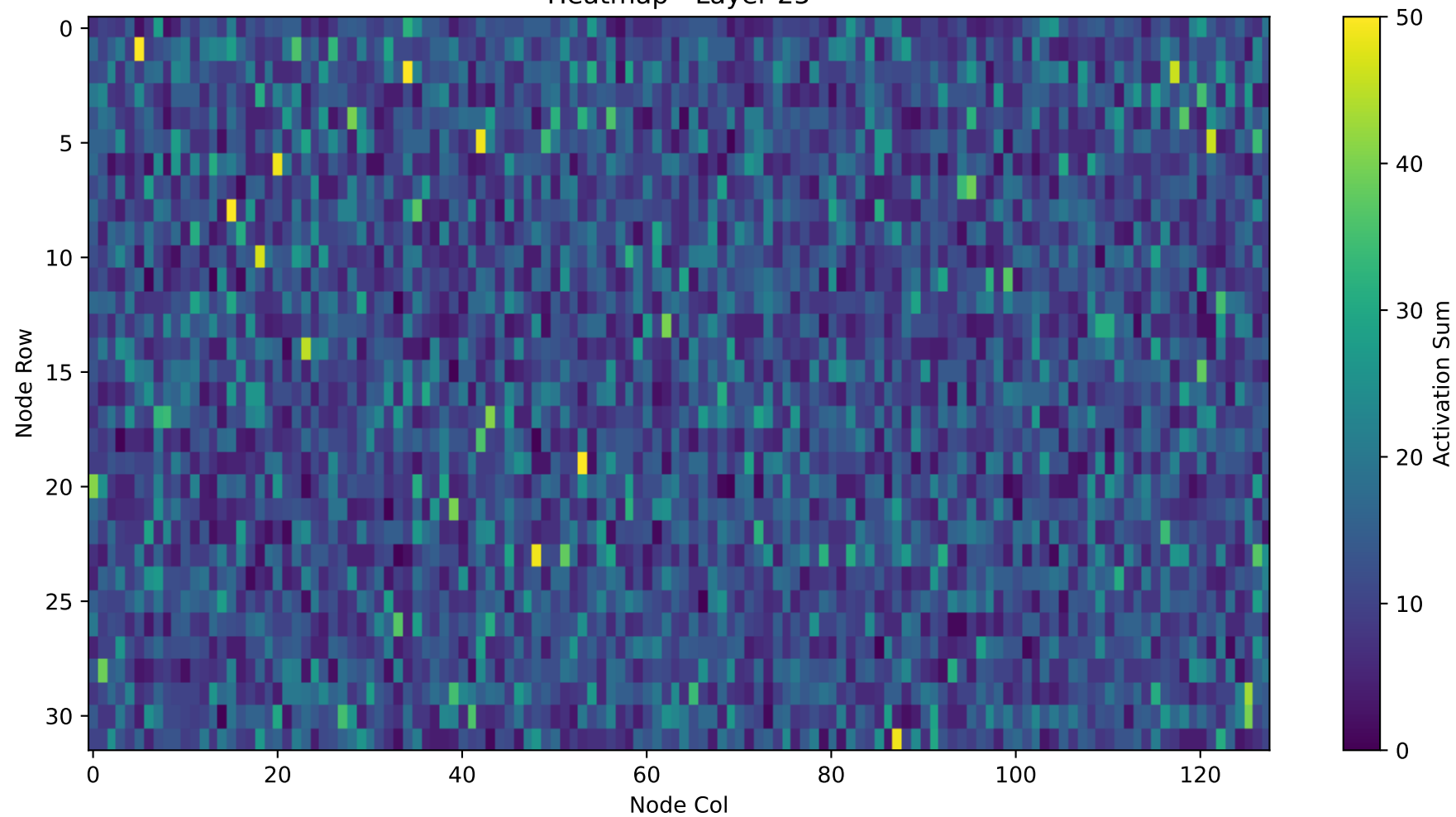
Heatmap - Layer 25
