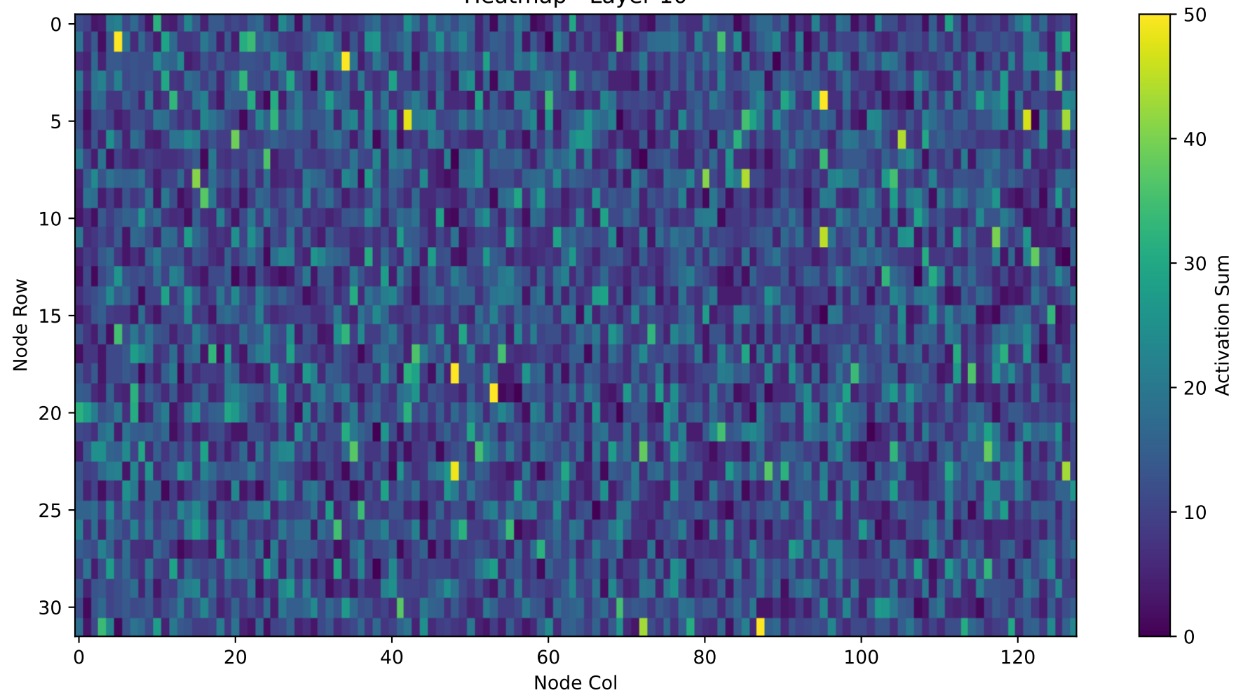
Heatmap - Layer 10
