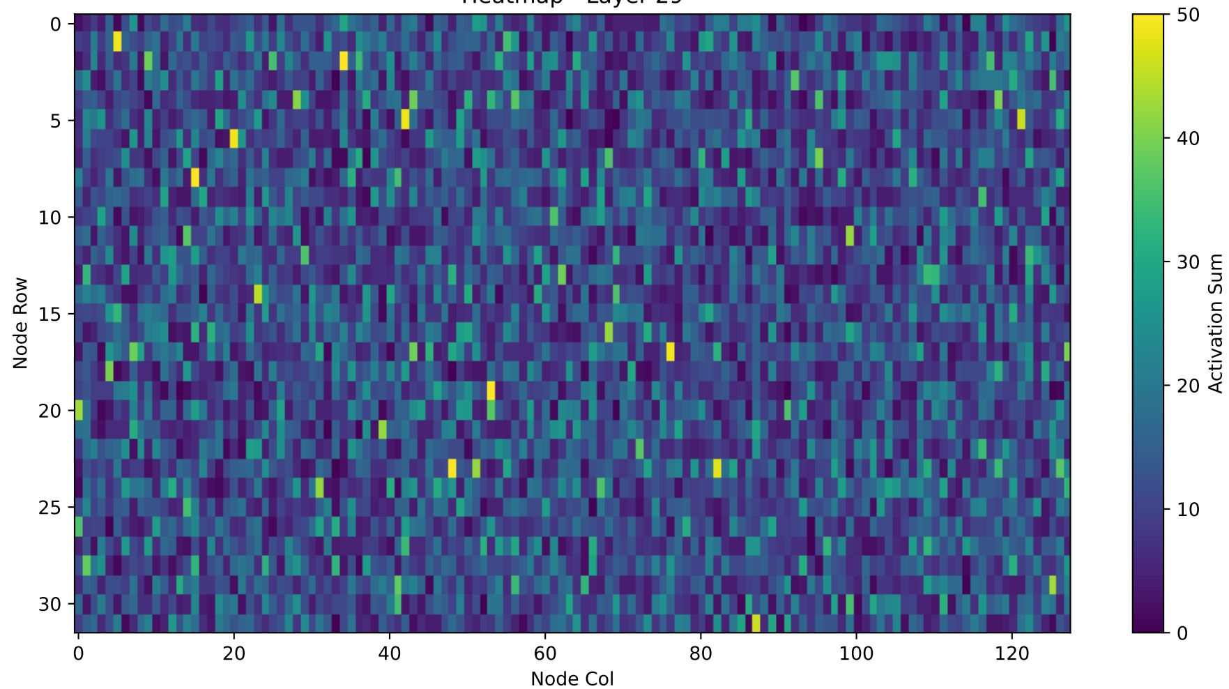
Heatmap - Layer 29
