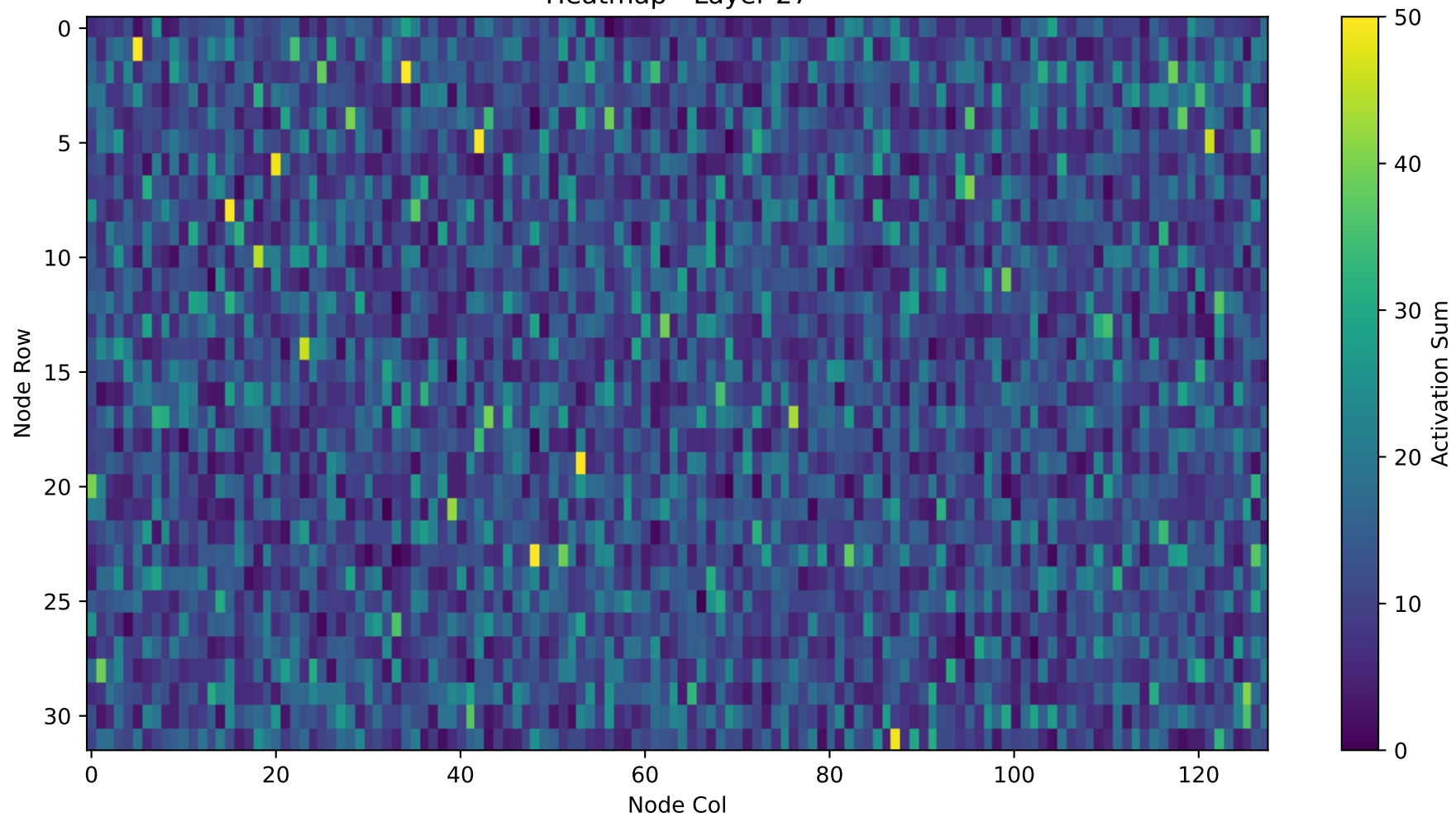
Heatmap - Layer 27
