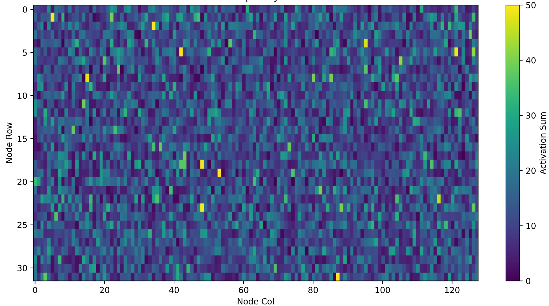
Heatmap - Layer 13
