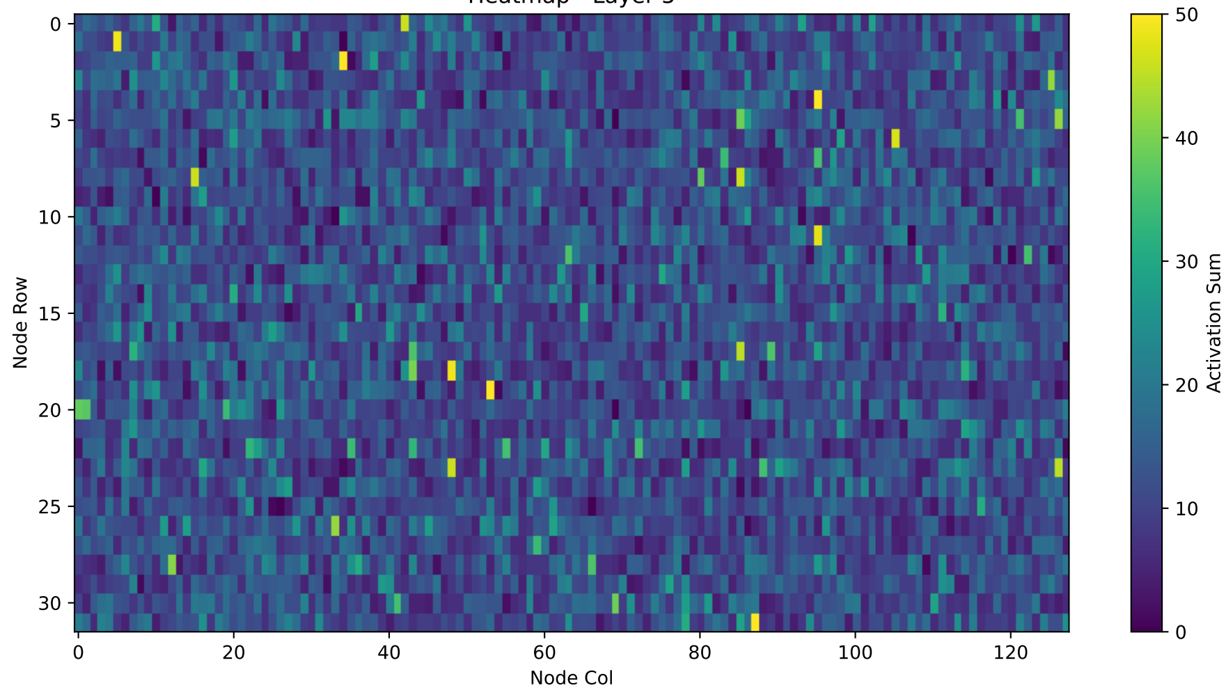
Heatmap - Layer 5
