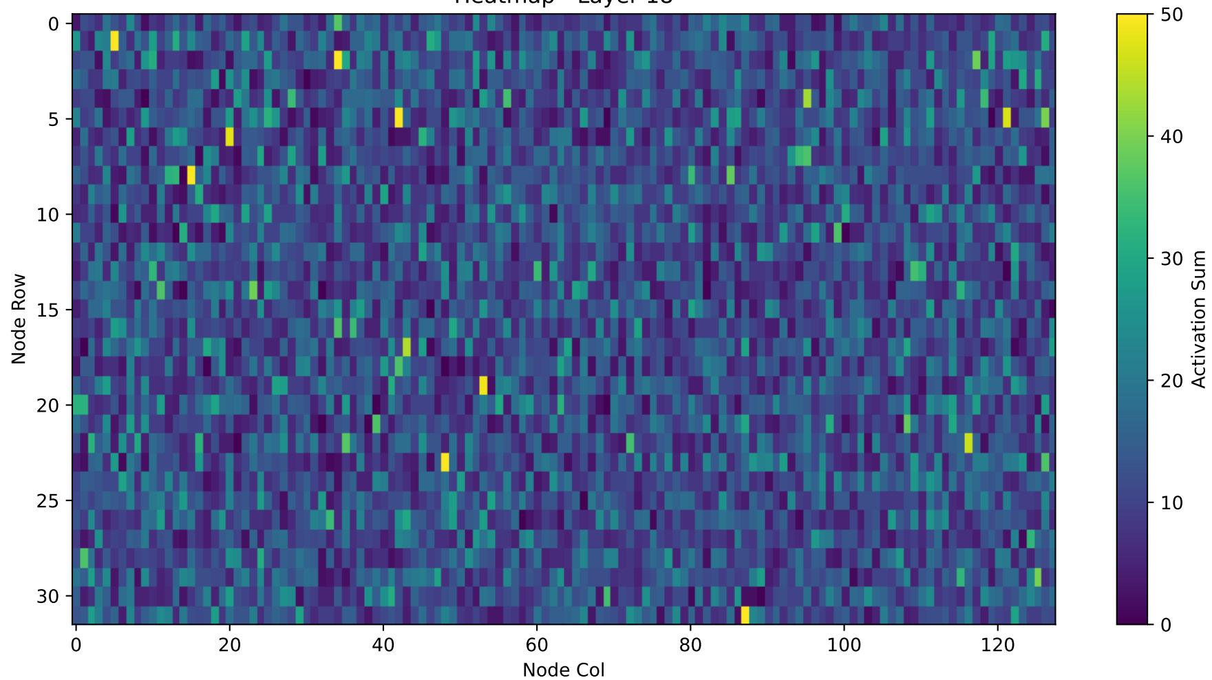
Heatmap - Layer 18
