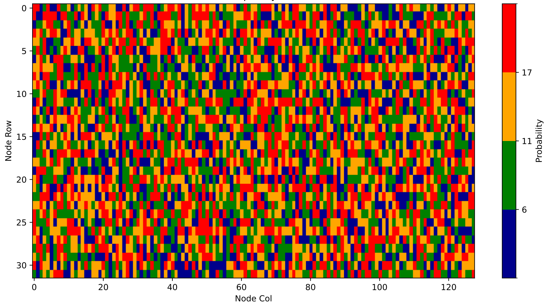
Heatmap - Layer 16
