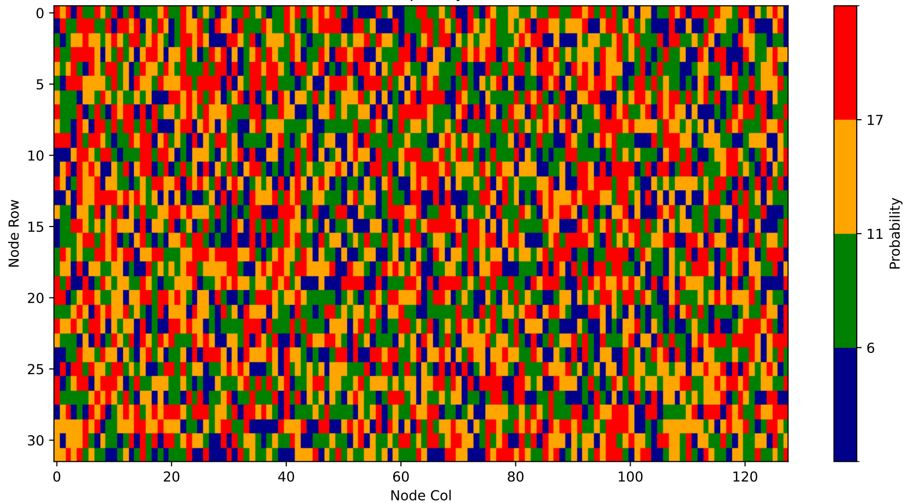
Heatmap - Layer 6
