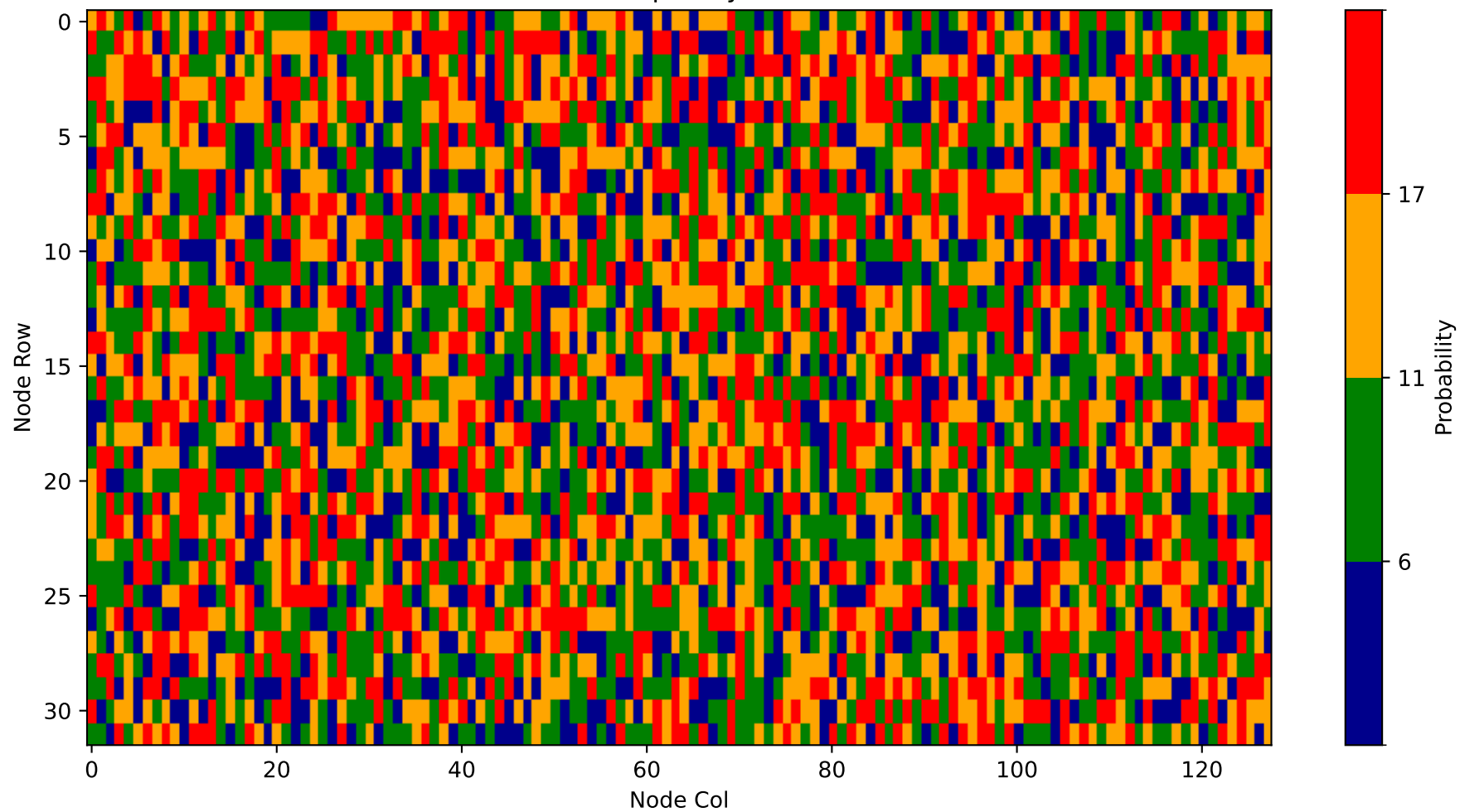
Heatmap - Layer 18
