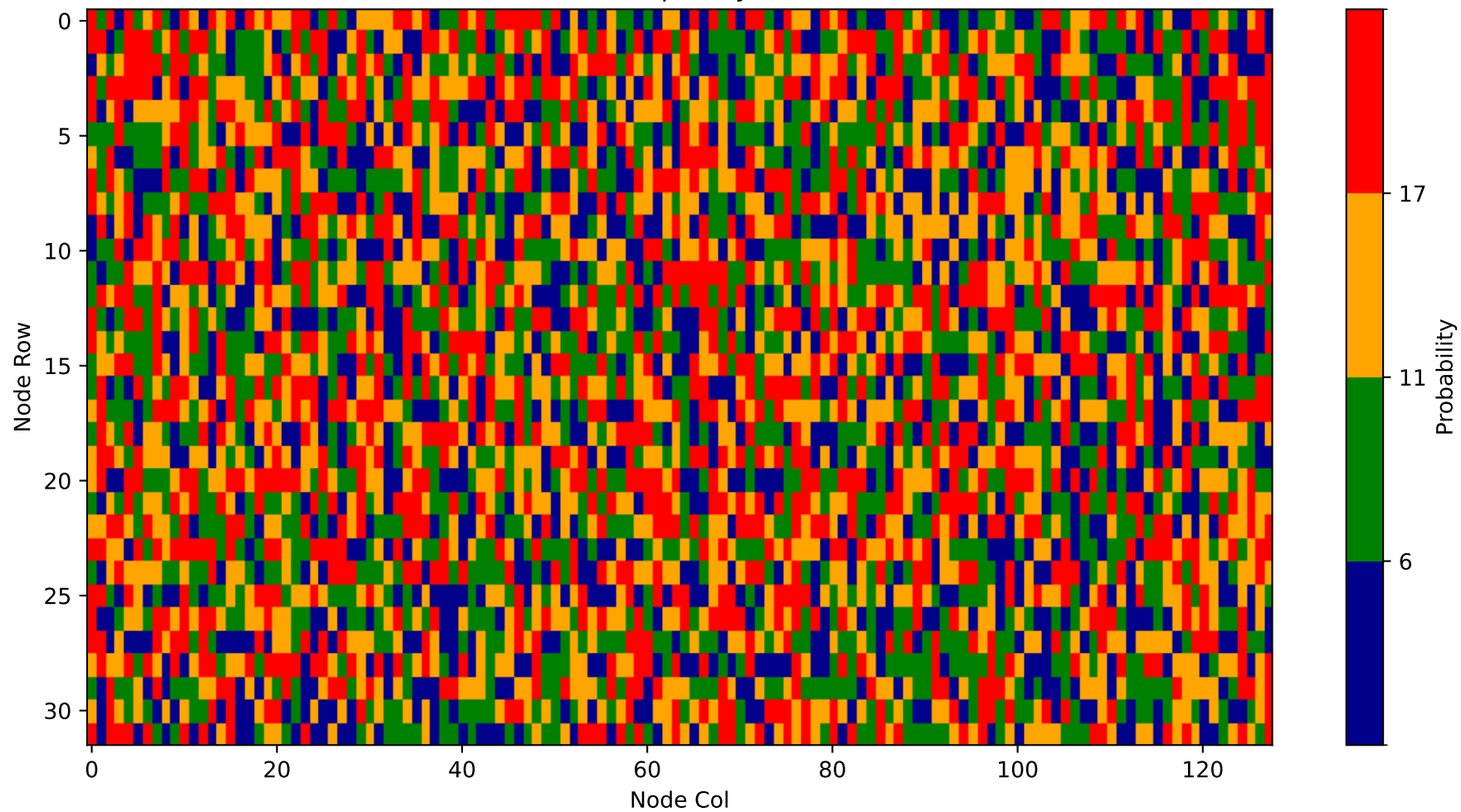
Heatmap - Layer 9
