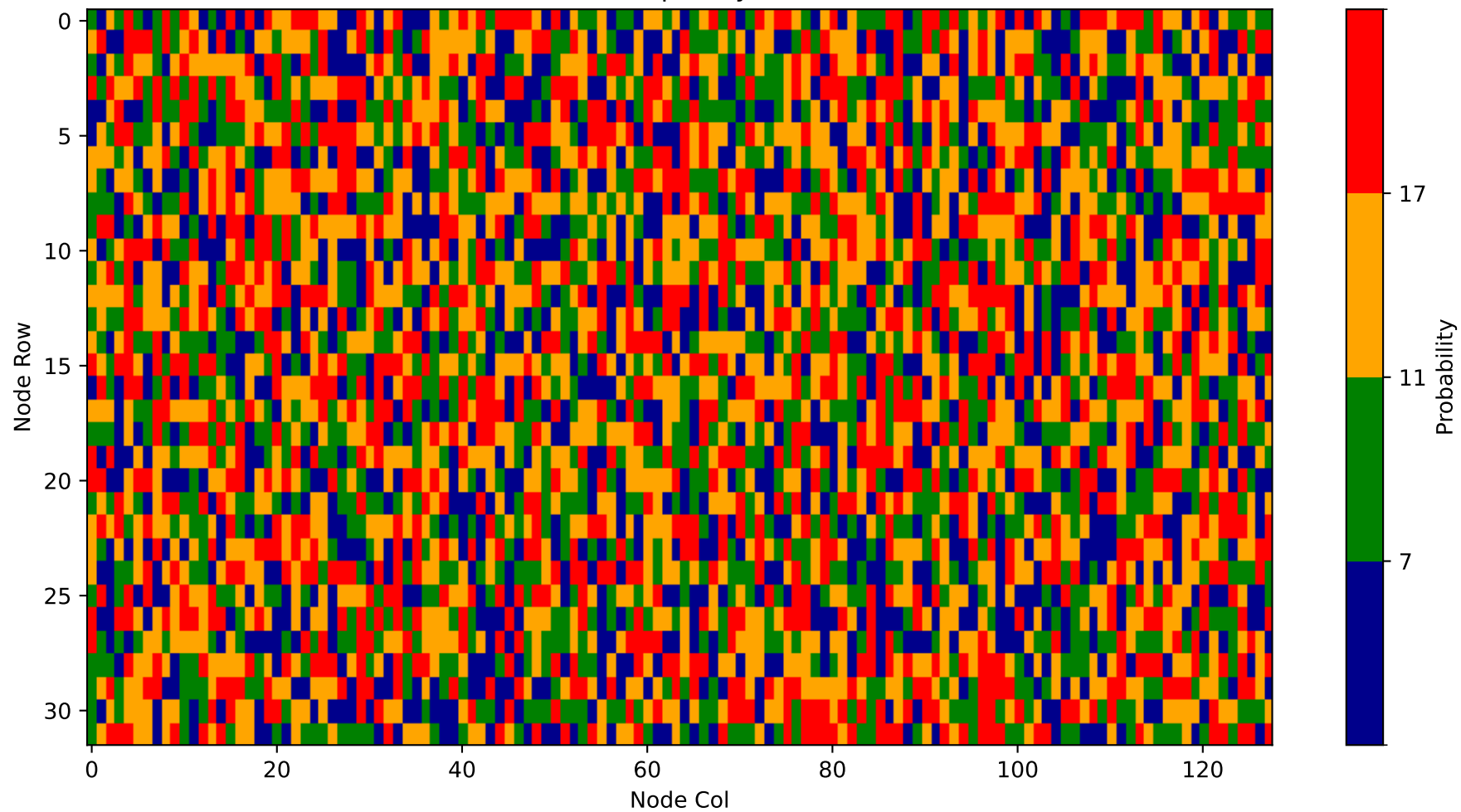
Heatmap - Layer 5
