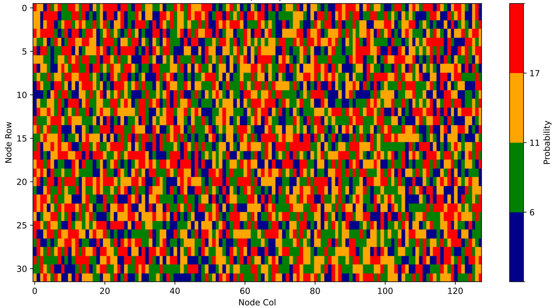
Heatmap - Layer 8
