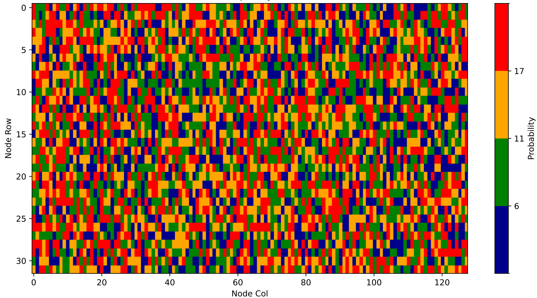
Heatmap - Layer 13
