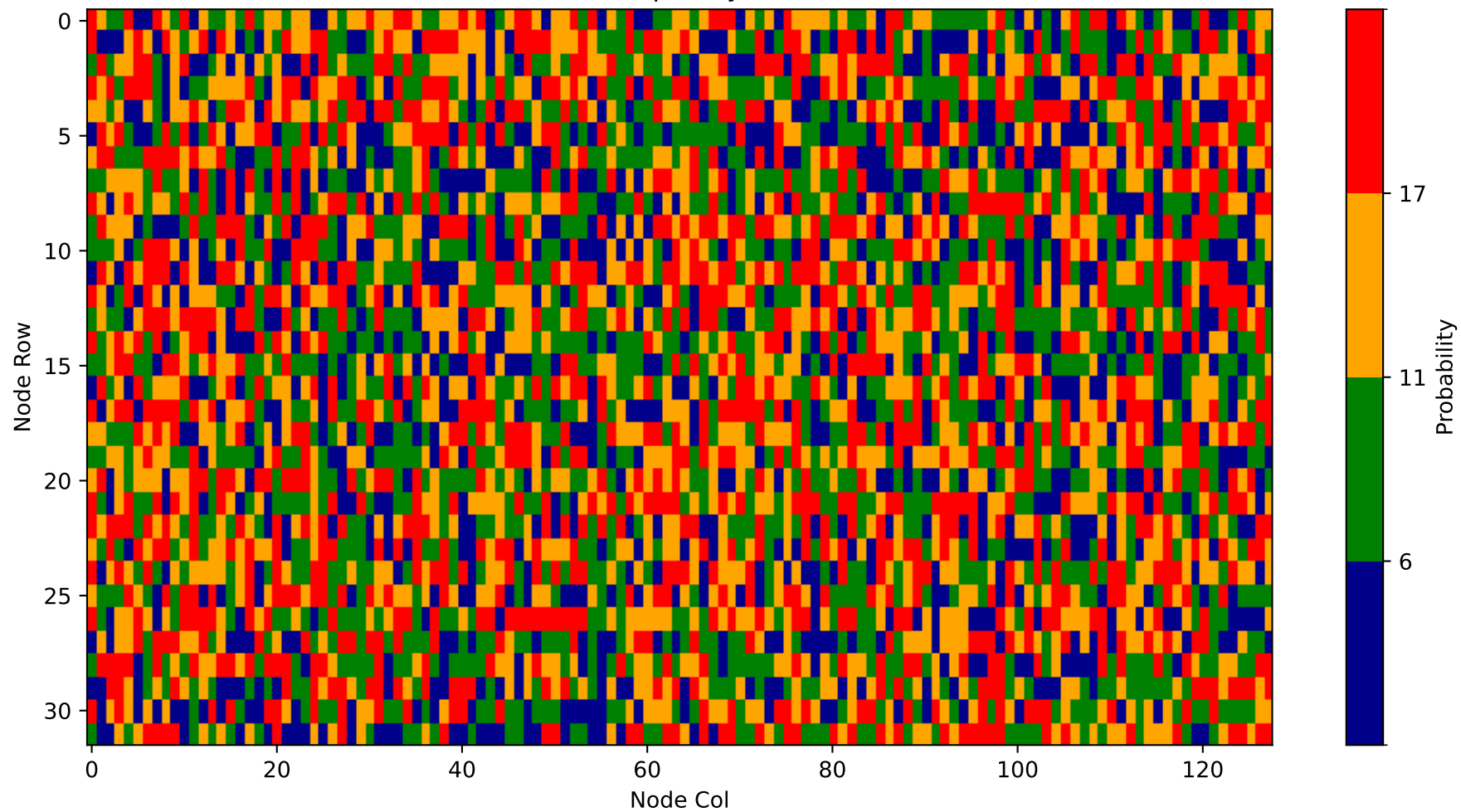
Heatmap - Layer 15
