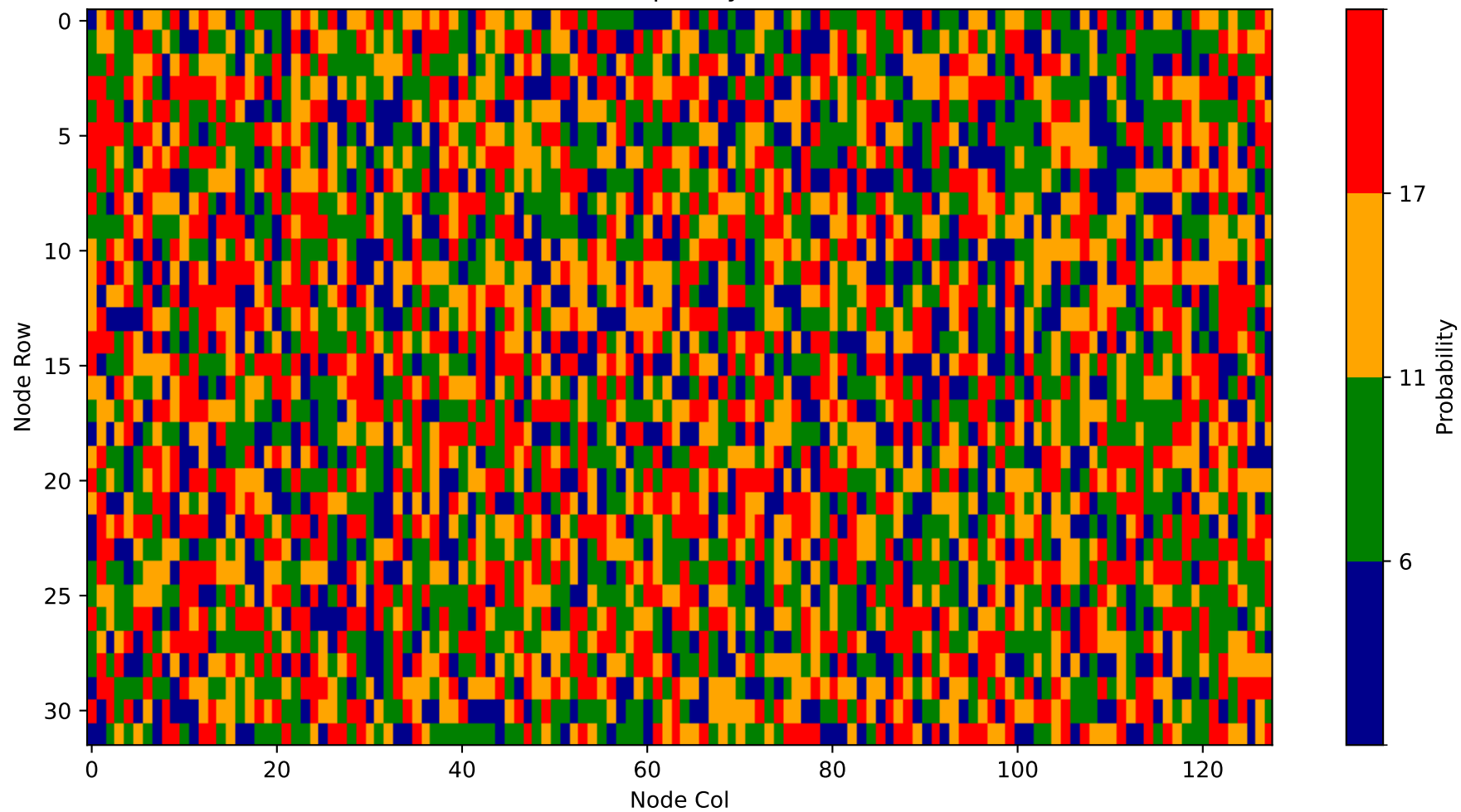
Heatmap - Layer 29
