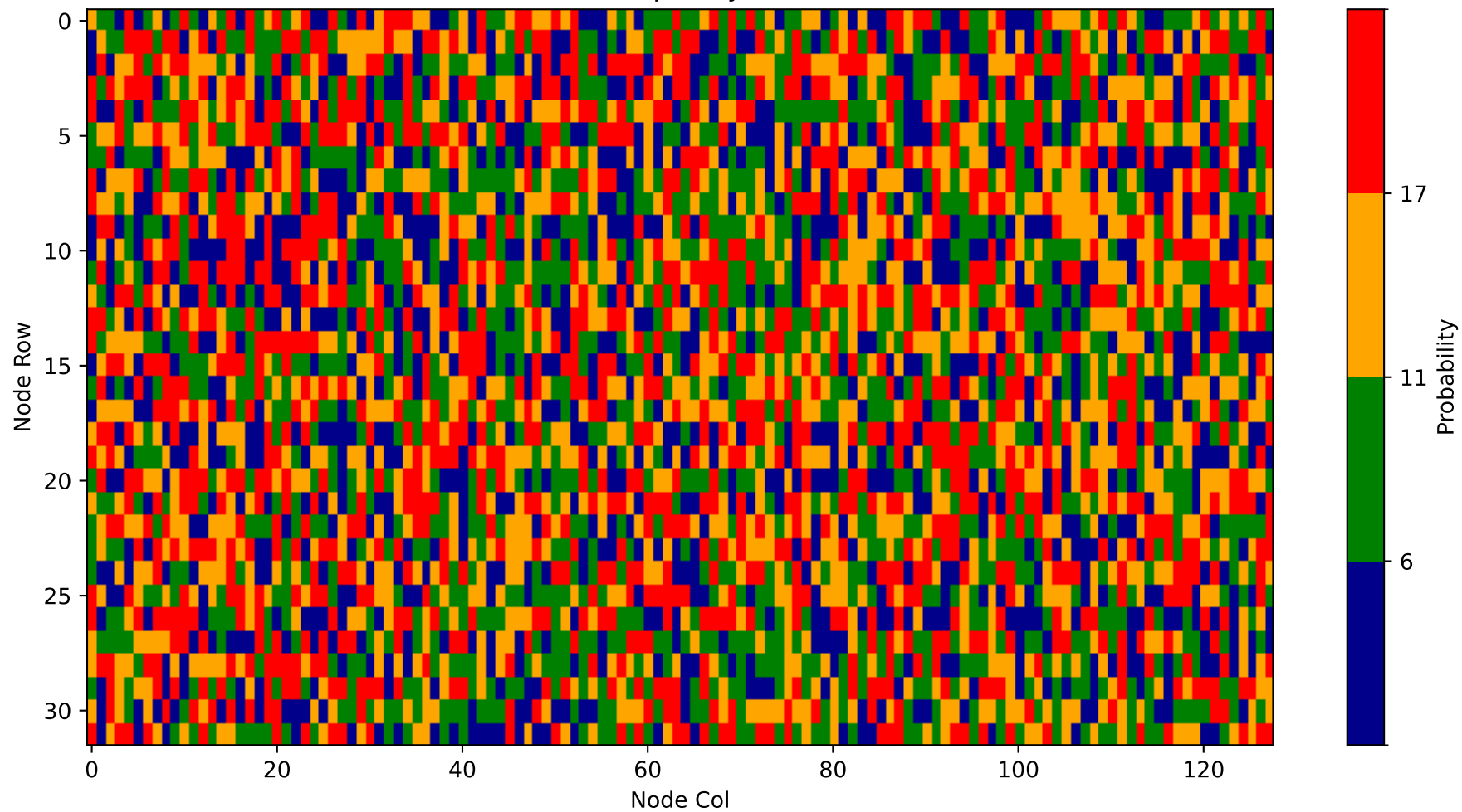
Heatmap - Layer 11
