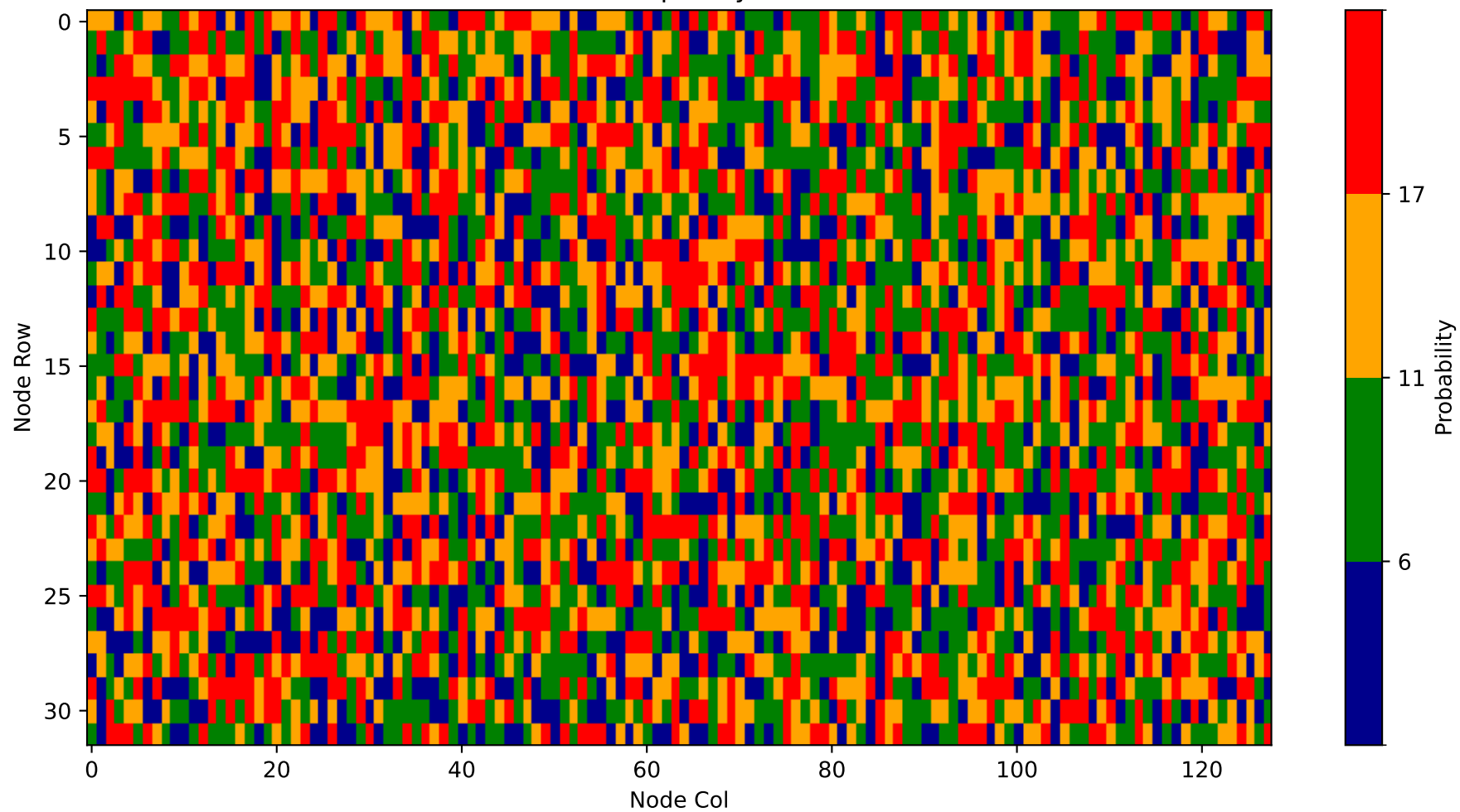
Heatmap - Layer 7
