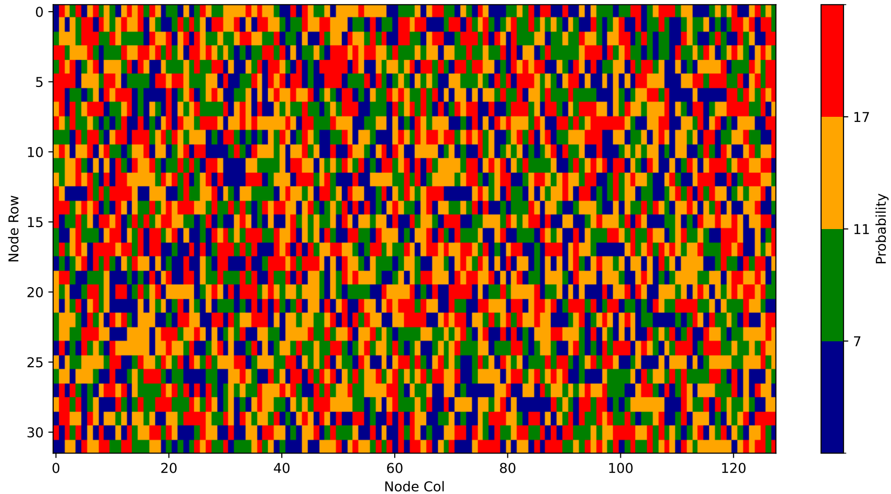
Heatmap - Layer 24
