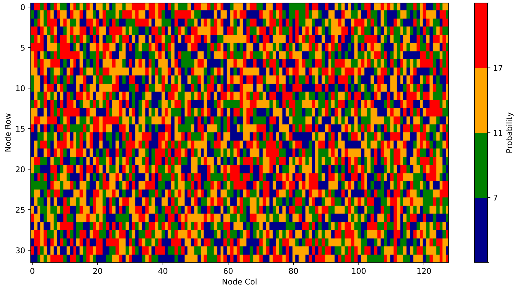
Heatmap - Layer 22
