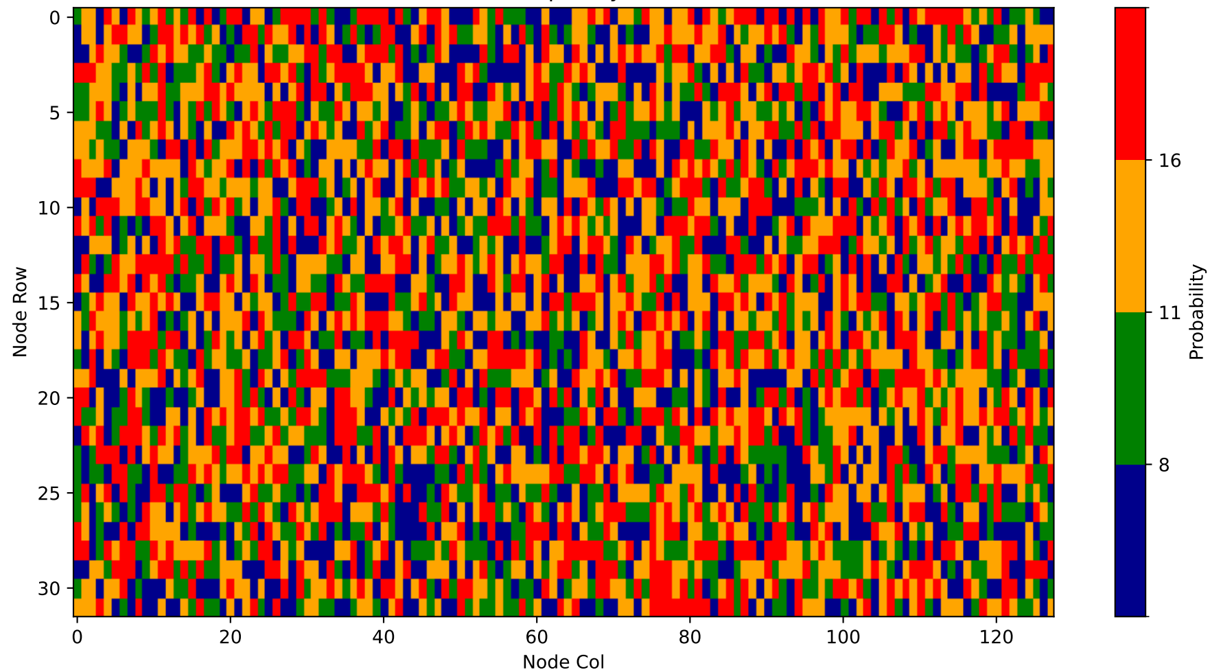
Heatmap - Layer 3
