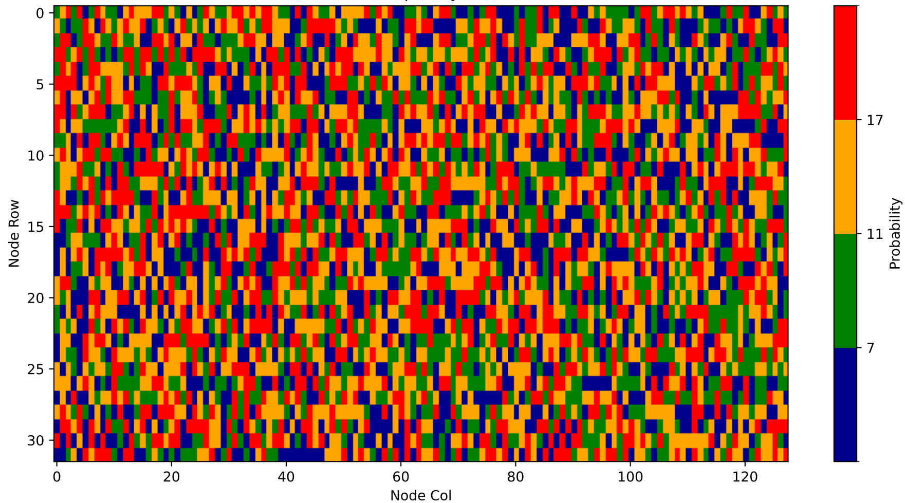
Heatmap - Layer 23
