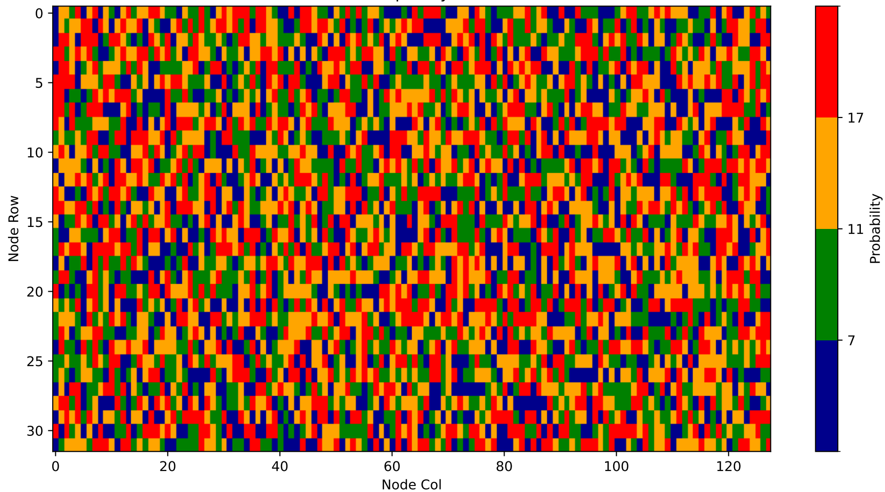
Heatmap - Layer 25
