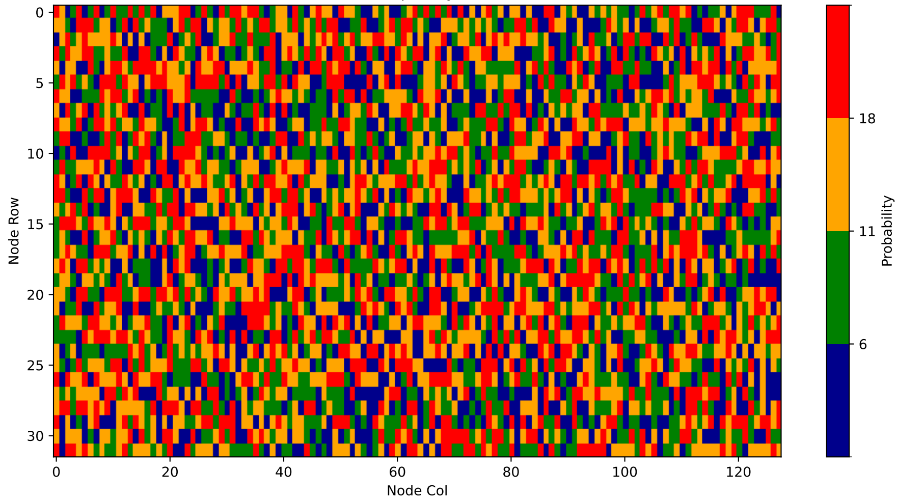
Heatmap - Layer 12
