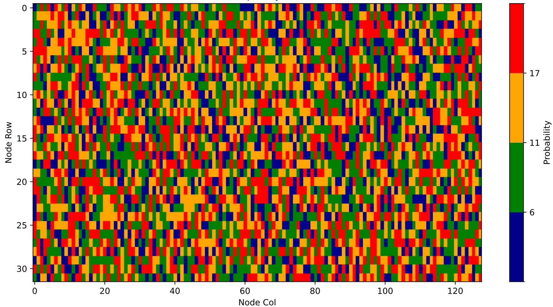
Heatmap - Layer 30
