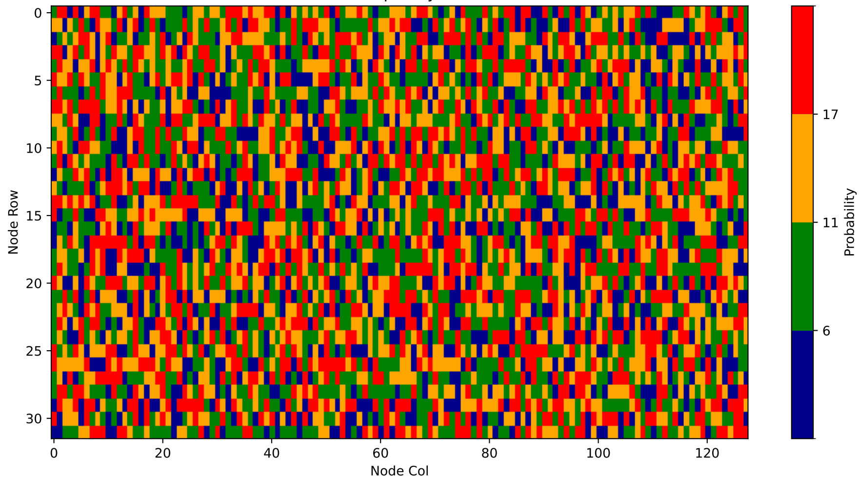
Heatmap - Layer 20
