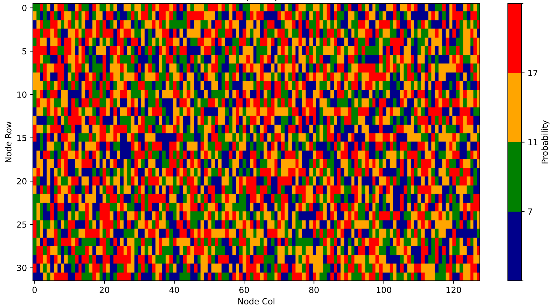
Heatmap - Layer 21
