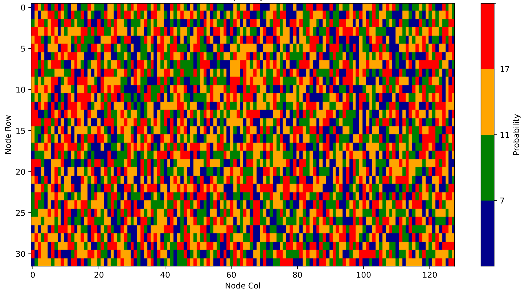
Heatmap - Layer 27
