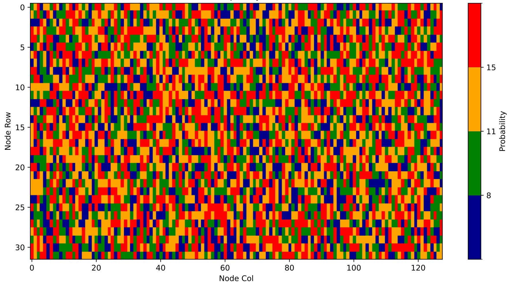
Heatmap - Layer 1
