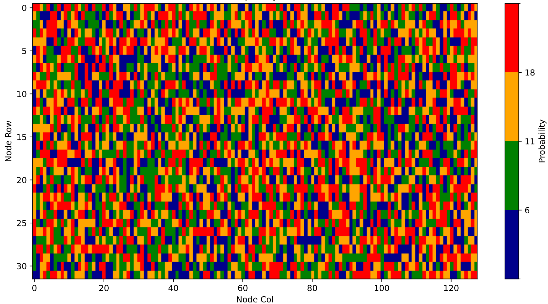
Heatmap - Layer 14
