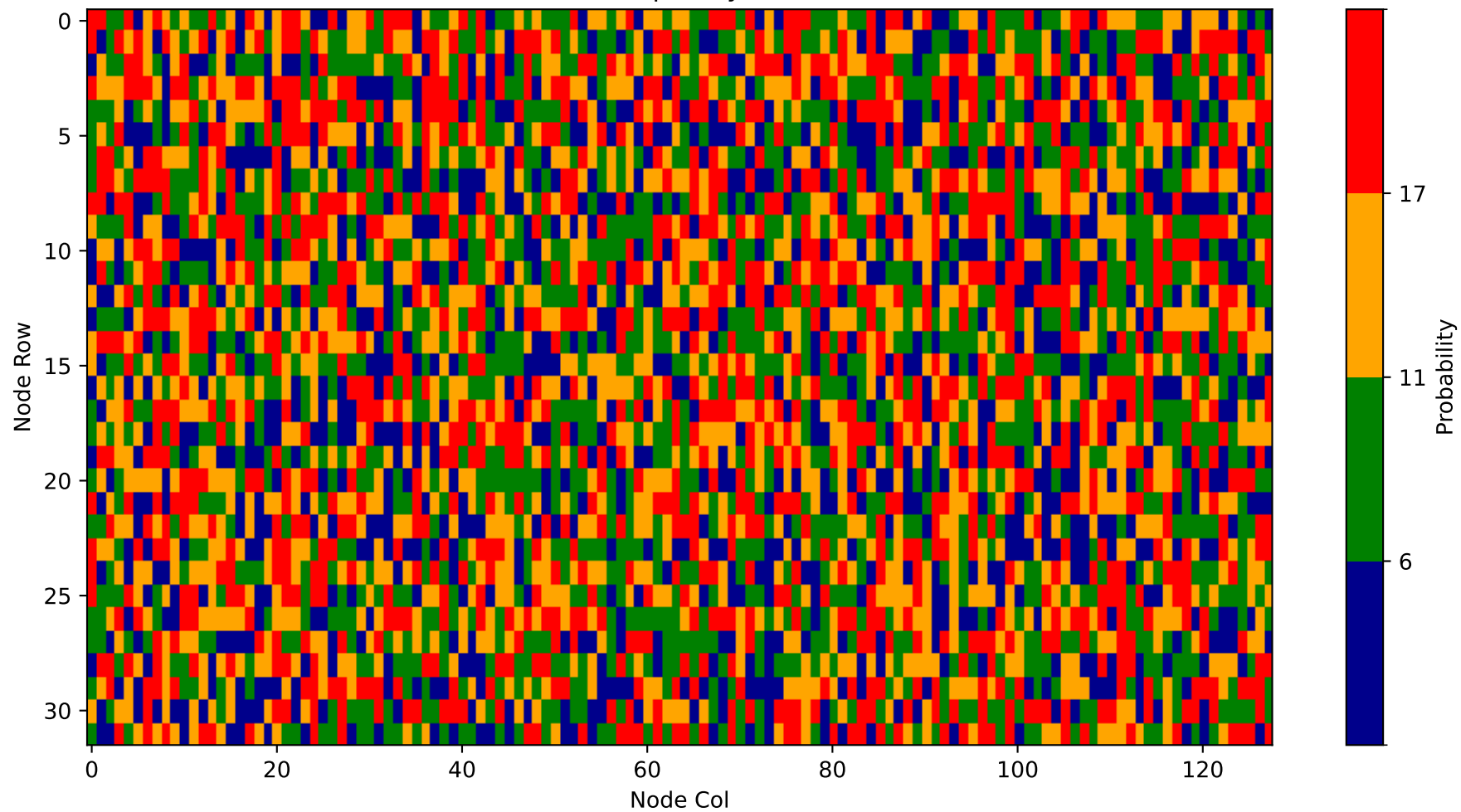
Heatmap - Layer 17
