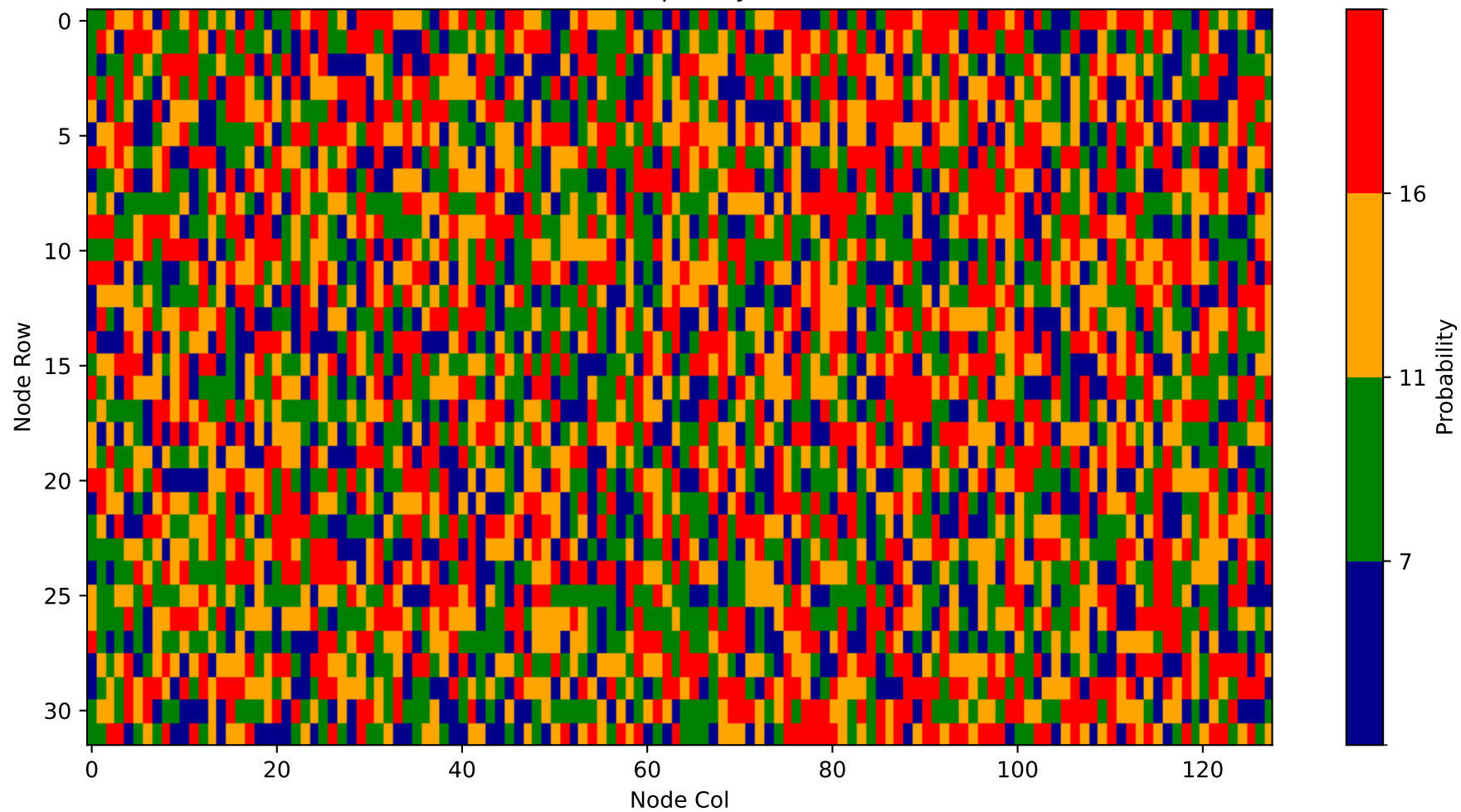
Heatmap - Layer 4
