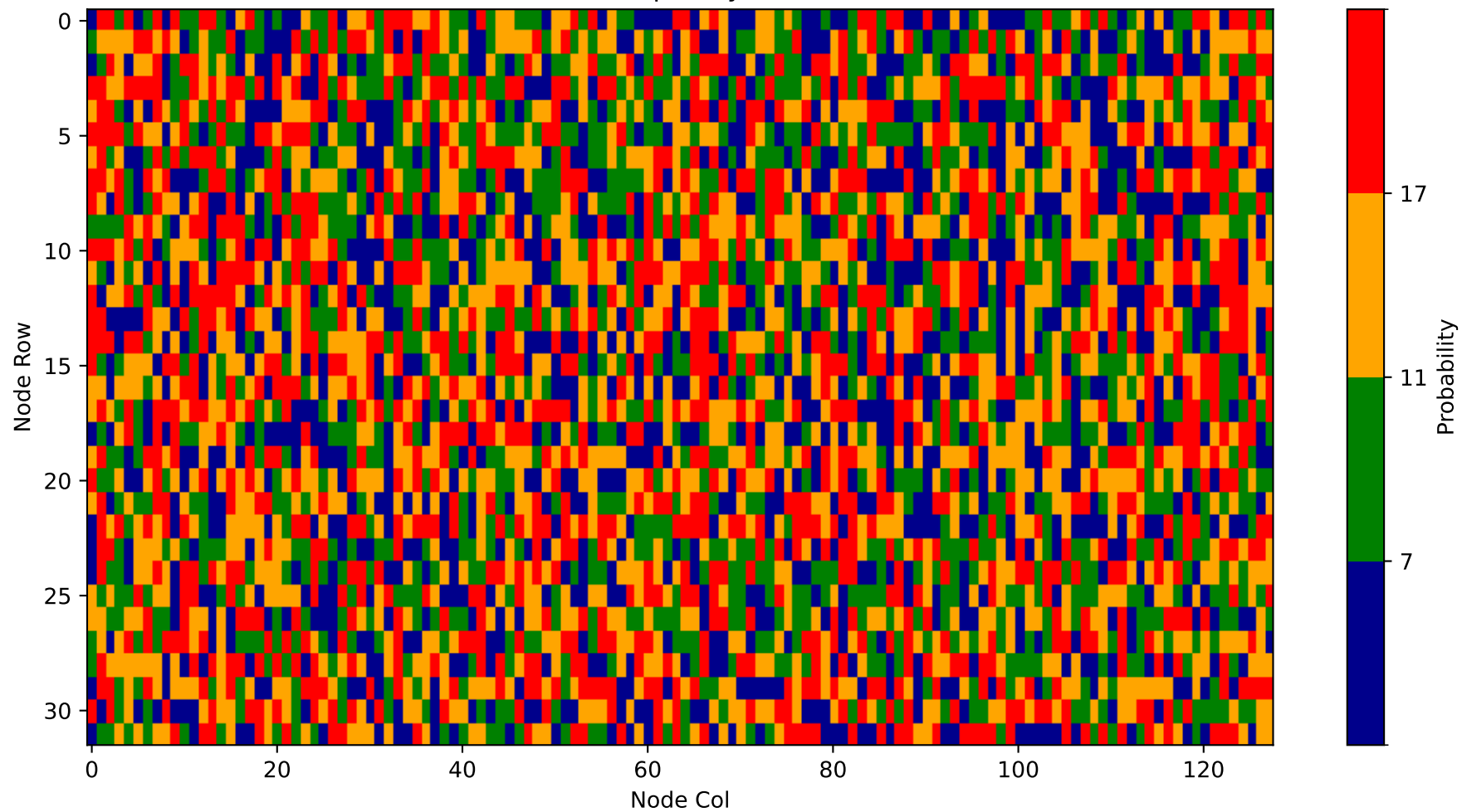
Heatmap - Layer 28
