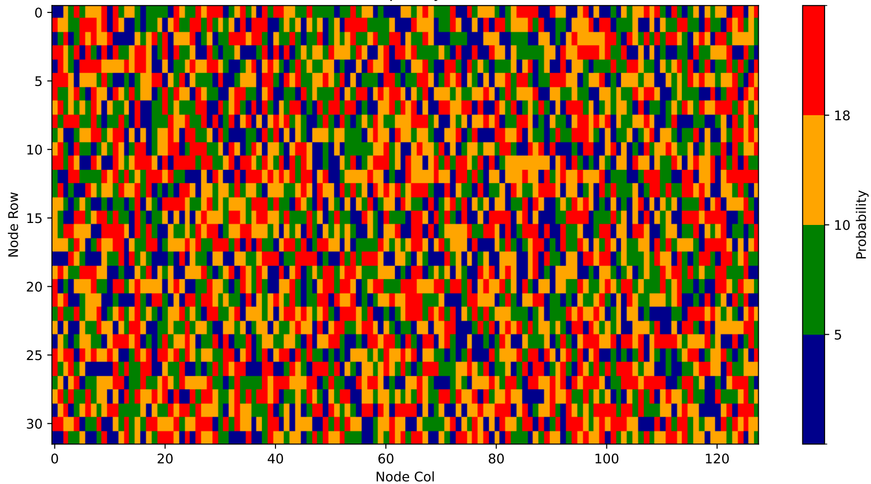
Heatmap - Layer 31
