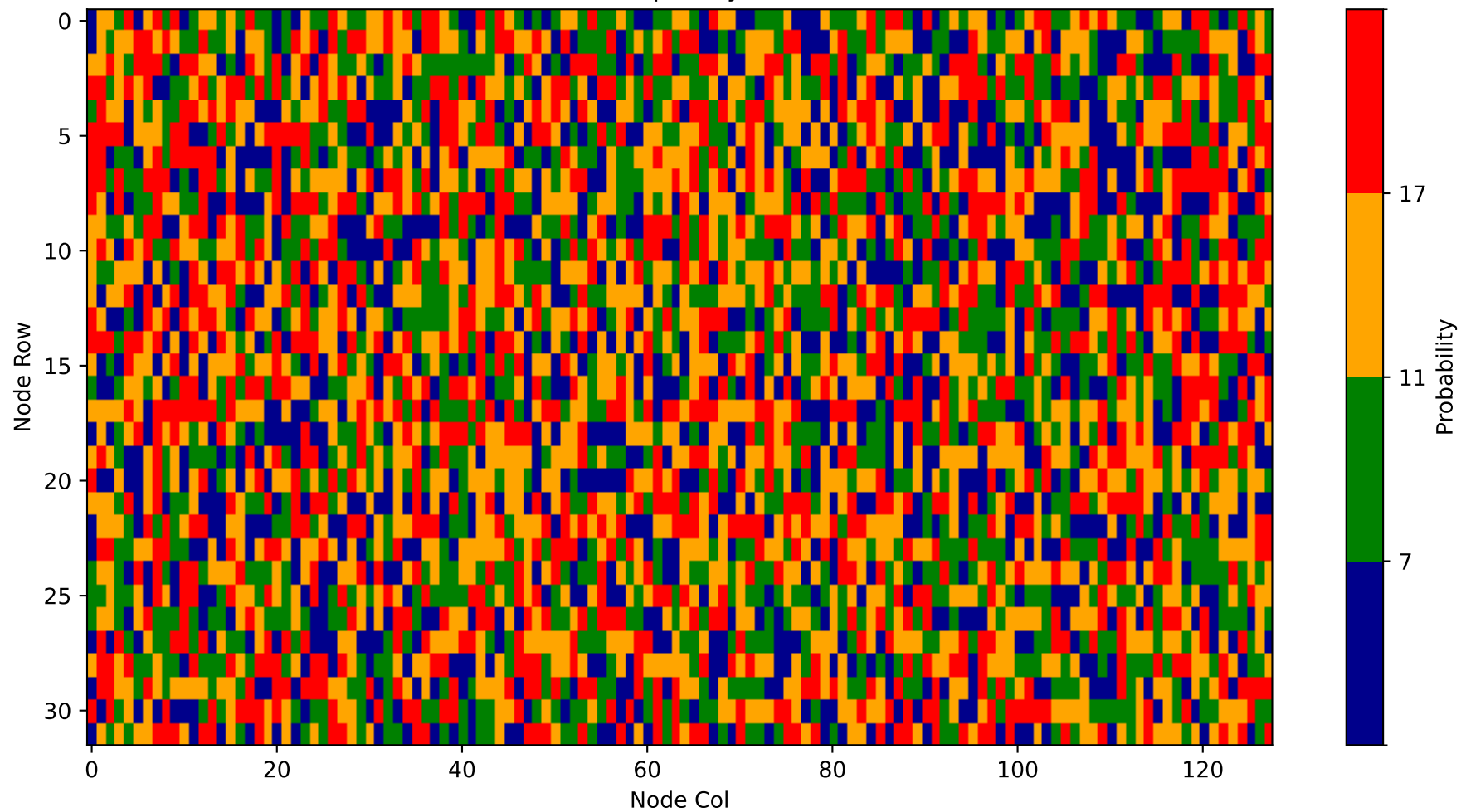
Heatmap - Layer 26
