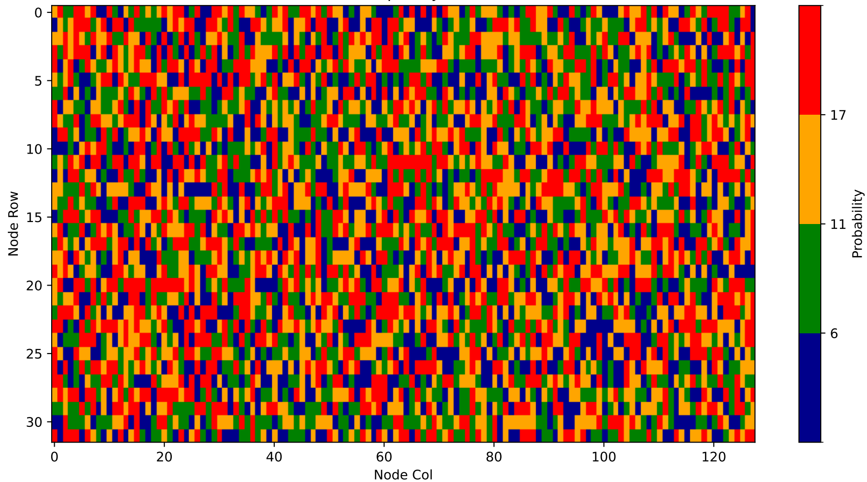
Heatmap - Layer 10
