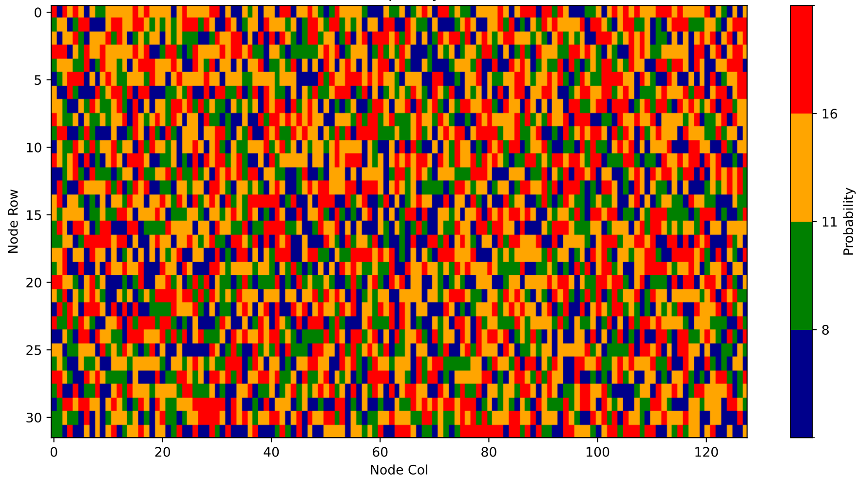
Heatmap - Layer 2
