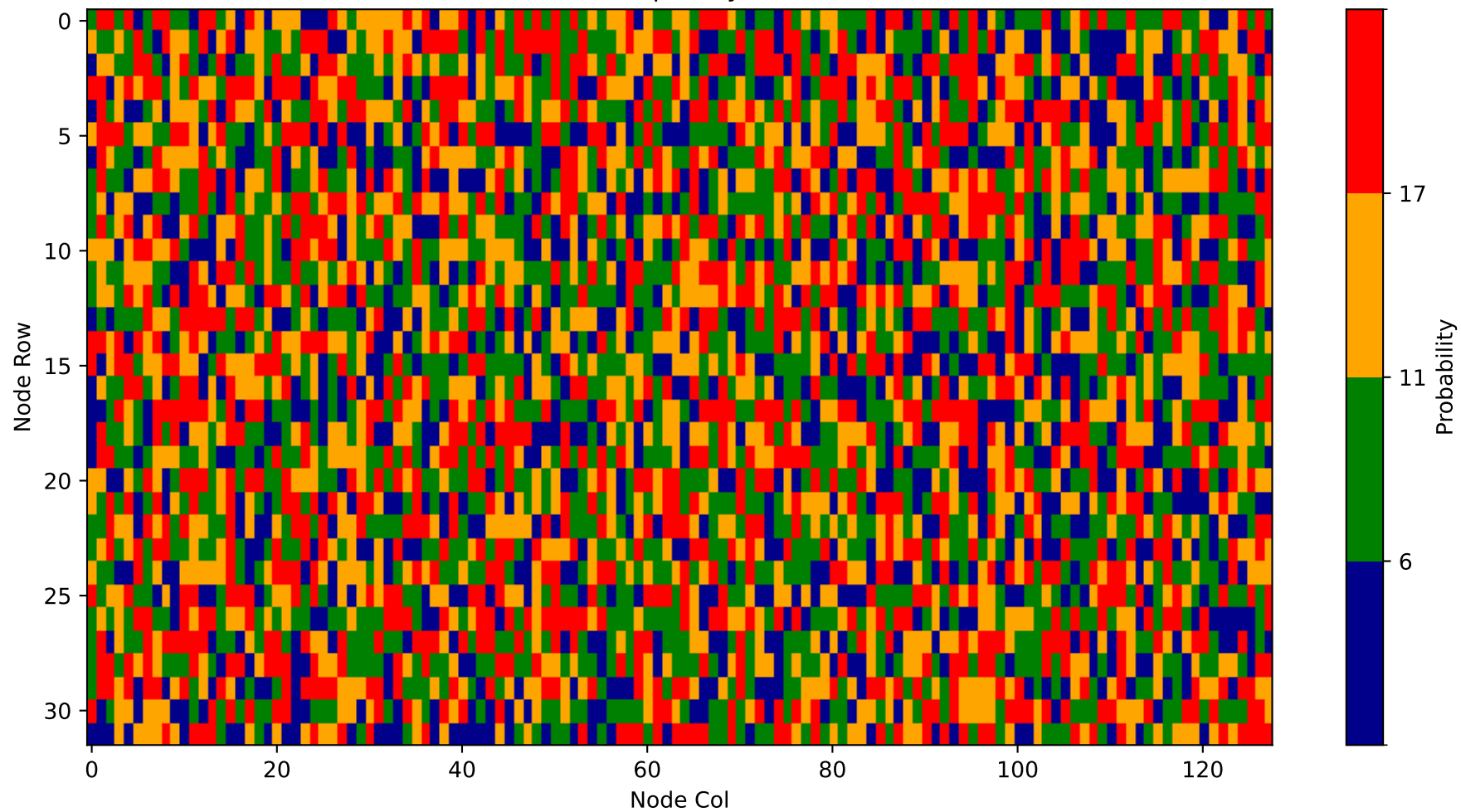
Heatmap - Layer 19
