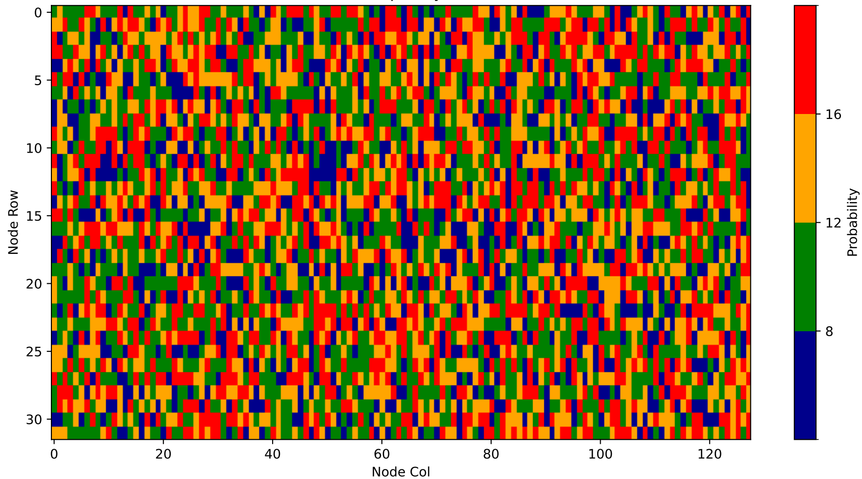
Heatmap - Layer 0
