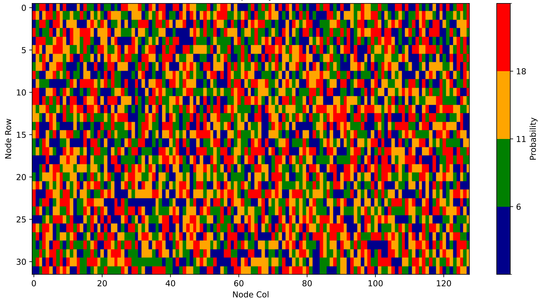
Heatmap - Layer 32
