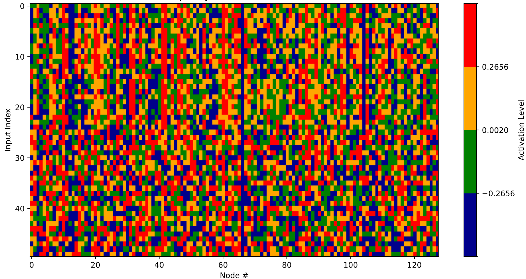
Heatmap - Layer 29 (Nodes 3200-3328)
