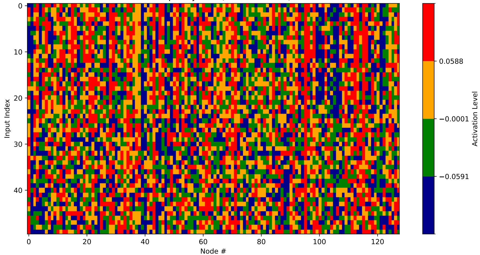
Heatmap - Layer 10 (Nodes 512-640)
