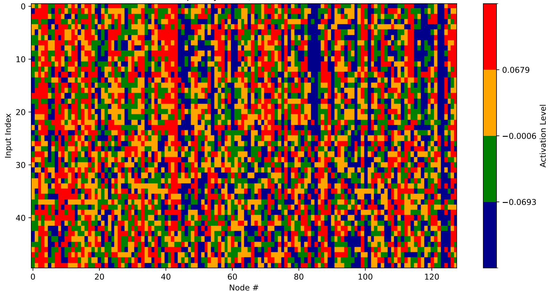
Heatmap - Layer 14 (Nodes 2176-2304)
