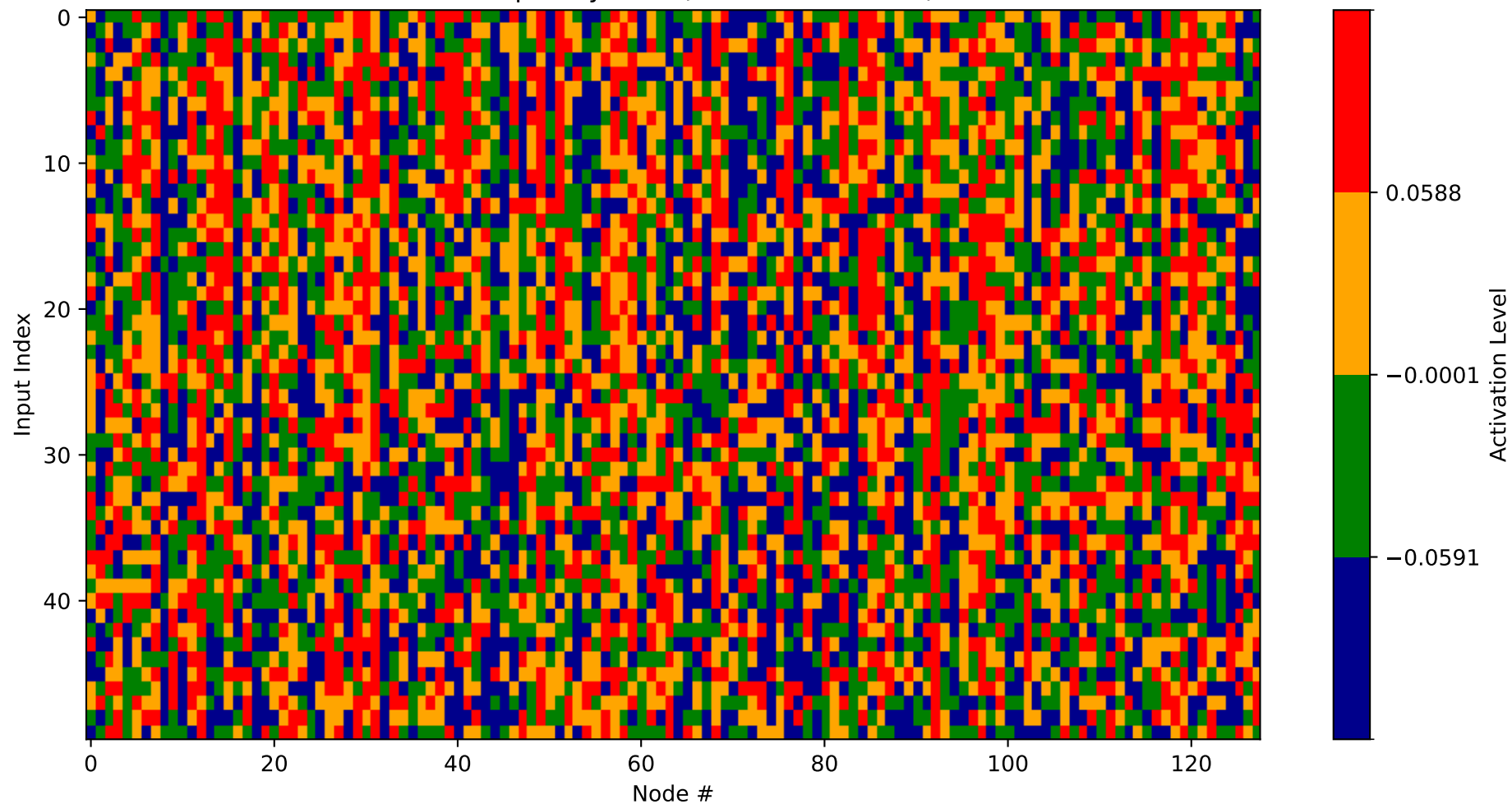
Heatmap - Layer 10 (Nodes 3712-3840)
