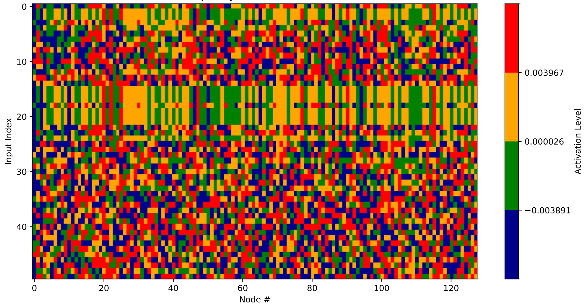
Heatmap - Layer 0 (Nodes 896-1024)
