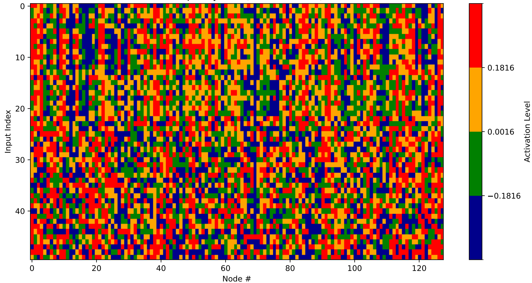
Heatmap - Layer 25 (Nodes 640-768)
