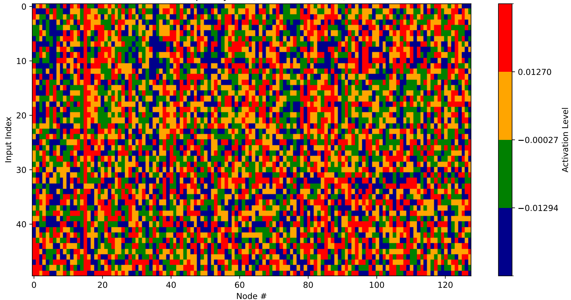
Heatmap - Layer 2 (Nodes 1024-1152)
