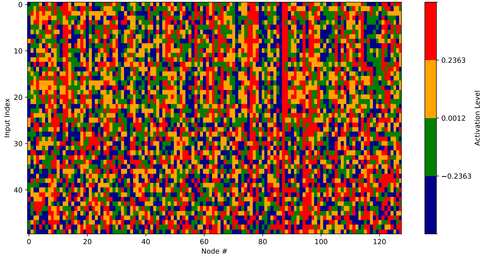
Heatmap - Layer 28 (Nodes 3968-4096)
