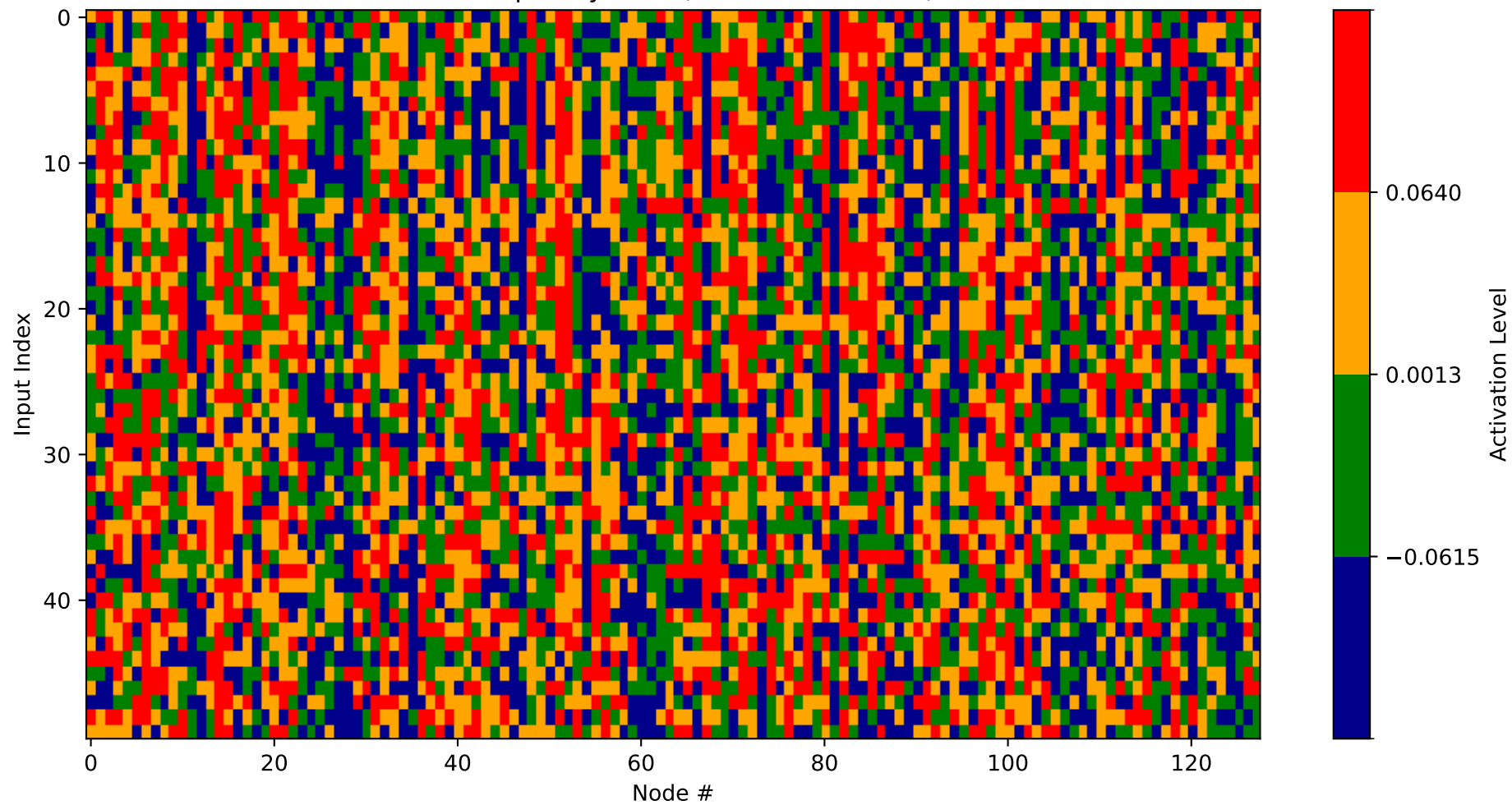
Heatmap - Layer 12 (Nodes 1920-2048)
