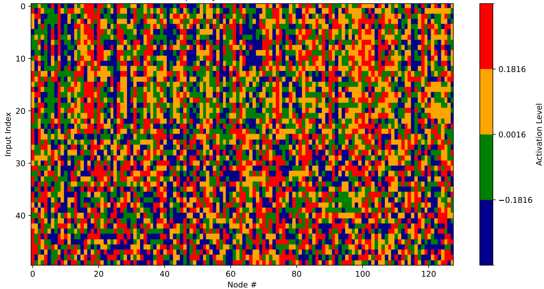
Heatmap - Layer 25 (Nodes 3840-3968)
