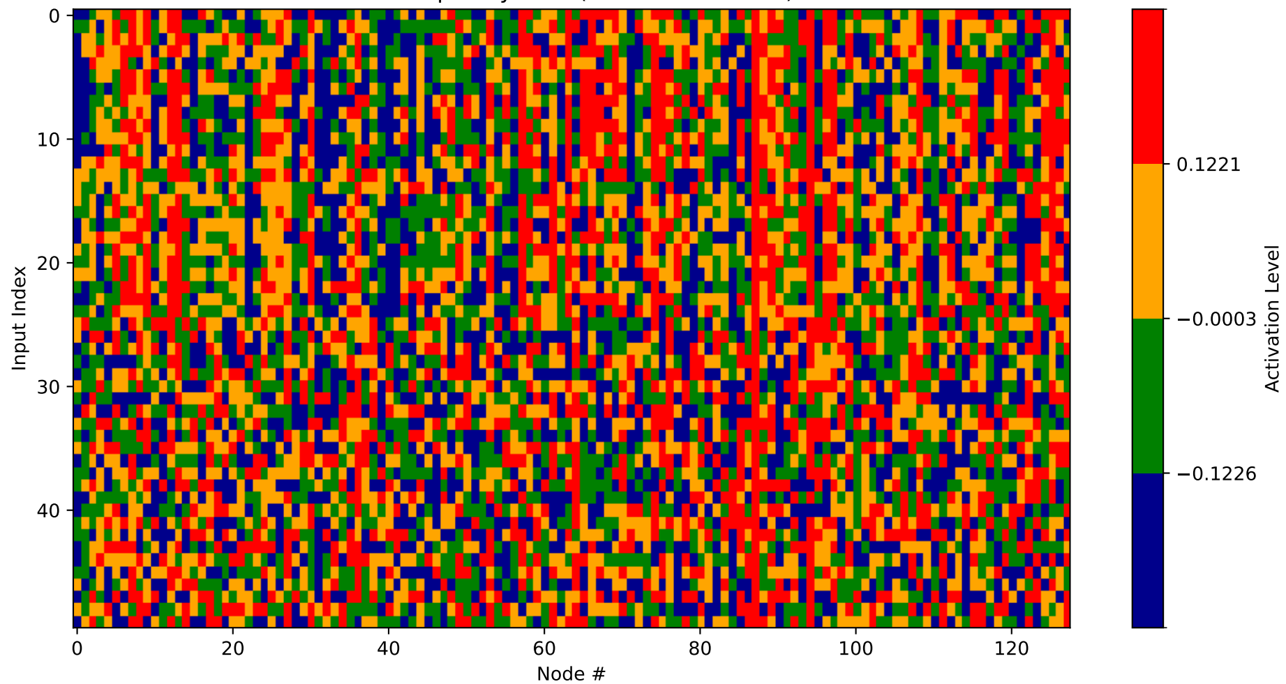
Heatmap - Layer 20 (Nodes 3968-4096)
