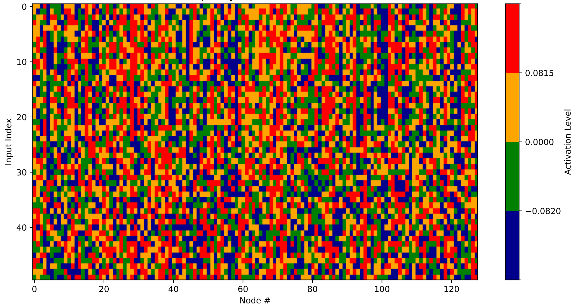
Heatmap - Layer 16 (Nodes 512-640)
