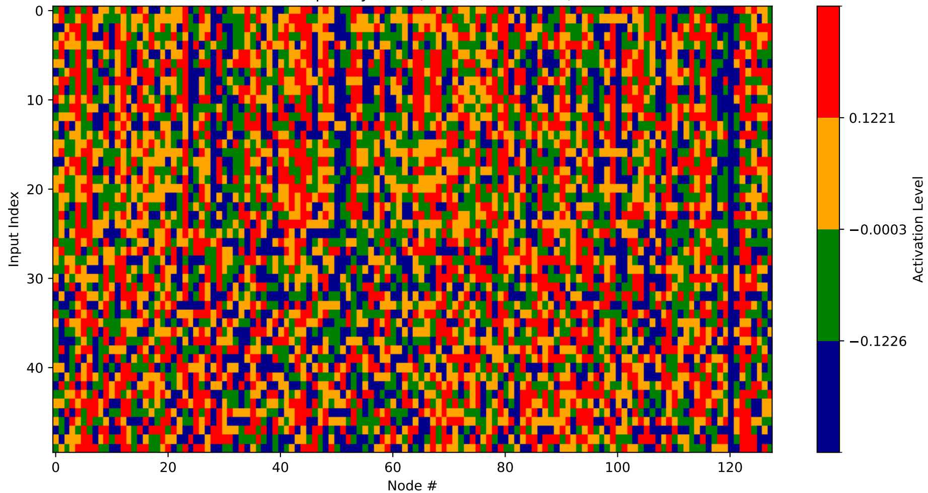
Heatmap - Layer 20 (Nodes 1536-1664)
