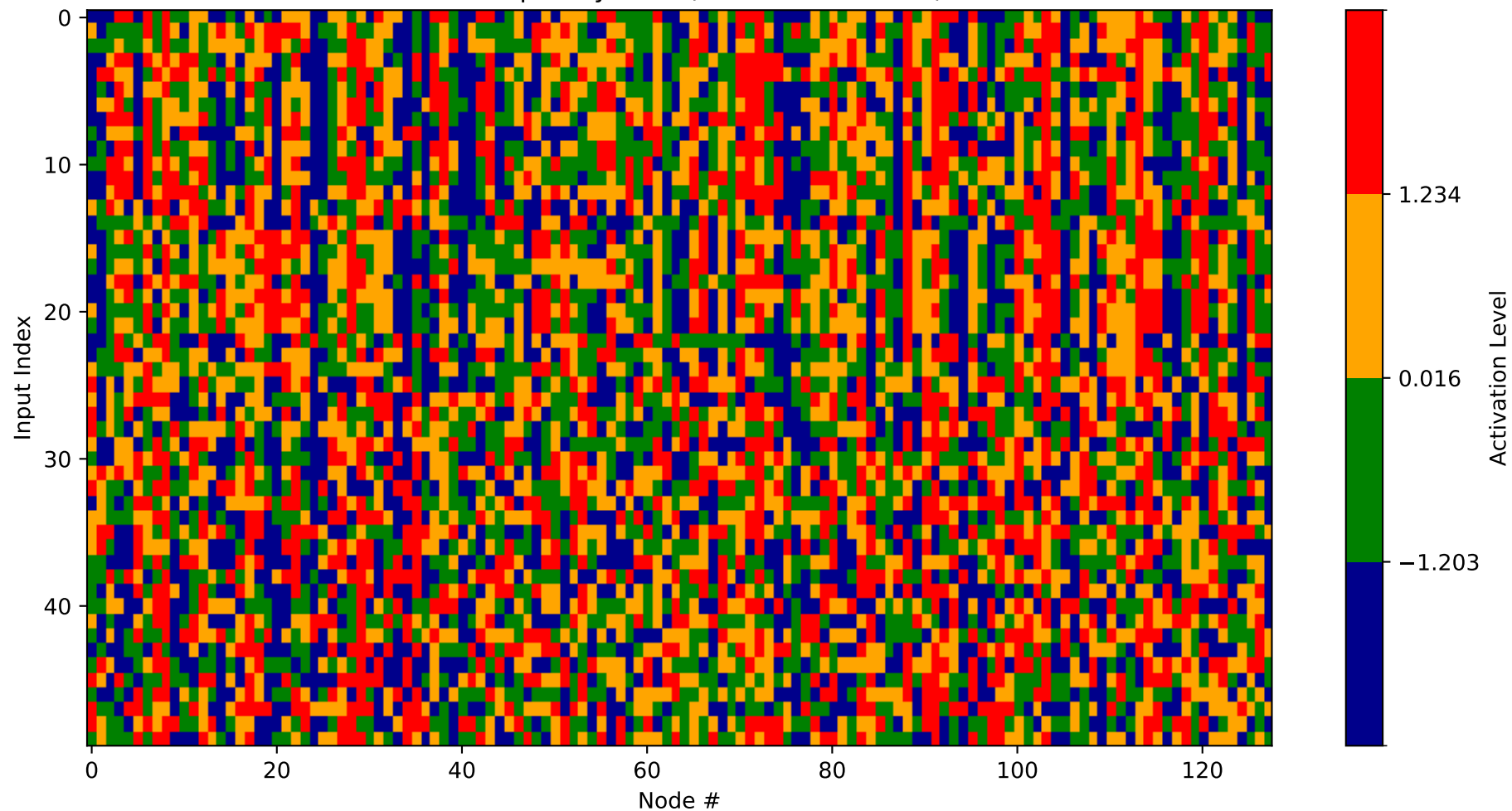
Heatmap - Layer 32 (Nodes 2560-2688)
