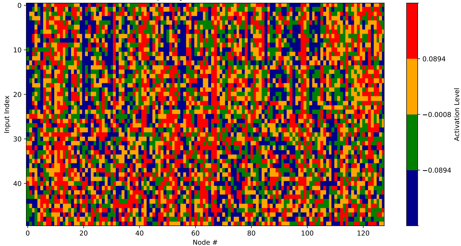
Heatmap - Layer 17 (Nodes 1664-1792)
