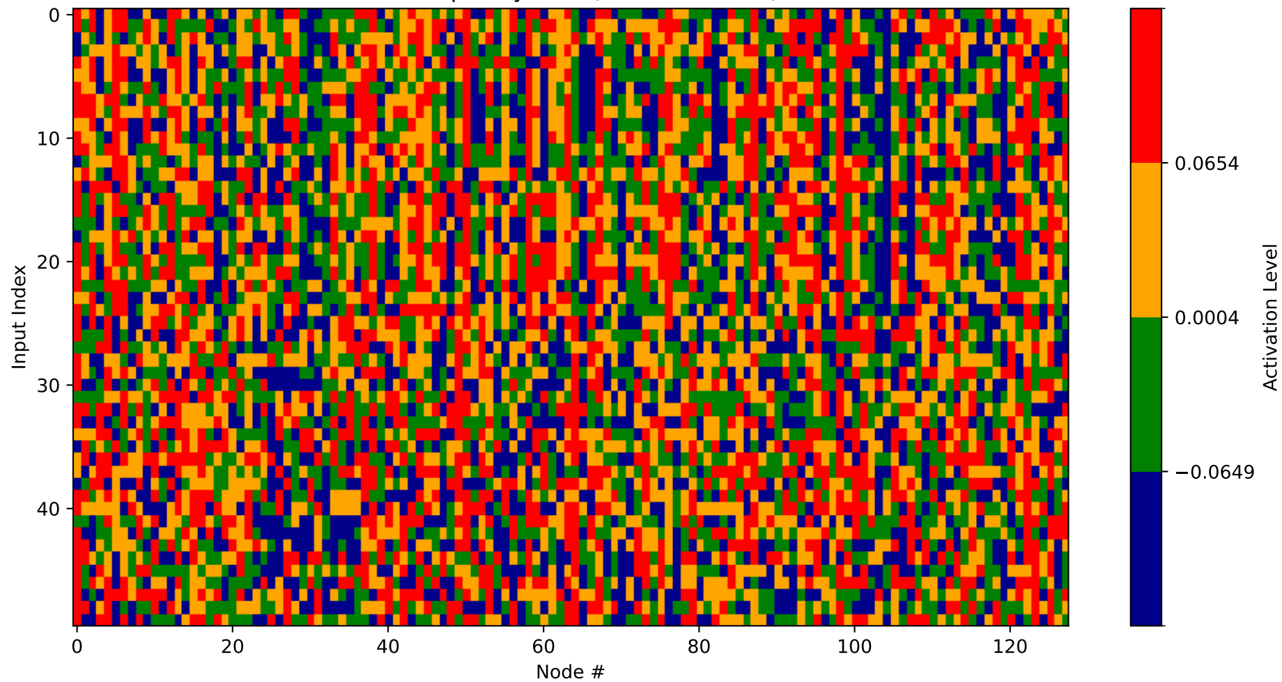
Heatmap - Layer 13 (Nodes 384-512)
