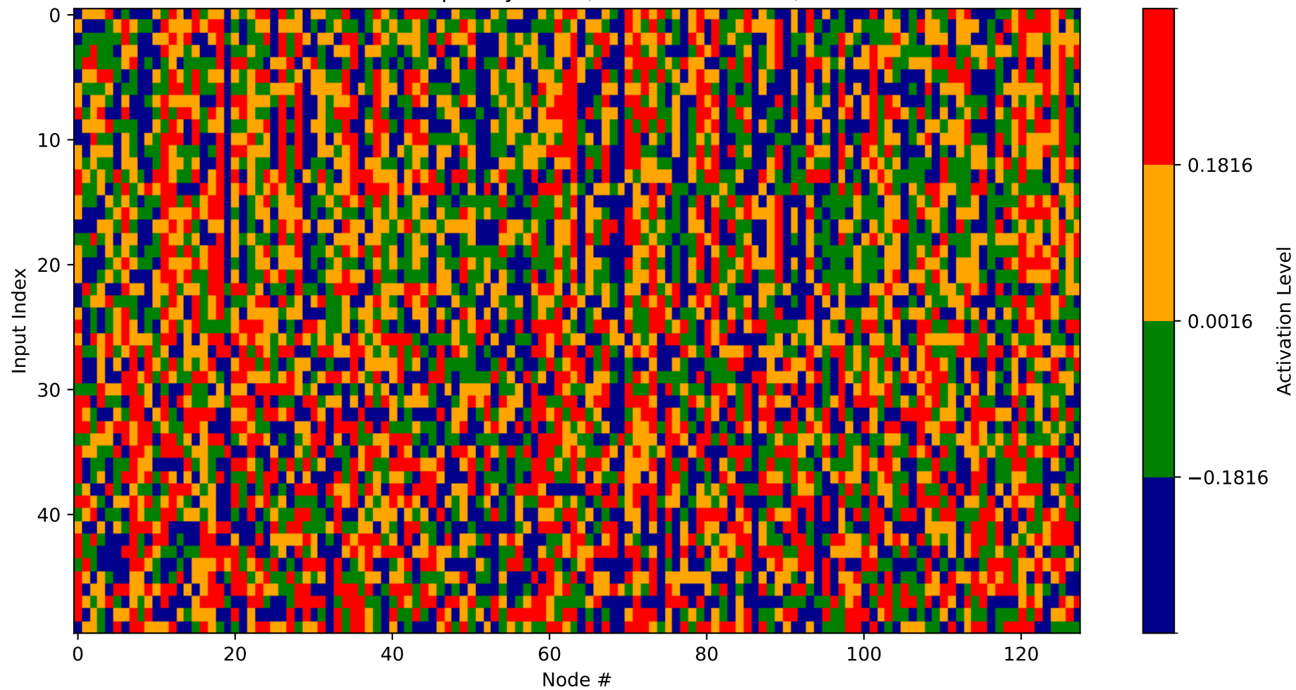
Heatmap - Layer 25 (Nodes 2560-2688)
