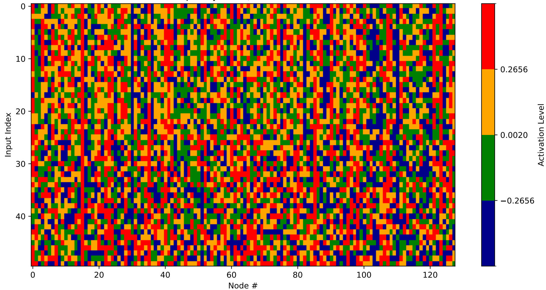
Heatmap - Layer 29 (Nodes 1024-1152)
