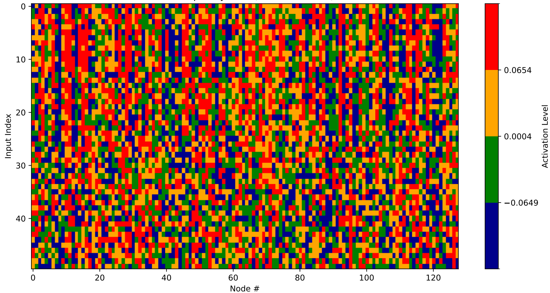
Heatmap - Layer 13 (Nodes 512-640)
