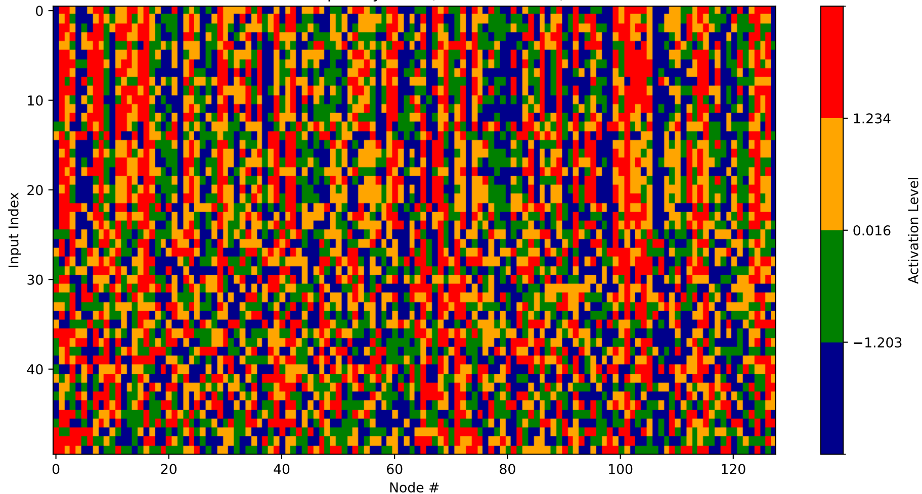
Heatmap - Layer 32 (Nodes 512-640)
