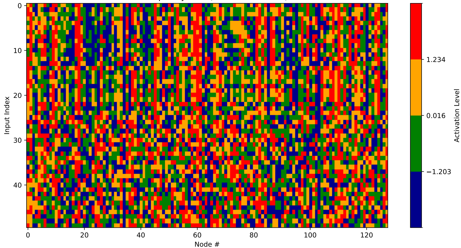
Heatmap - Layer 32 (Nodes 1280-1408)
