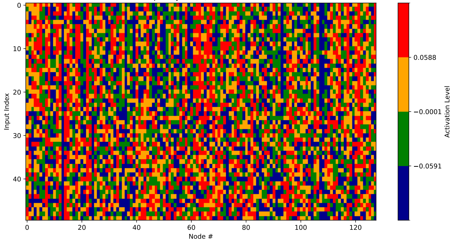
Heatmap - Layer 10 (Nodes 1408-1536)
