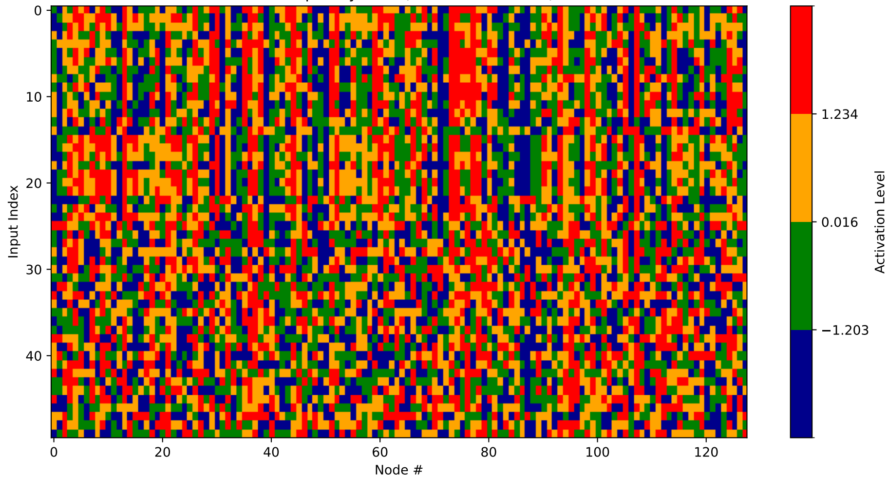
Heatmap - Layer 32 (Nodes 3968-4096)
