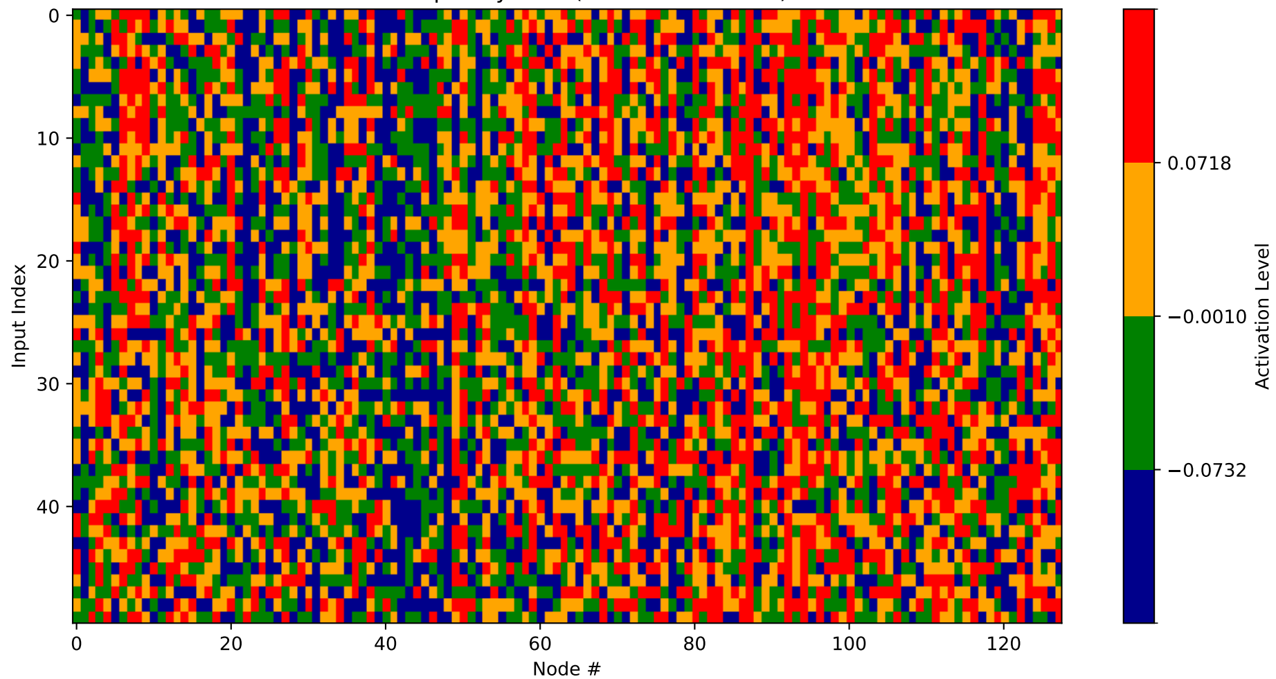
Heatmap - Layer 15 (Nodes 3968-4096)
