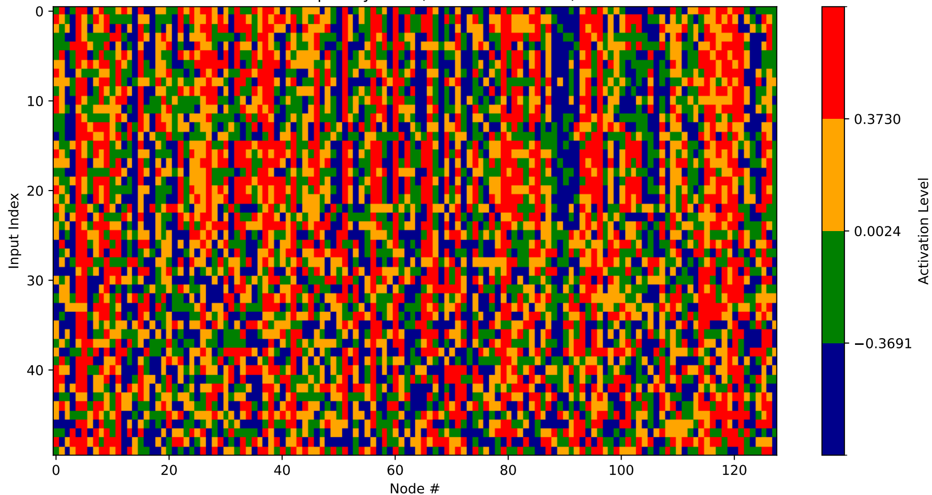
Heatmap - Layer 31 (Nodes 1920-2048)
