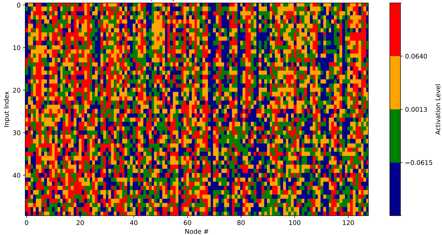
Heatmap - Layer 12 (Nodes 2560-2688)
