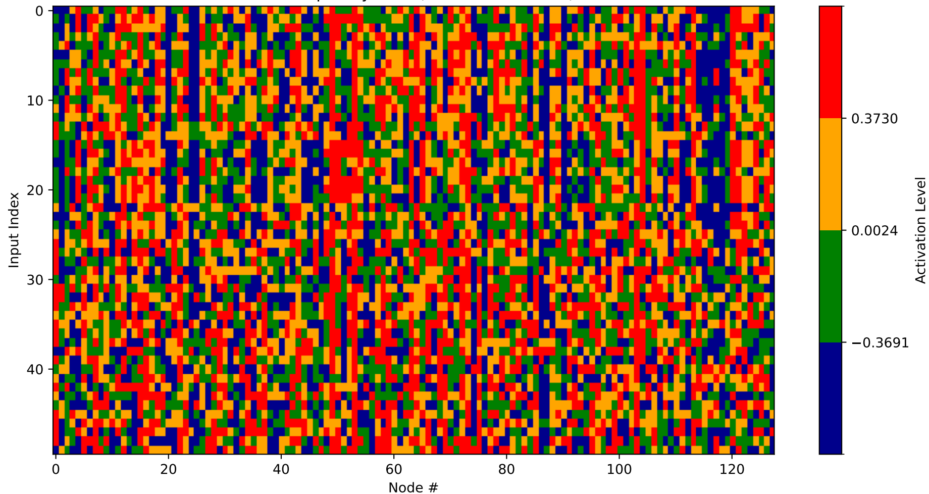
Heatmap - Layer 31 (Nodes 2560-2688)
