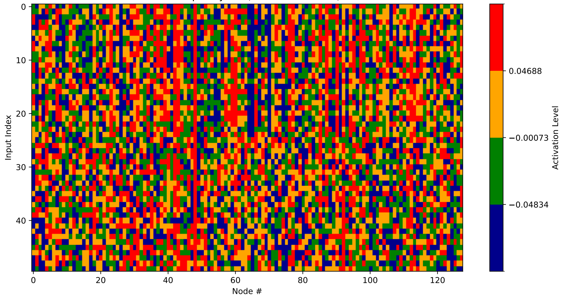
Heatmap - Layer 7 (Nodes 2304-2432)
