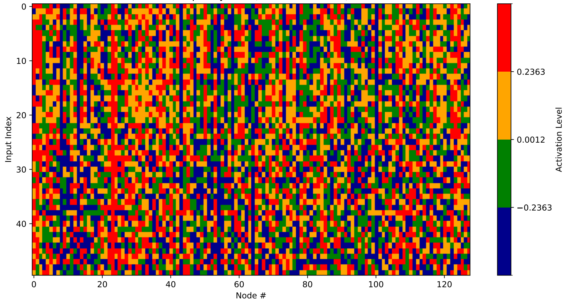
Heatmap - Layer 28 (Nodes 1792-1920)
