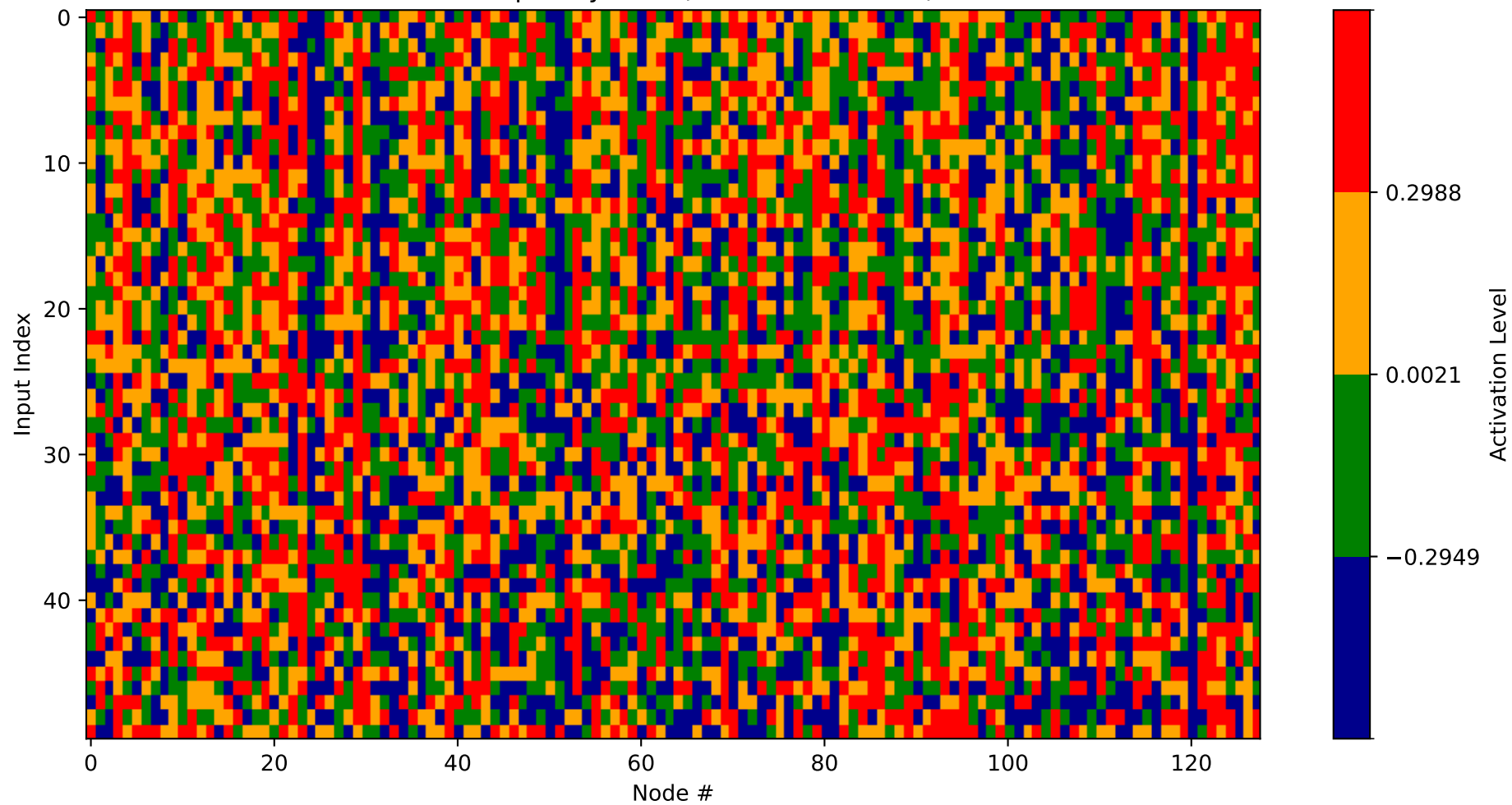
Heatmap - Layer 30 (Nodes 1536-1664)
