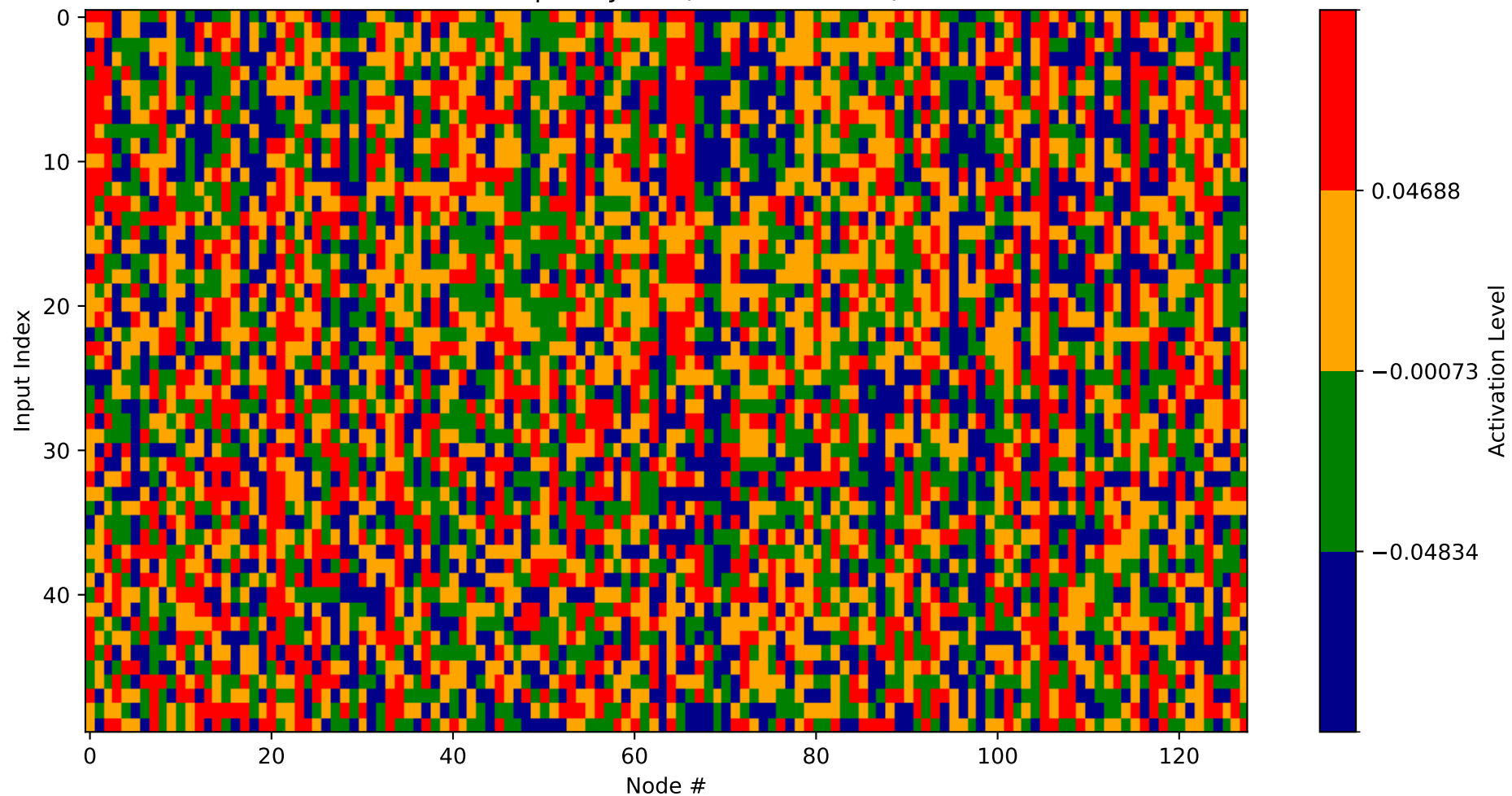
Heatmap - Layer 7 (Nodes 768-896)
