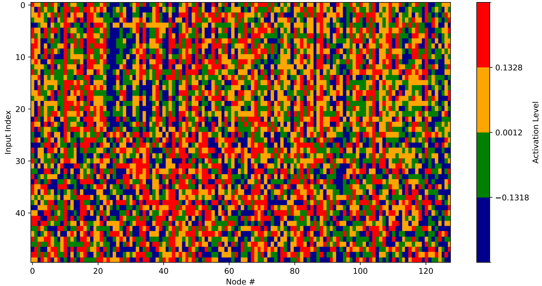
Heatmap - Layer 21 (Nodes 3328-3456)
