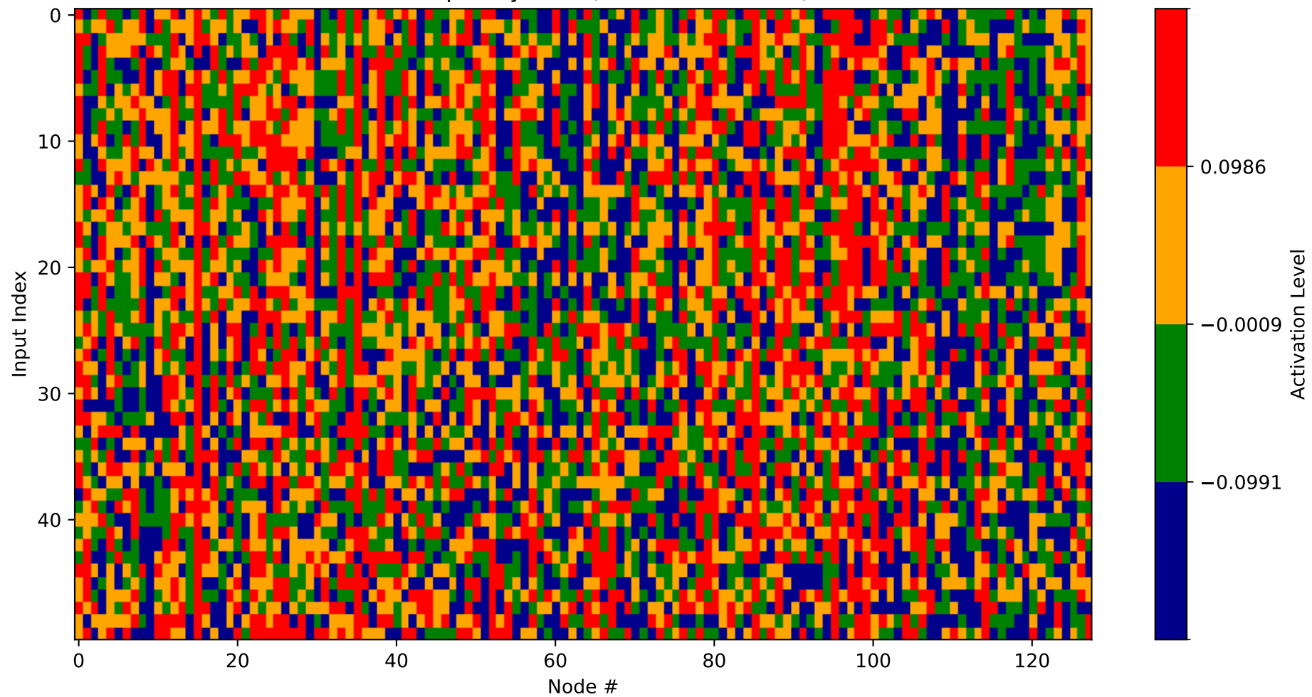
Heatmap - Layer 18 (Nodes 1024-1152)
