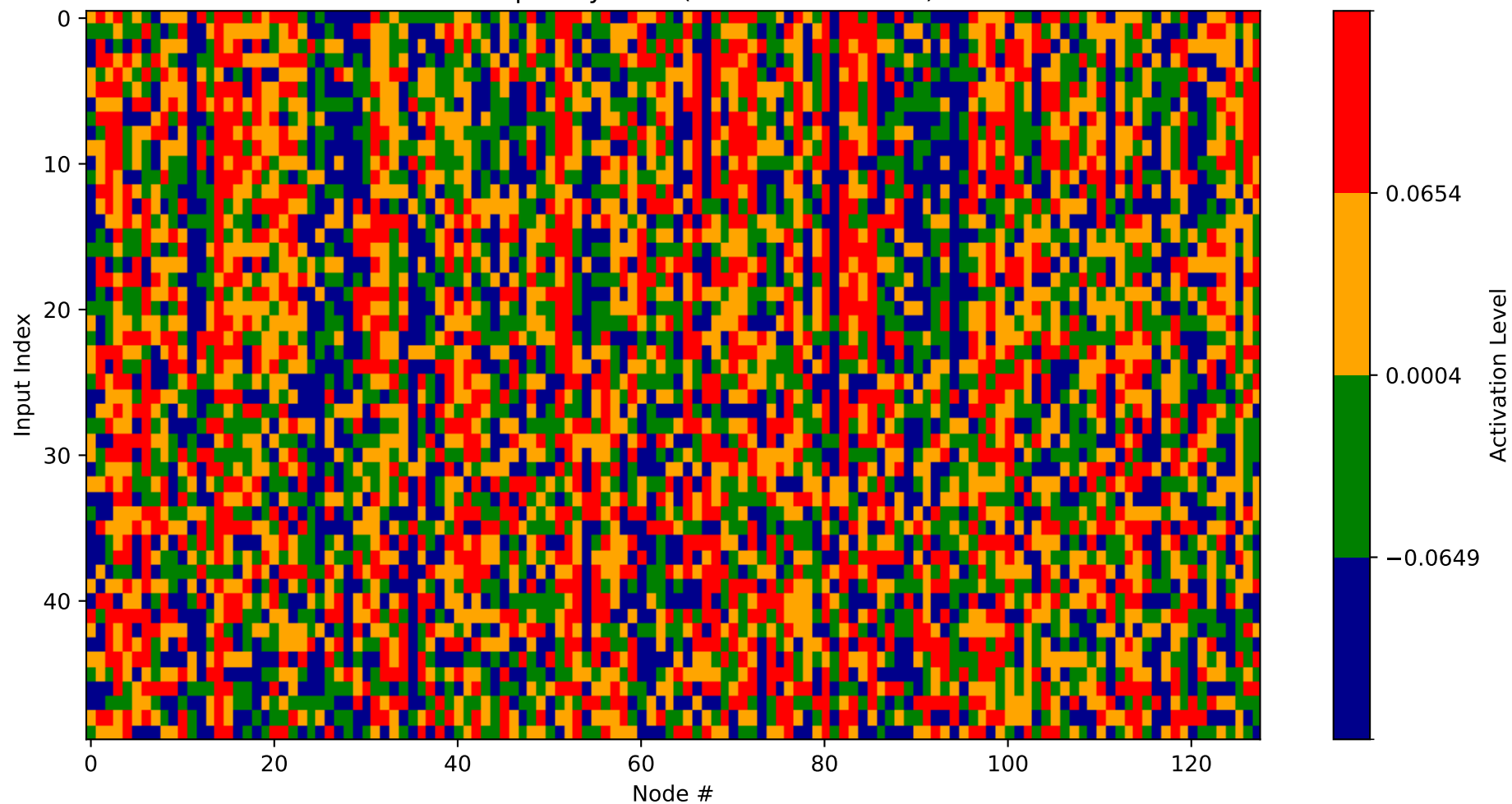
Heatmap - Layer 13 (Nodes 1920-2048)
