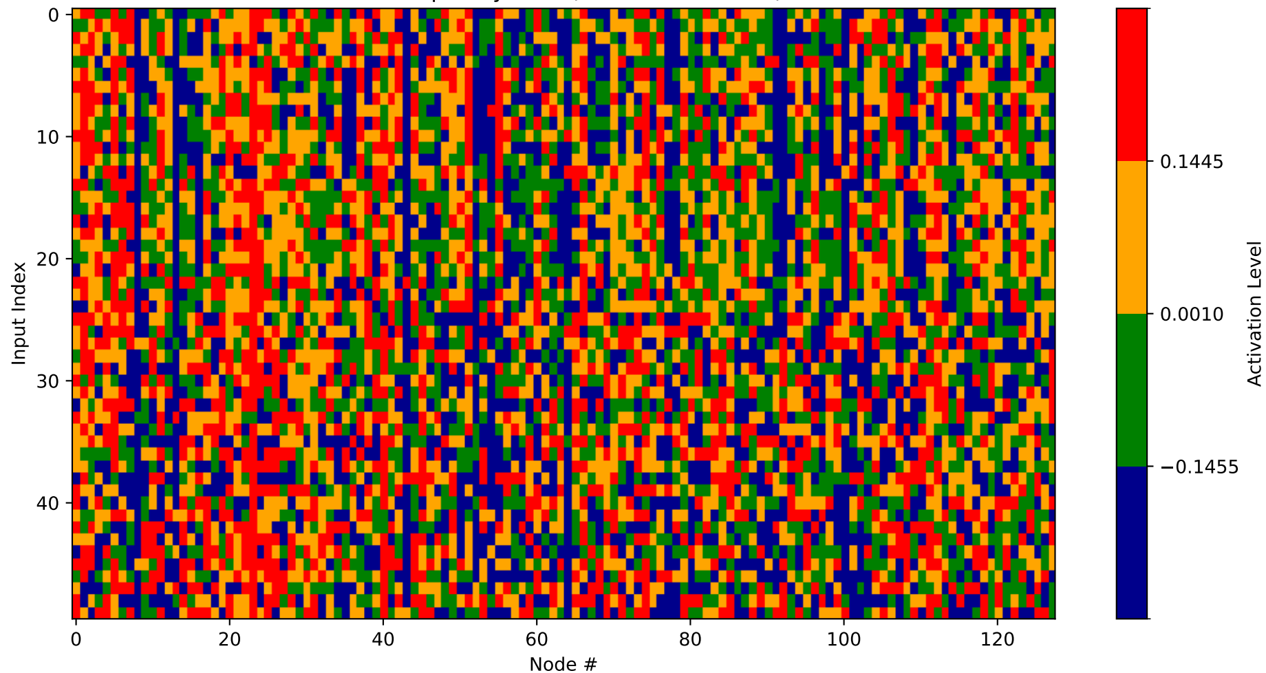
Heatmap - Layer 22 (Nodes 1792-1920)
