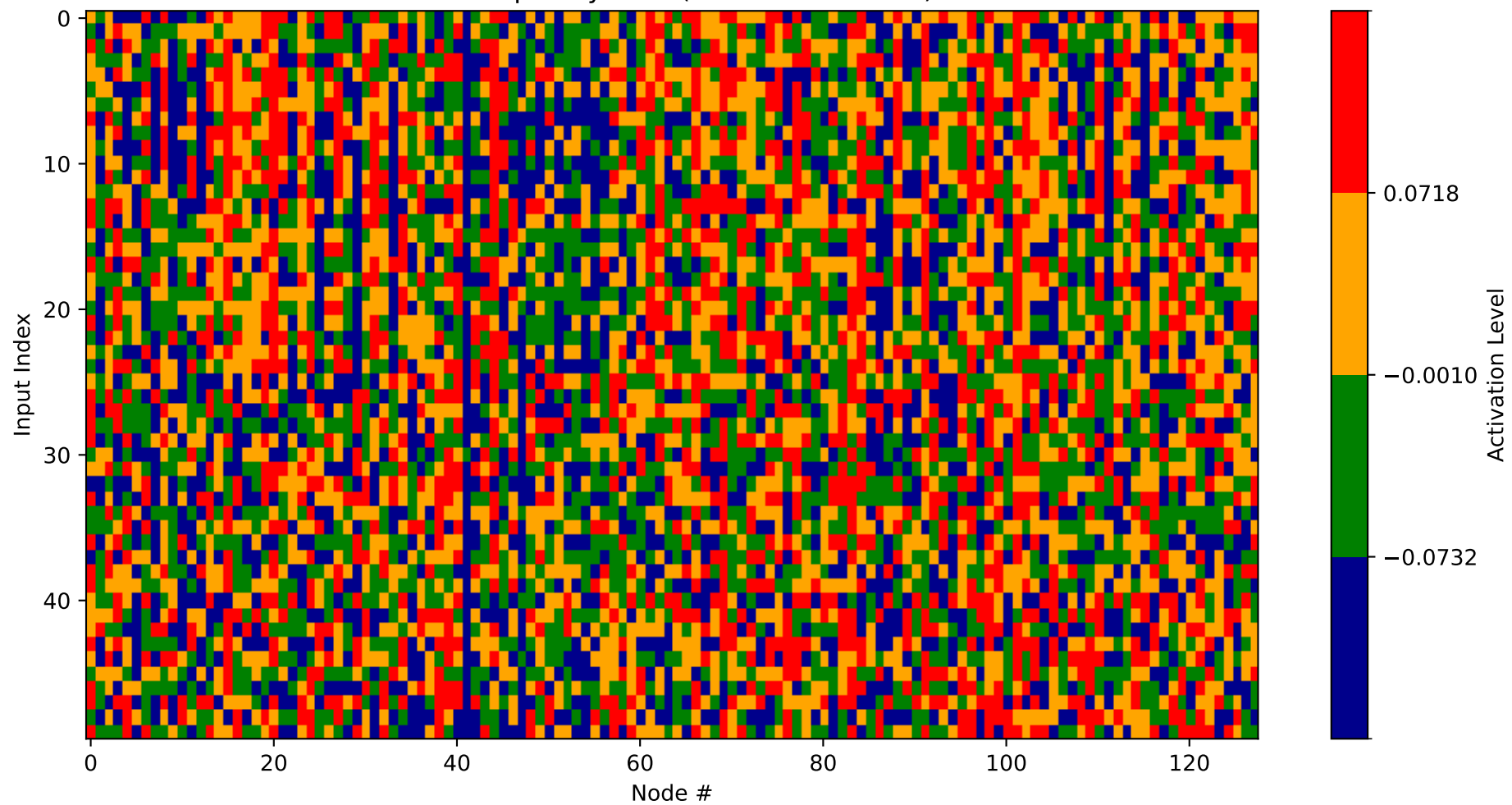
Heatmap - Layer 15 (Nodes 3840-3968)
