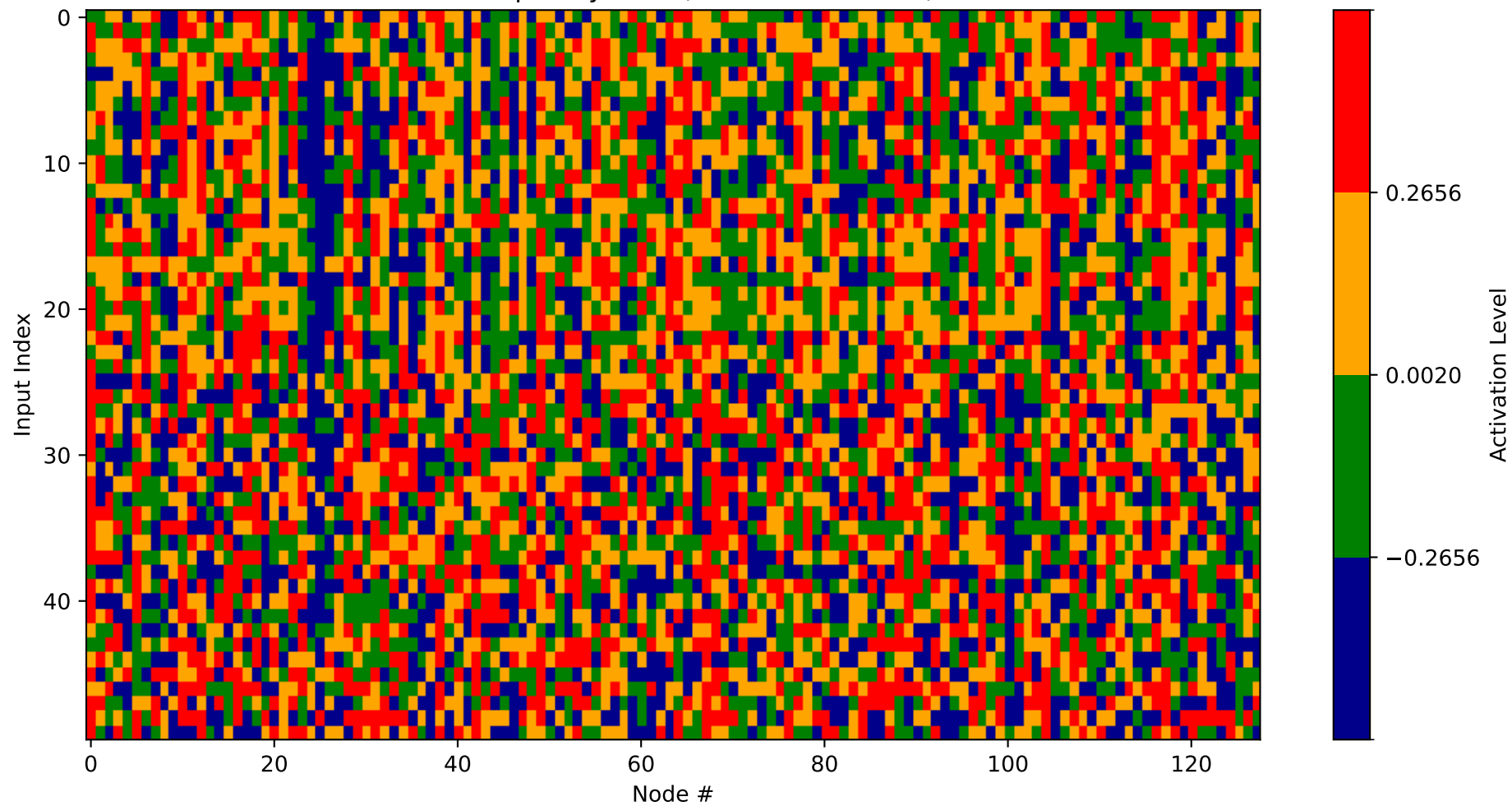
Heatmap - Layer 29 (Nodes 3328-3456)
