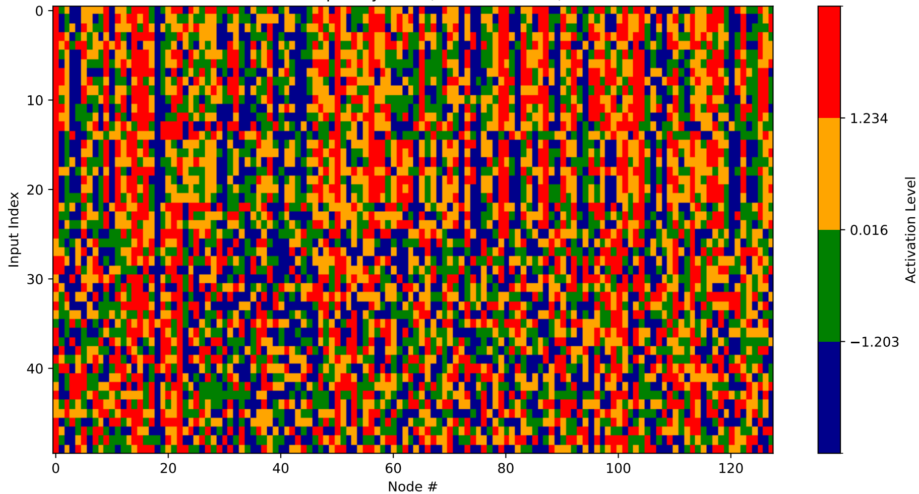
Heatmap - Layer 32 (Nodes 384-512)
