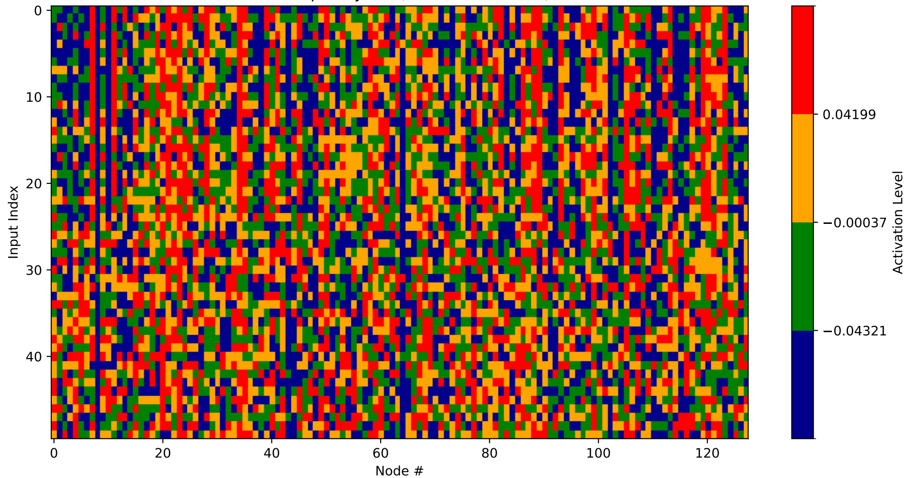
Heatmap - Layer 6 (Nodes 1792-1920)
