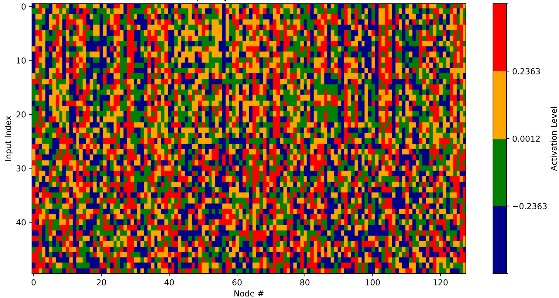
Heatmap - Layer 28 (Nodes 512-640)
