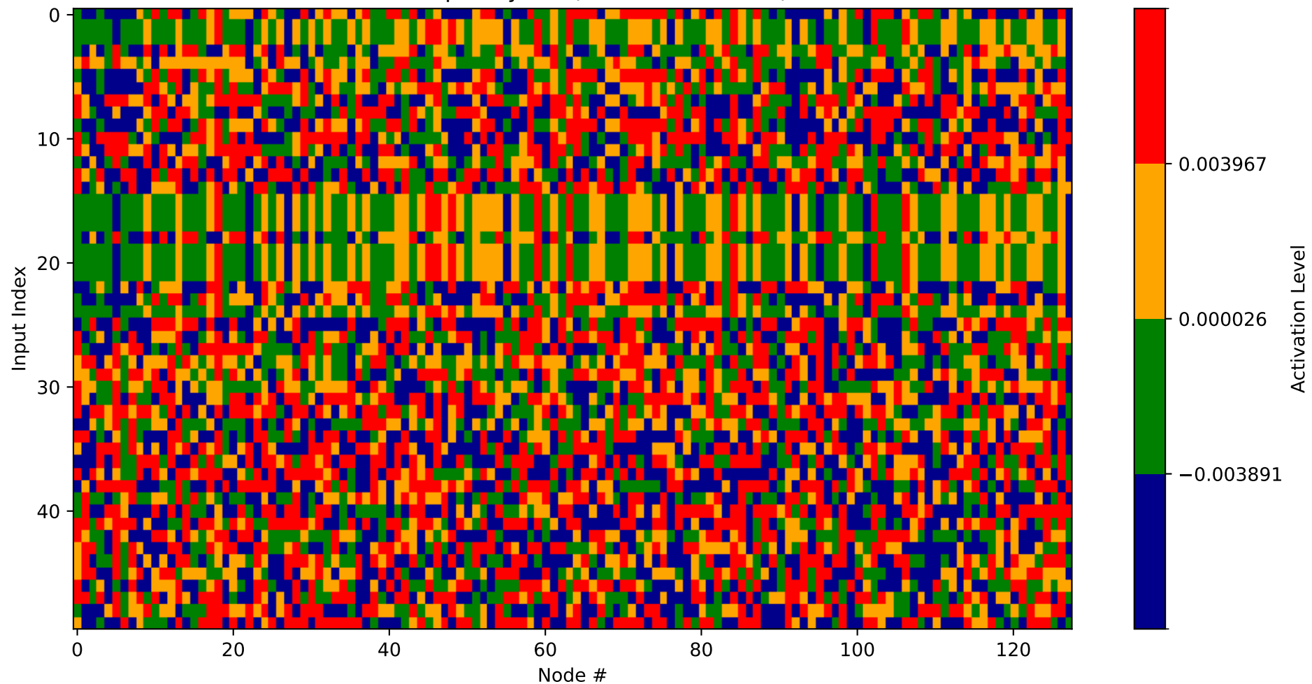
Heatmap - Layer 0 (Nodes 1664-1792)
