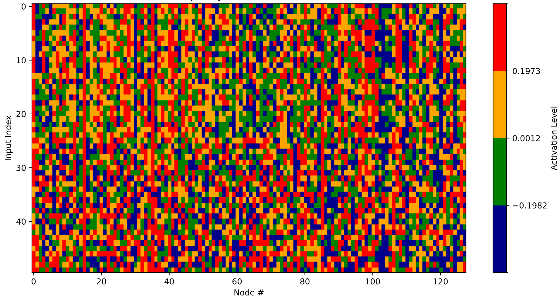
Heatmap - Layer 26 (Nodes 1024-1152)
