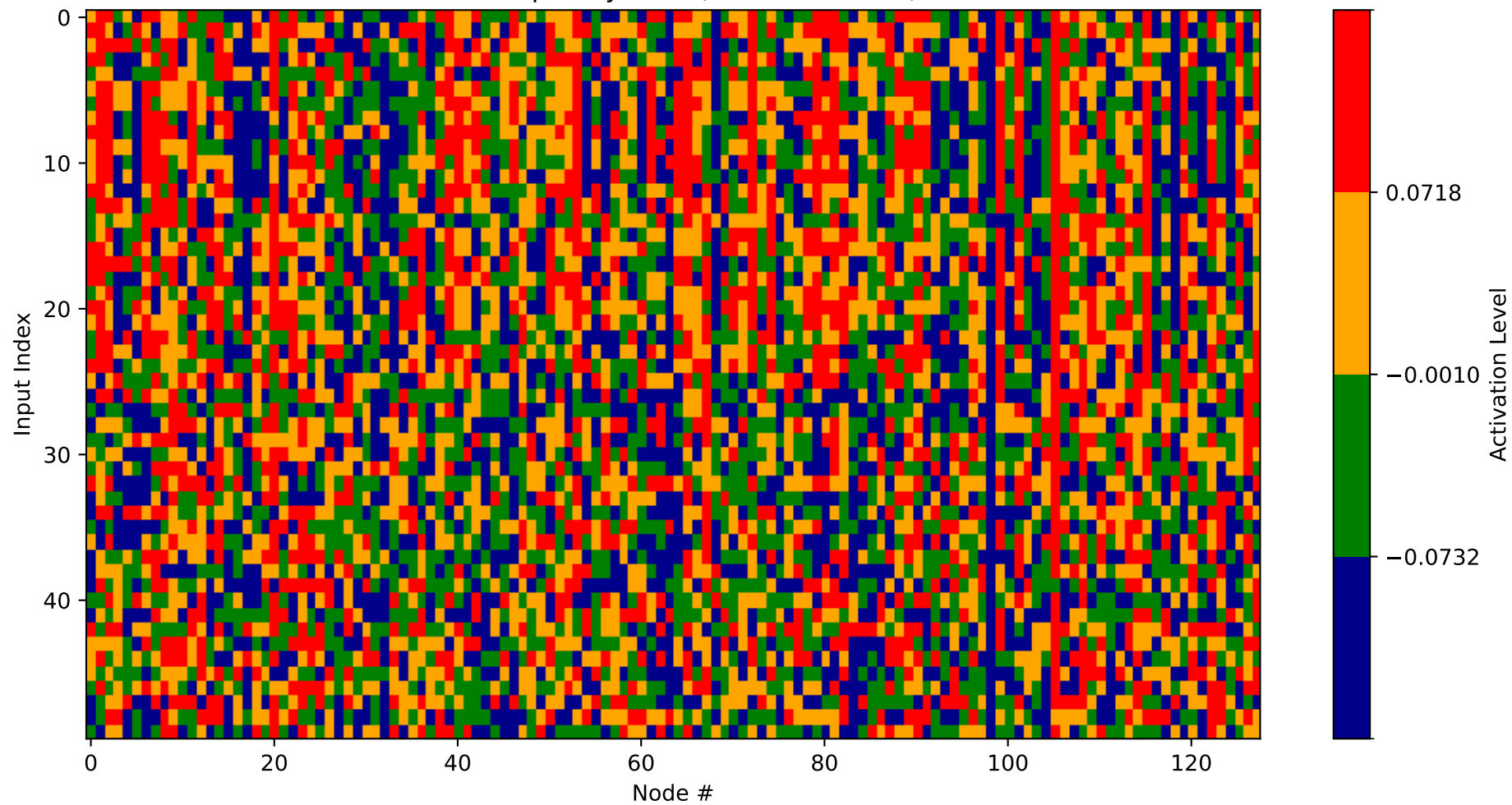
Heatmap - Layer 15 (Nodes 768-896)
