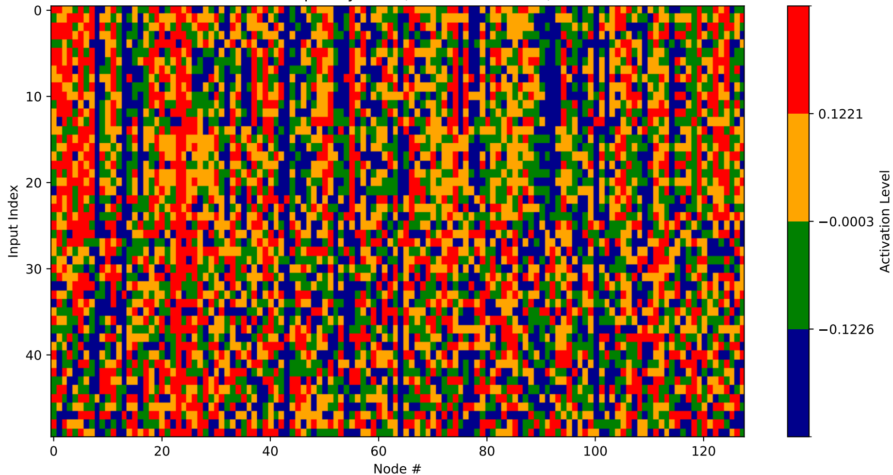
Heatmap - Layer 20 (Nodes 1792-1920)
