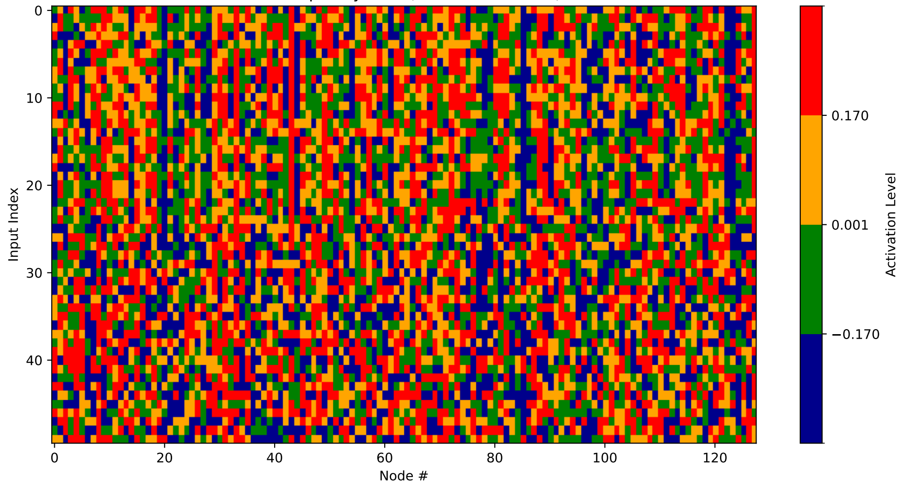
Heatmap - Layer 24 (Nodes 2176-2304)
