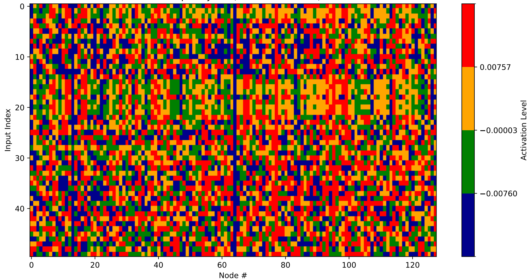
Heatmap - Layer 1 (Nodes 1408-1536)
