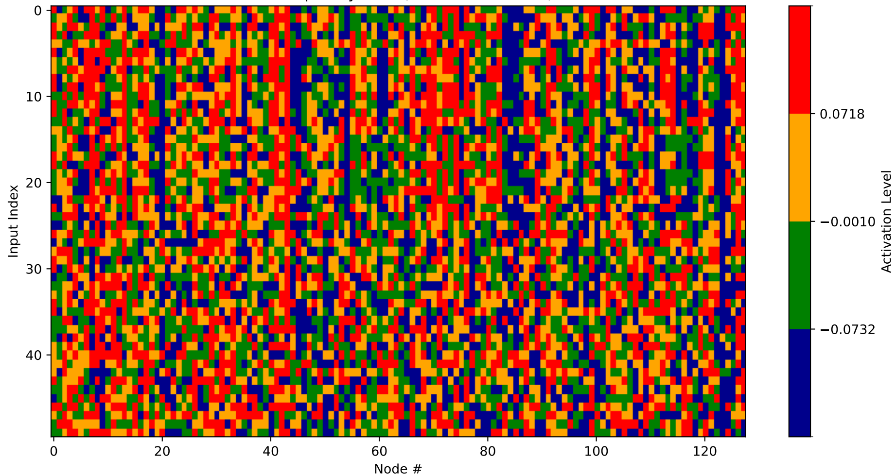
Heatmap - Layer 15 (Nodes 2176-2304)
