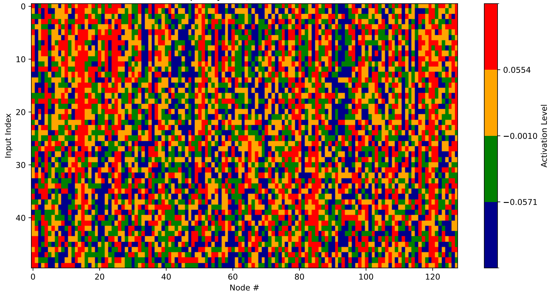
Heatmap - Layer 9 (Nodes 1024-1152)
