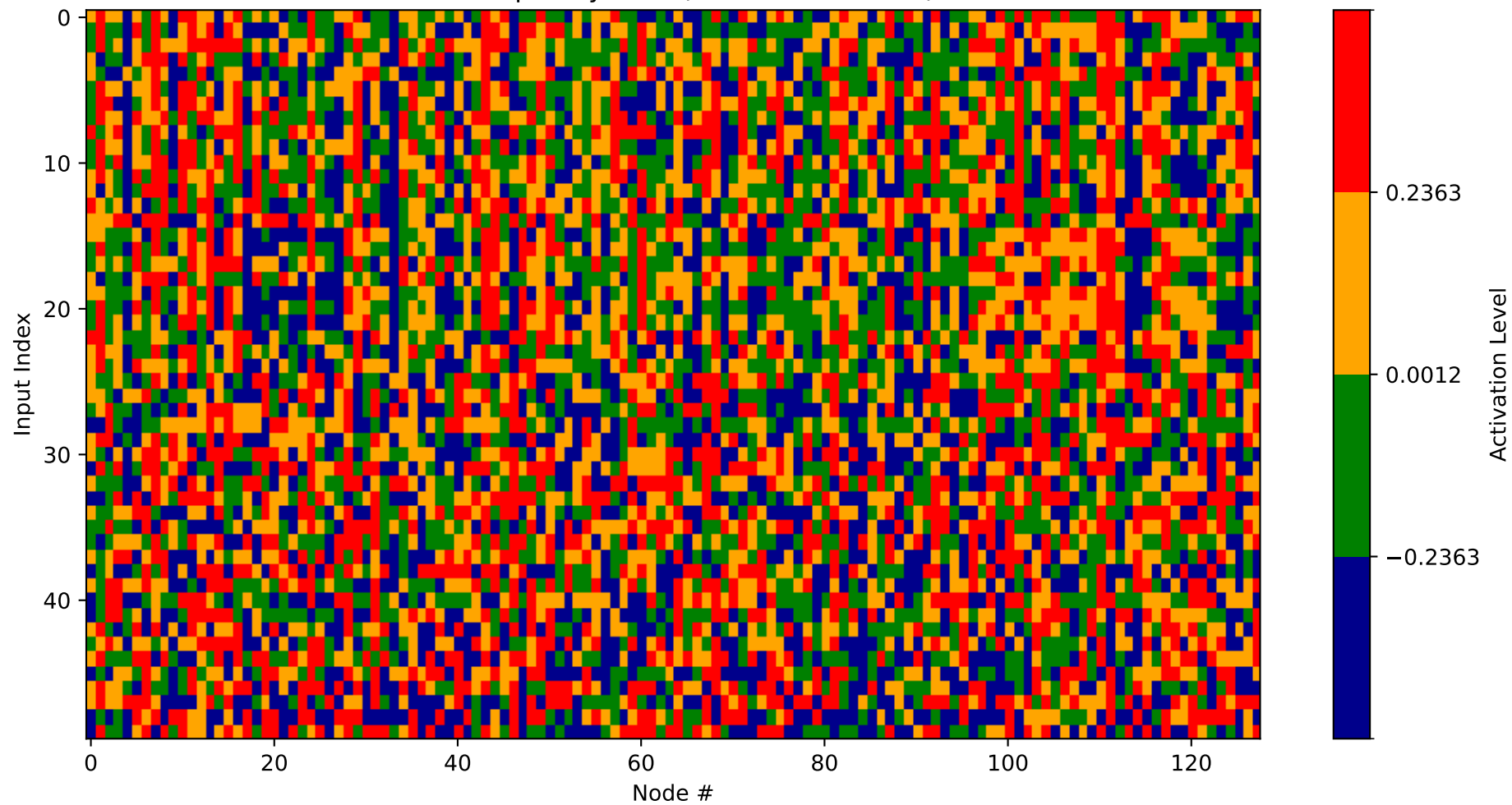
Heatmap - Layer 28 (Nodes 3072-3200)
