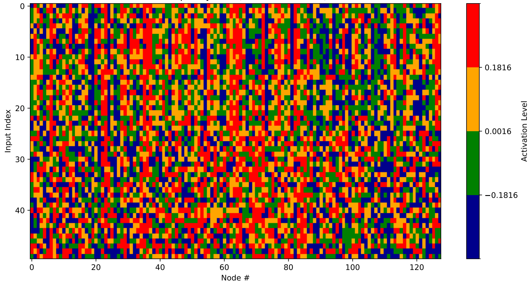
Heatmap - Layer 25 (Nodes 2816-2944)
