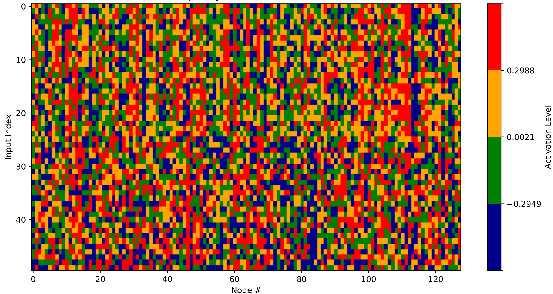
Heatmap - Layer 30 (Nodes 3072-3200)
