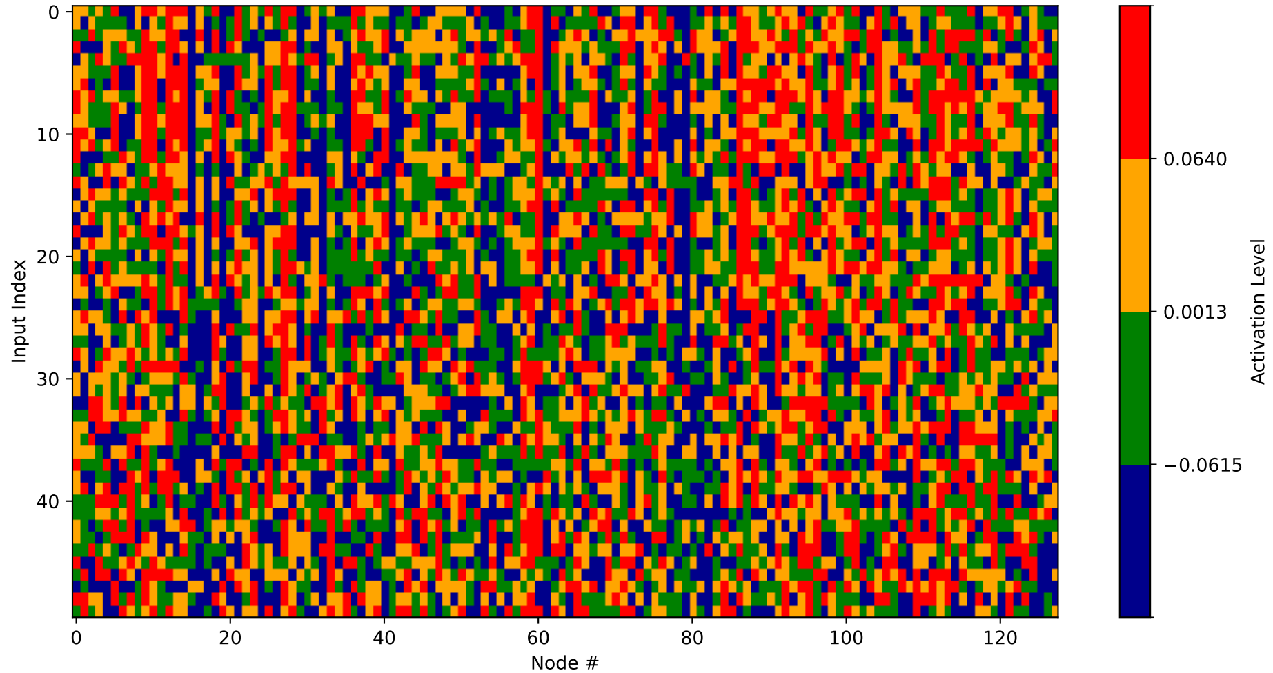
Heatmap - Layer 12 (Nodes 3456-3584)
