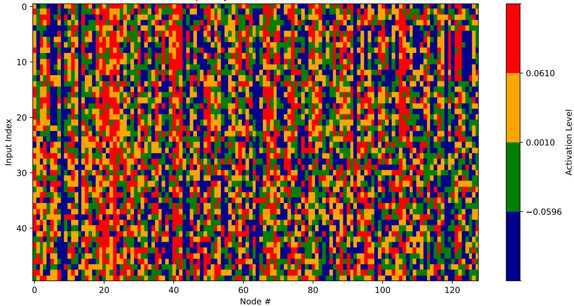
Heatmap - Layer 11 (Nodes 1792-1920)
