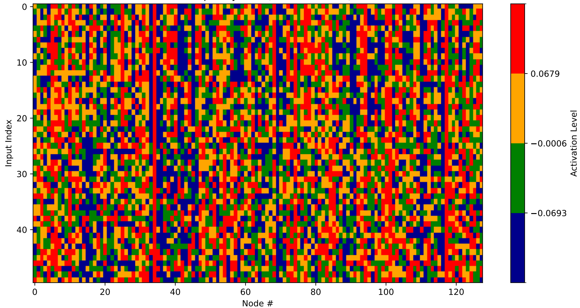
Heatmap - Layer 14 (Nodes 256-384)
