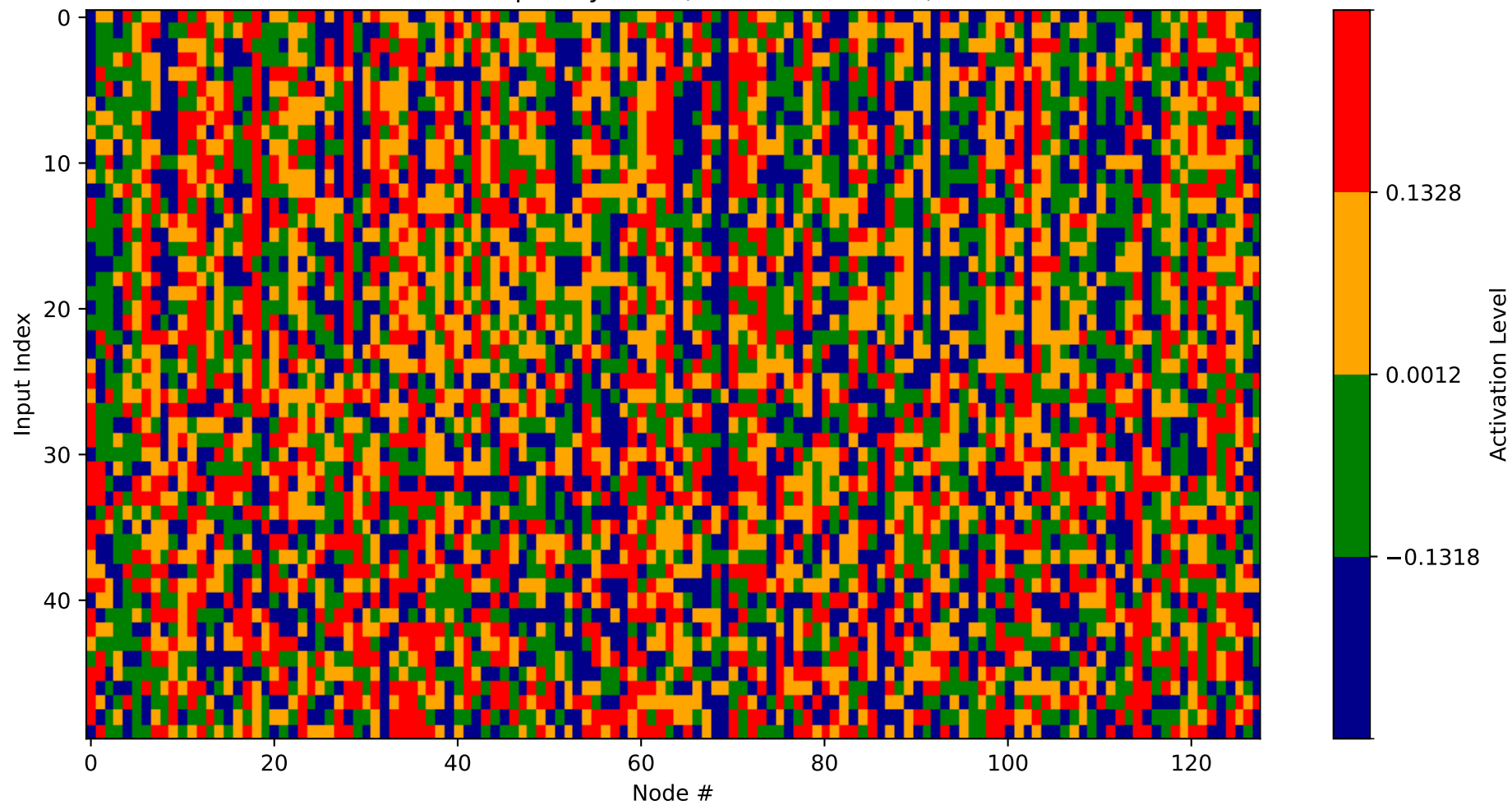
Heatmap - Layer 21 (Nodes 2560-2688)
