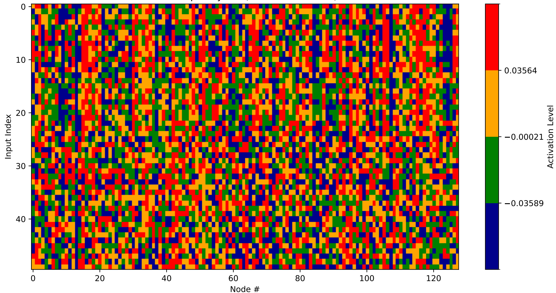
Heatmap - Layer 5 (Nodes 1408-1536)
