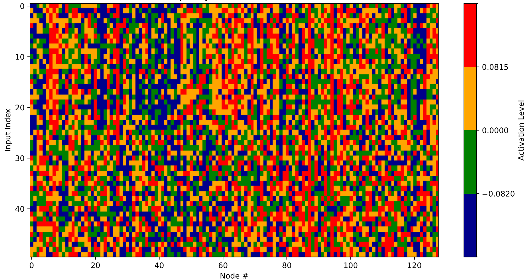
Heatmap - Layer 16 (Nodes 3968-4096)
