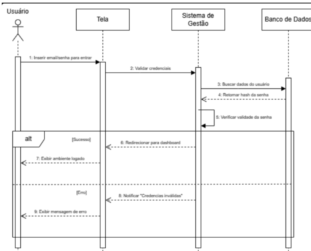
Imagem 10:Diagrama de Sequência 5 (Realizar Login)
