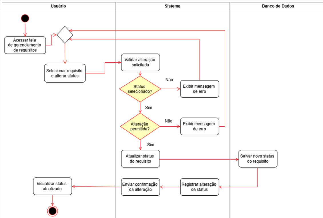
Imagem 12:Diagrama de Atividade 2 (Alterar Status Requisitos)
