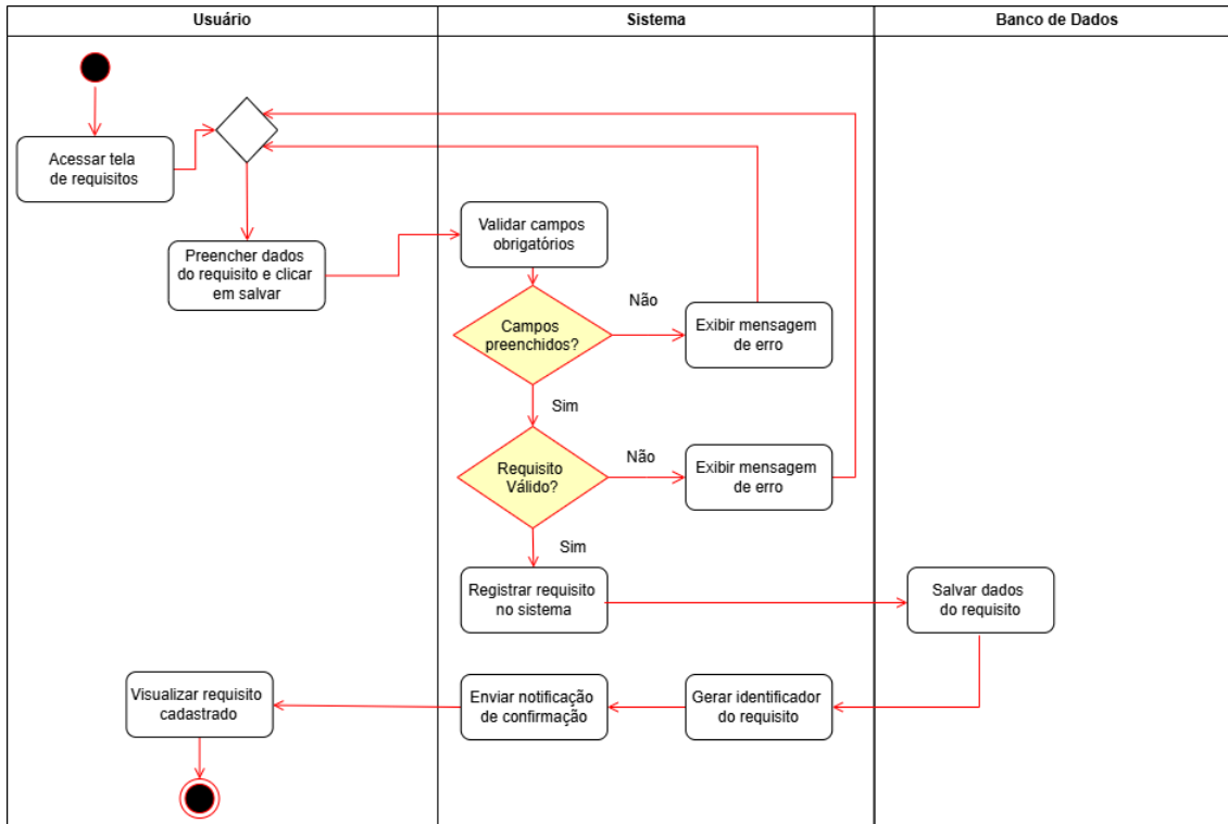
Imagem 11:Diagrama de Atividade 1 (Cadastrar Requisitos)
