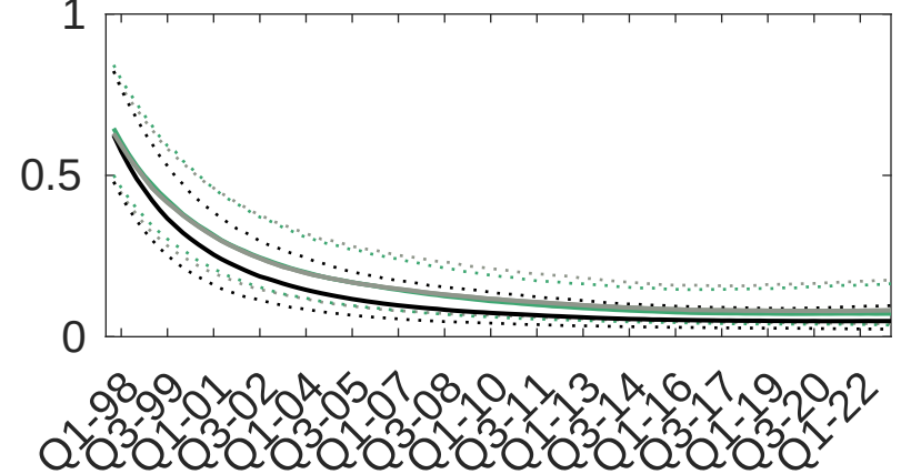
SV: Trend
