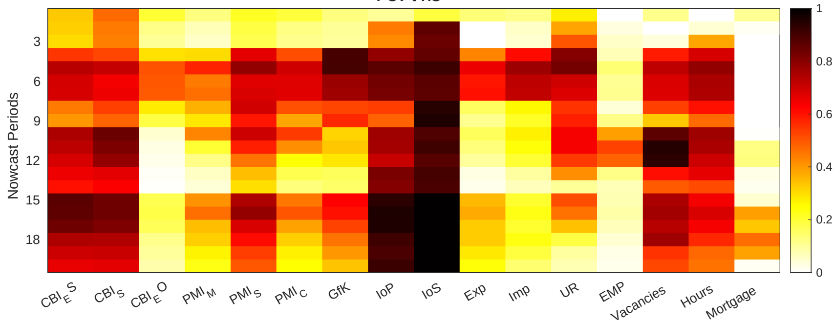
T-SV-t-HS
