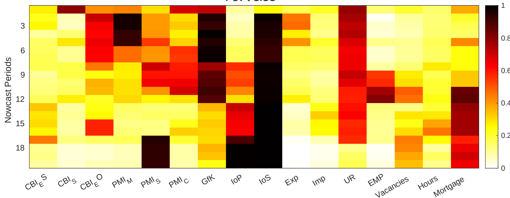
T-SV-t-GIGG
