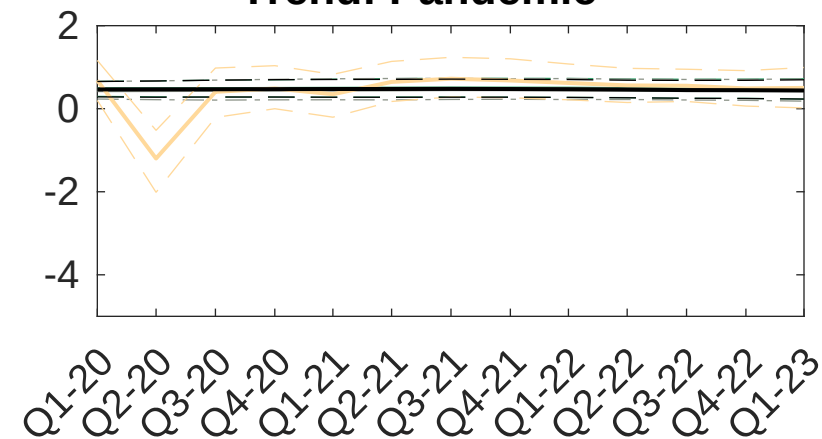
SV: Trend
