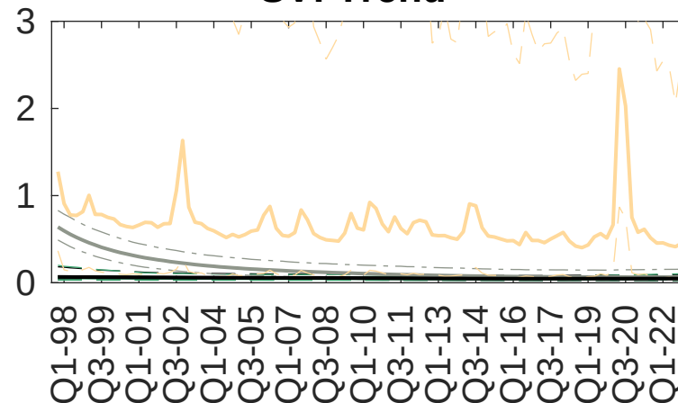
SV: Trend
