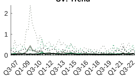
SV: Trend
