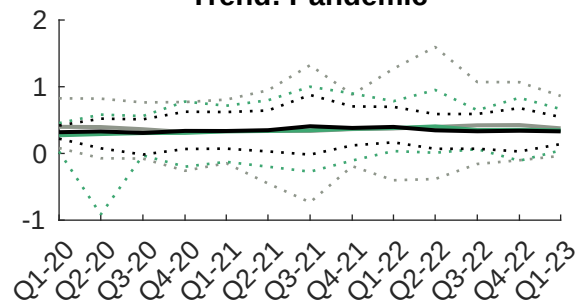
SV: Trend
