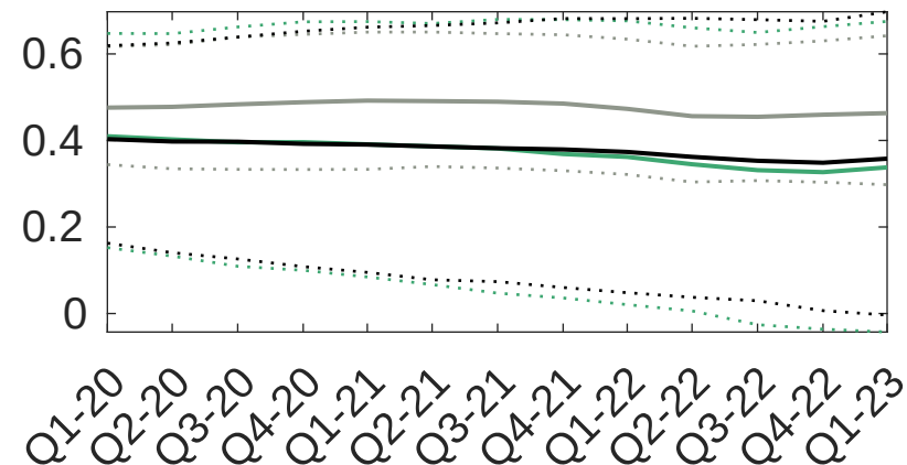
SV: Trend
