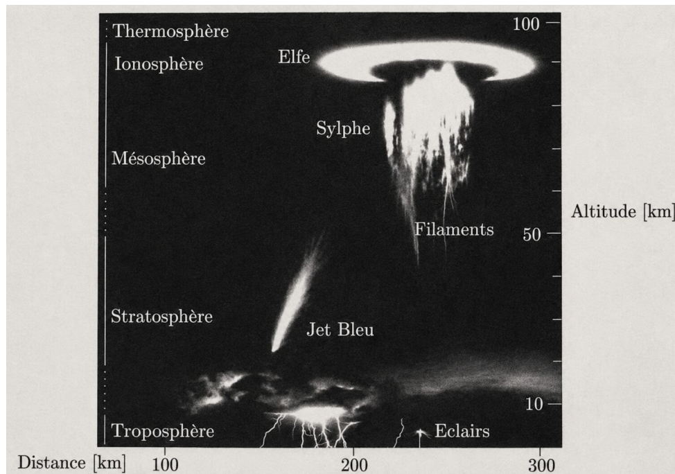
FIGURE 1 – Différentes formes de phénomènes lumineux éphémères atmosphériques.
