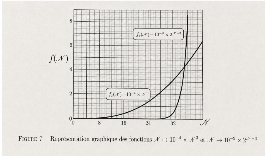
FIGURE 7 – Représentation graphique des fonctions \mathcal{N} \mapsto 10^{-4} \mathcal{N}^3 et \mathcal{N} \mapsto 10^{-9} 2^{\mathcal{N}-3} .
