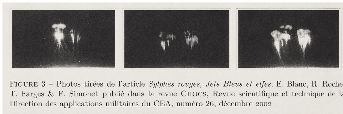
FIGURE 3 – Photos tirées de l'article Sylphes rouges, jets bleus et elfes , E. Blanc, R. Roche, T. Farges et F. Simonet, publié dans la revue CHOCS, revue scientifique et technique de la Direction des applications militaires du CEA, numéro 26, décembre 2002.
