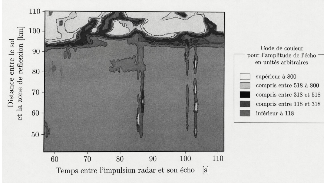
FIGURE 6 – Carte d'échos radar à 2,2 MHz depuis le sol pour l'événement enregistré à 13h39 le 15 octobre 1994 dans la station de Korhogo (Côte d'Ivoire). Figure tirée de l'article HF echoes from ionization potentially produced by high-altitude discharges , R. A. Roussel-Dupré et E. Blanc, Journal of Geophysical Research , vol. 102, n° A3, p. 4613–4622, 1997.
