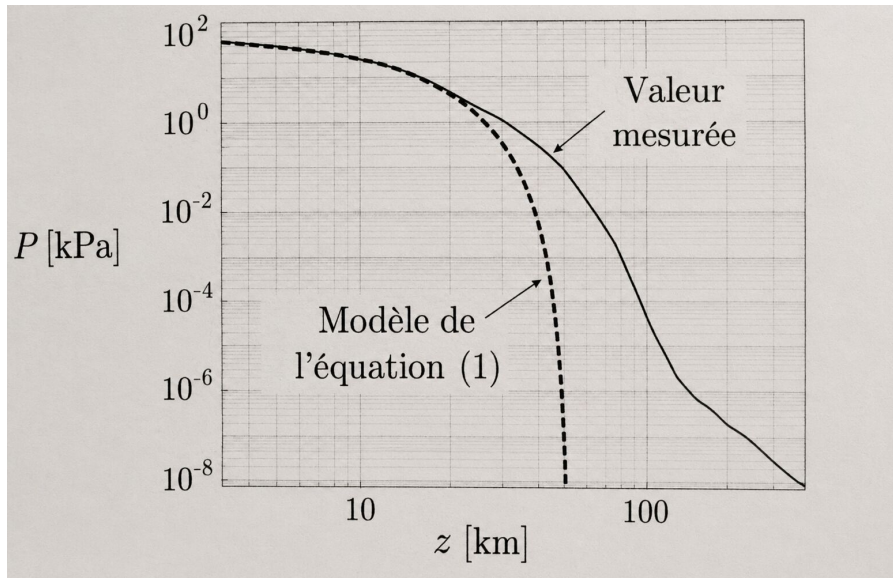
FIGURE 5 – Pression de l'air atmosphérique.
