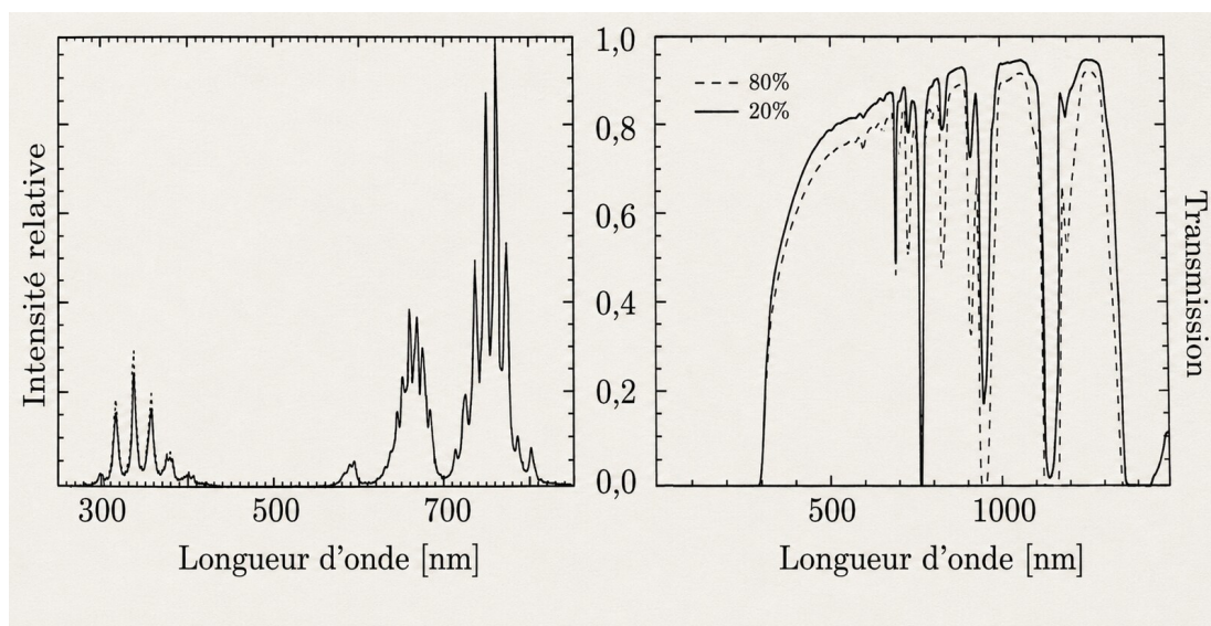
FIGURE 2 – À gauche : spectre d'émission d'un sylphe. À droite : coefficient de transmission de l'atmosphère avec deux taux d'humidité, 20 % et 80 %. Ces mesures ont été réalisées par un détecteur au sol placé sous une source située à 80 km d'altitude. Figure tirée de l'article Spectrum of Red Sprites , G. Milikh, J. A. Valdivia et K. Papadopoulos, Journal of Atmospheric and Solar-Terrestrial Physics , vol. 60, p. 907–915, 1998.
