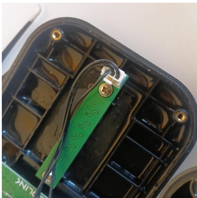
Fot. 1. Stan przy przyjęciu: krople wody i osady na dnie obudowy przy listwie LED.
