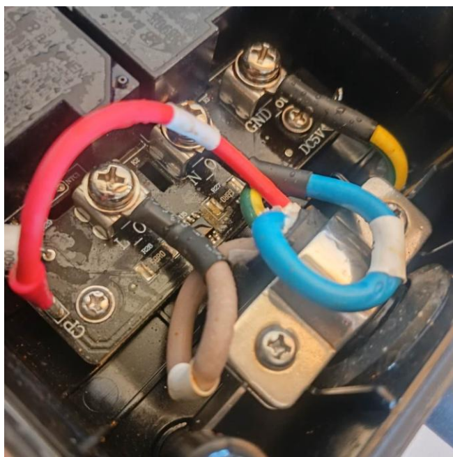
Fot. 2. Stan przy przyjęciu: ślady wody na zaciskach i przełączniku płyty głównej.
