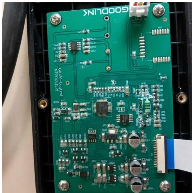
Fot. 4. Przed naprawą: płytka kontrolna zakwalifikowana do wymiany.
