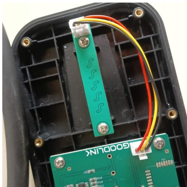
Fot. 5. Przed naprawą: listwa LED zakwalifikowana do wymiany.
