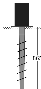
C. śruba ziemna \varnothing 76 \times 865 montaż bez betonu
