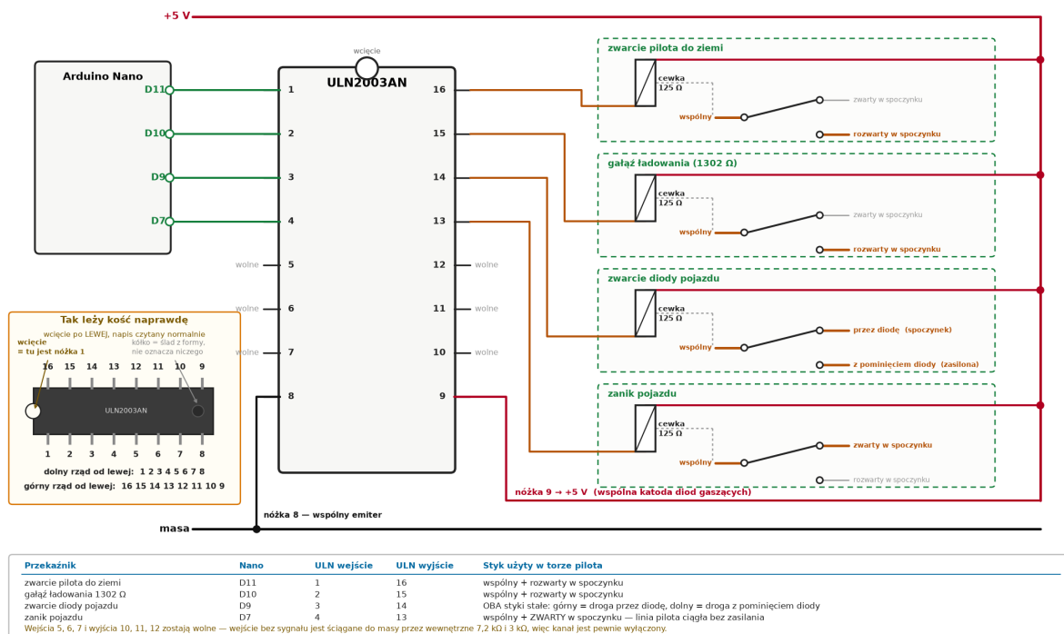
Rysunek 2: Schemat połączeń układu sterującego z procesorem i czterema przełącznikami, stan faktyczny. Wstawka w lewym dolnym rogu pokazuje rzeczywiste ułożenie kości: wcięcie po lewej, nóżka 1 na dole po lewej.
