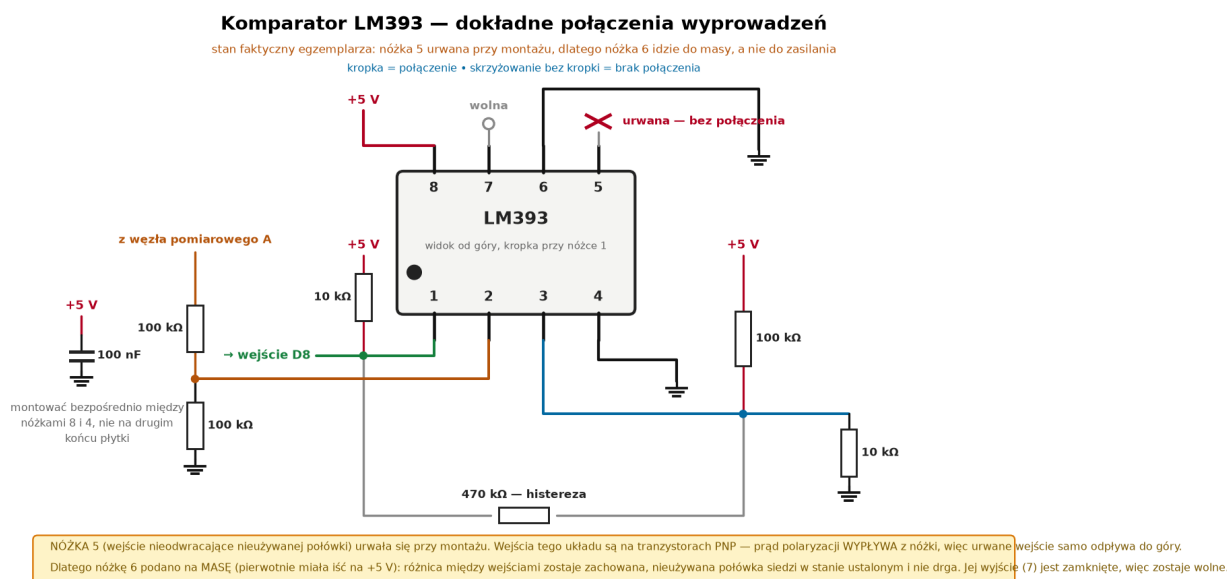
Rysunek 1: Dokładne połączenia wyprowadzeń komparatora, stan faktyczny egzemplarza.
