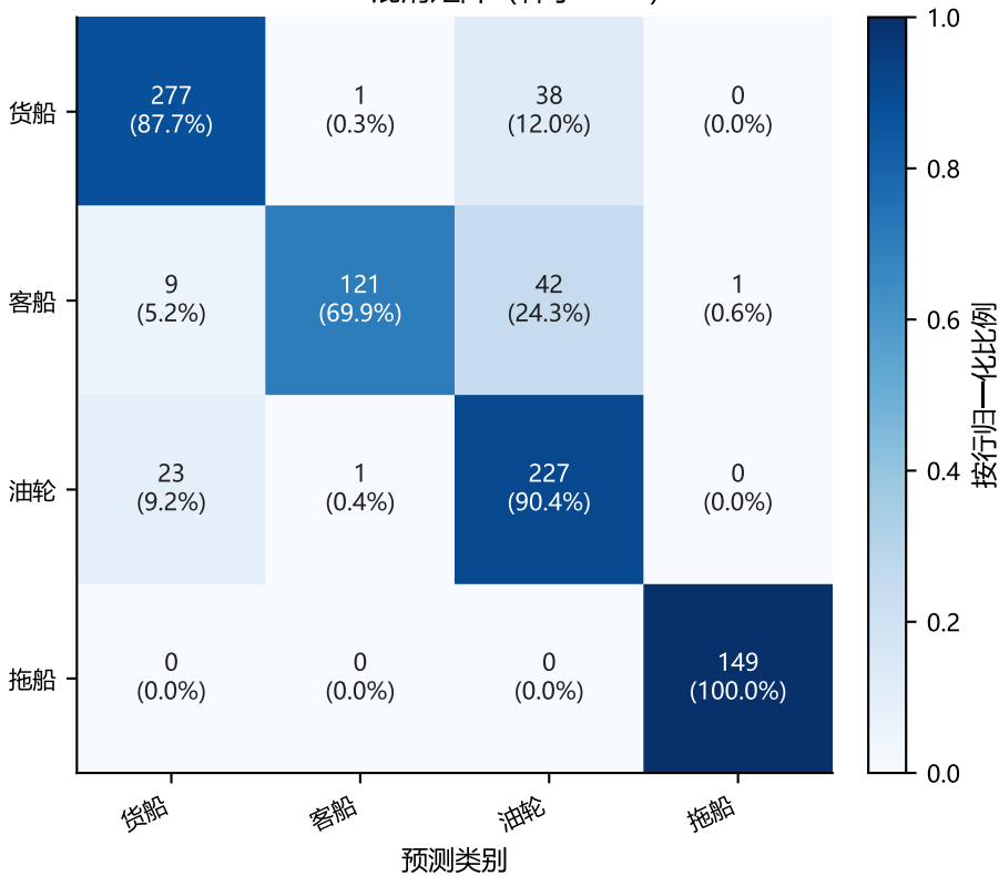
PVSC-Net混淆矩阵 (种子2026)
