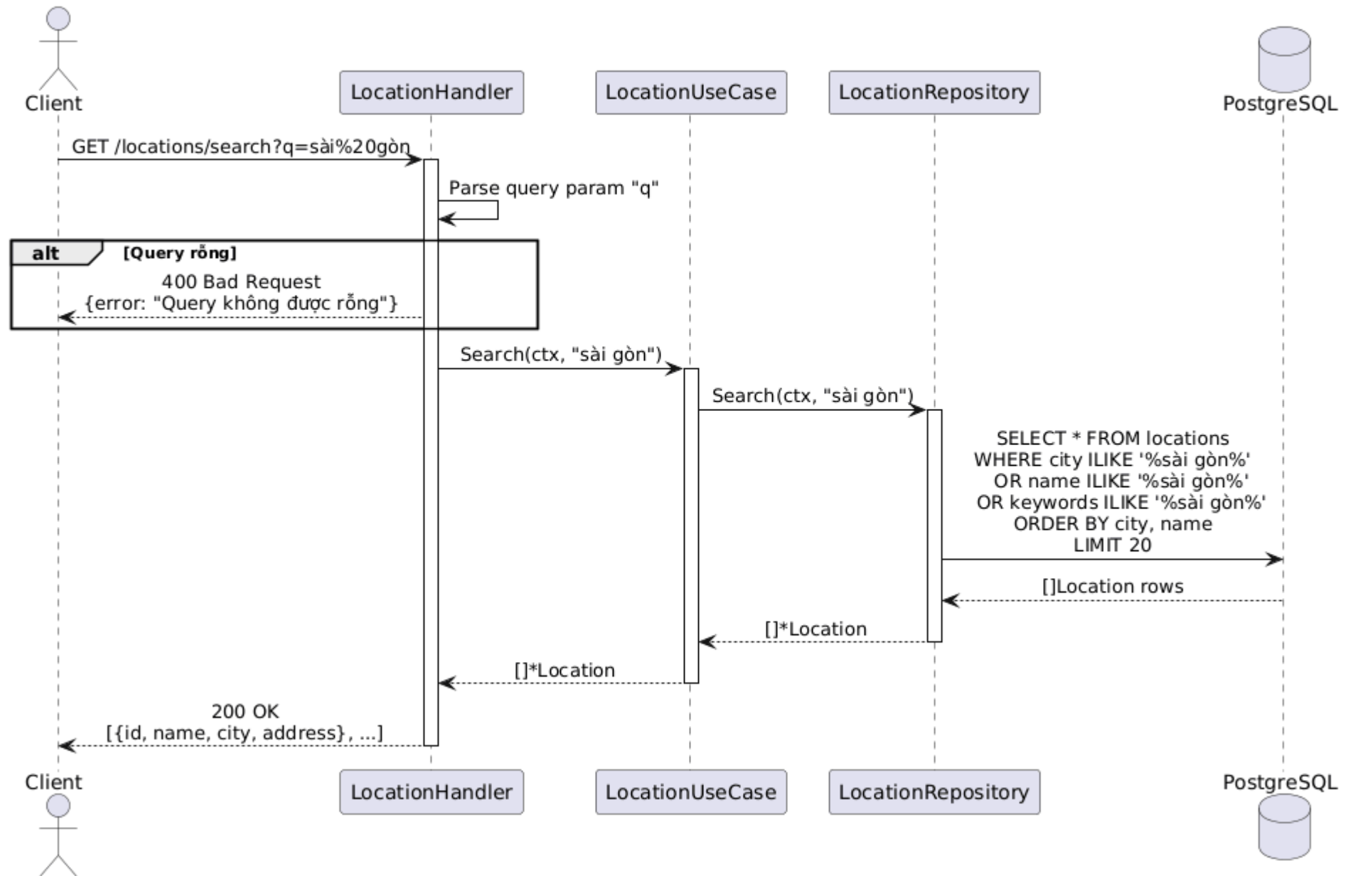
Sequence Diagram: Tìm kiếm Địa điểm
