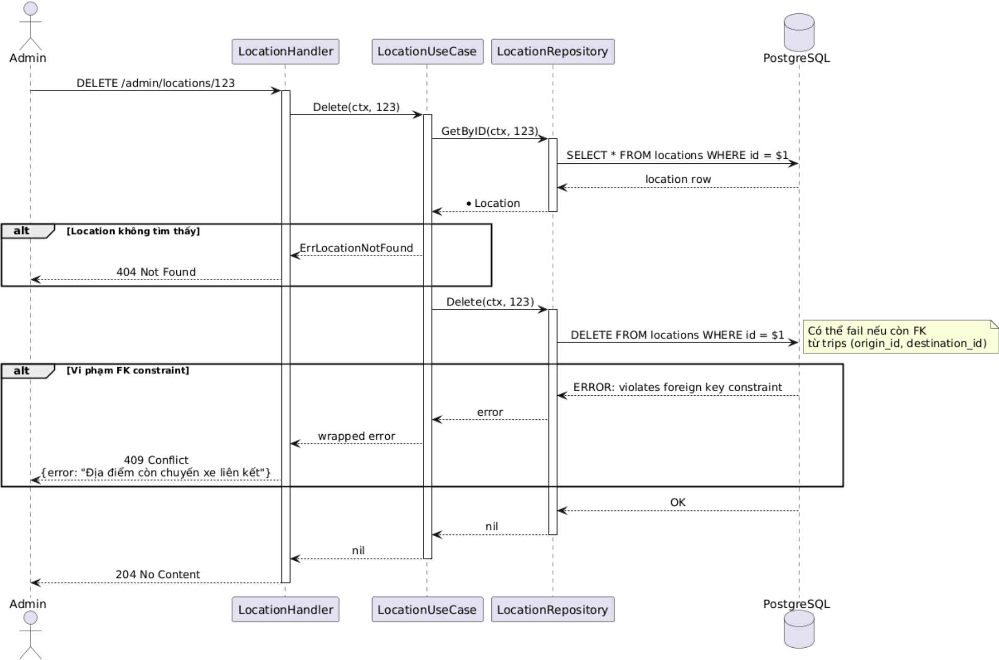
Sequence Diagram: Xóa Địa điểm
