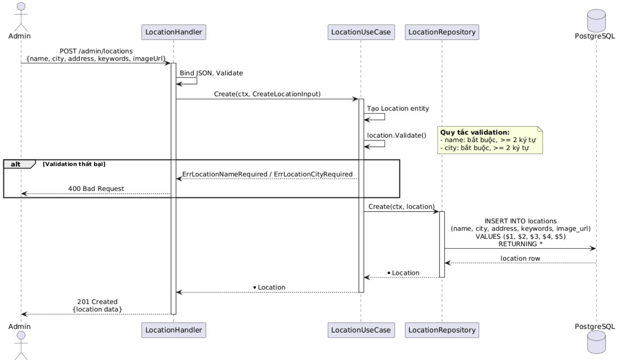
Sequence Diagram: Tạo Địa điểm Mới
