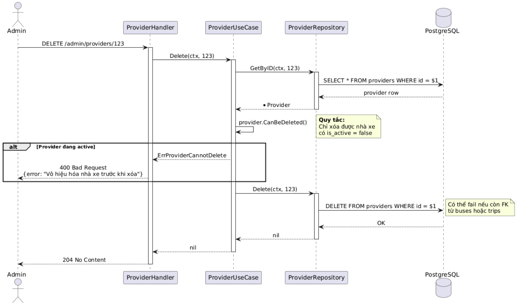
Sequence Diagram: Xóa Nhà xe
