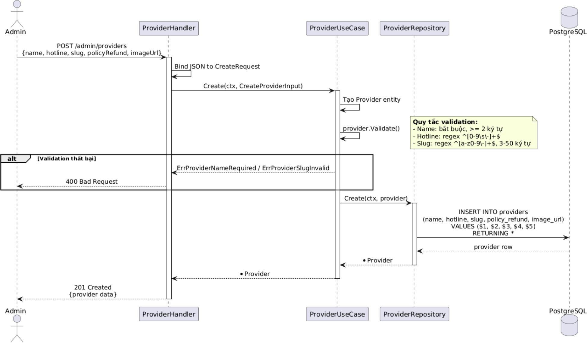
Sequence Diagram: Tạo Nhà xe Mới
