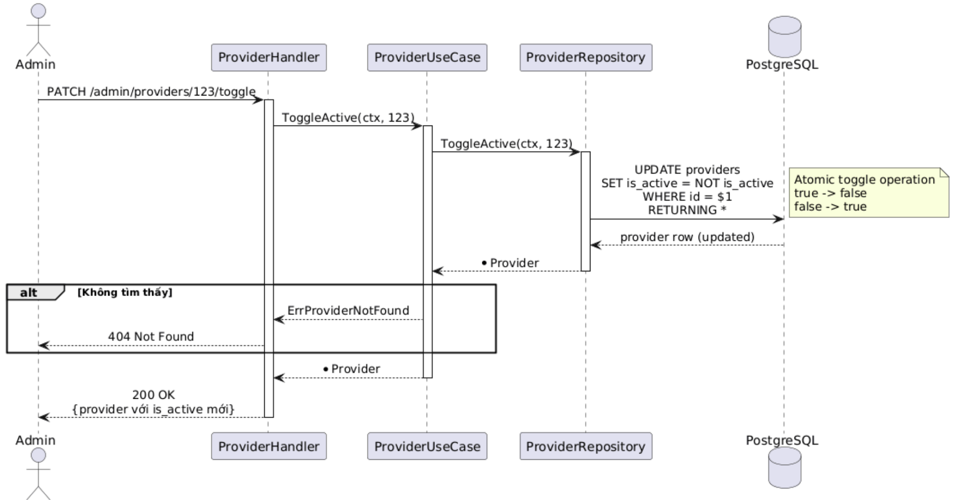
Sequence Diagram: Bật/Tắt Trạng thái Hoạt động
