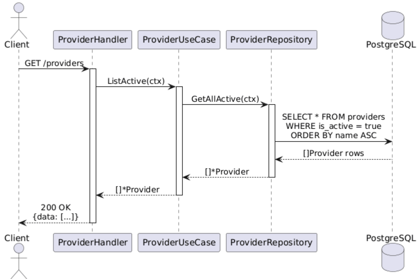
Sequence Diagram: Danh sách Nhà xe Hoạt động (Public)
