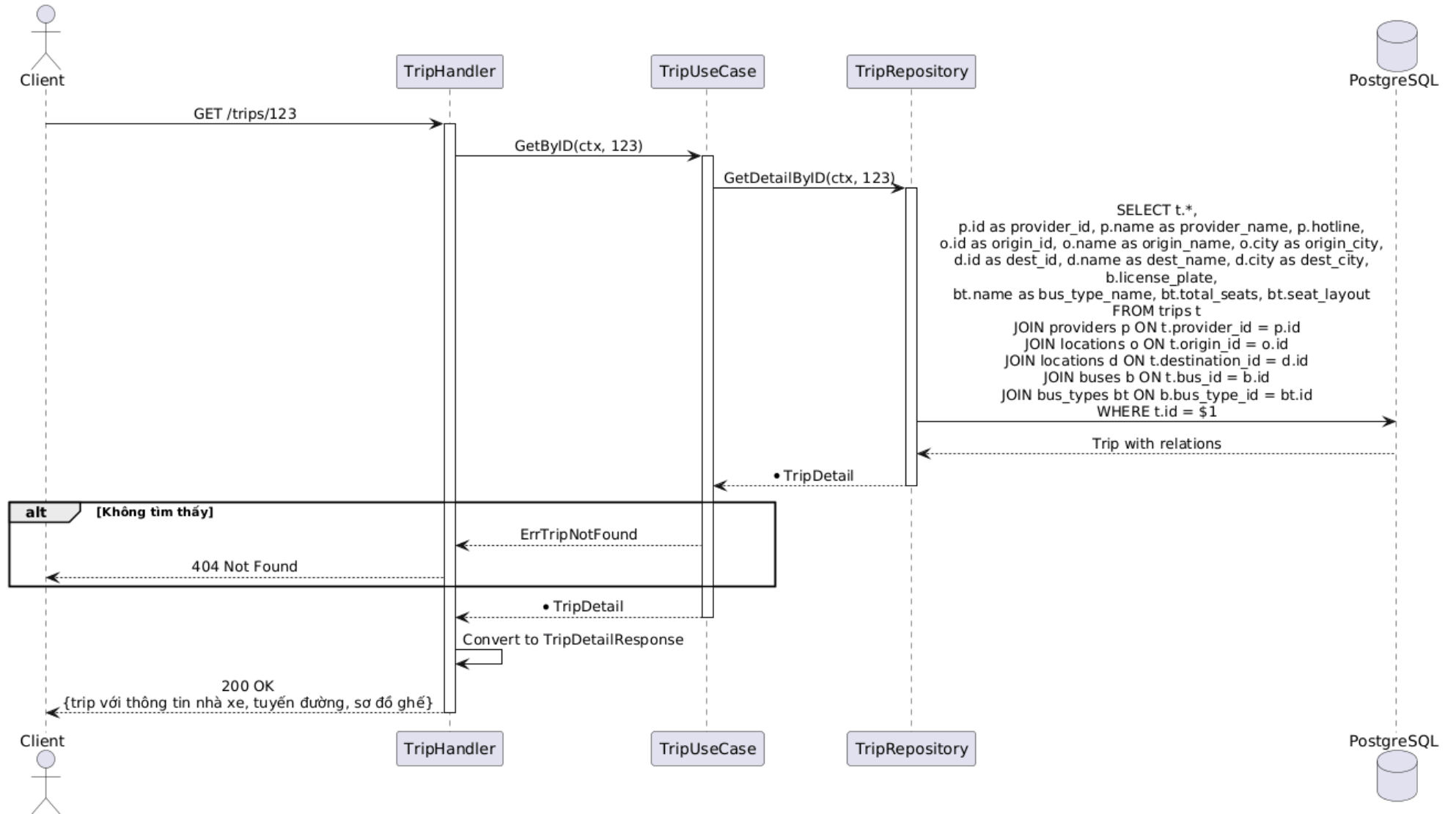
Sequence Diagram: Xem Chi tiết Chuyến xe
