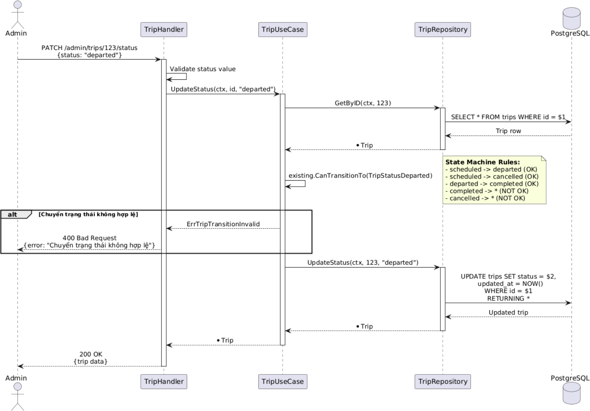
Sequence Diagram: Cập nhật Trạng thái Chuyến xe
