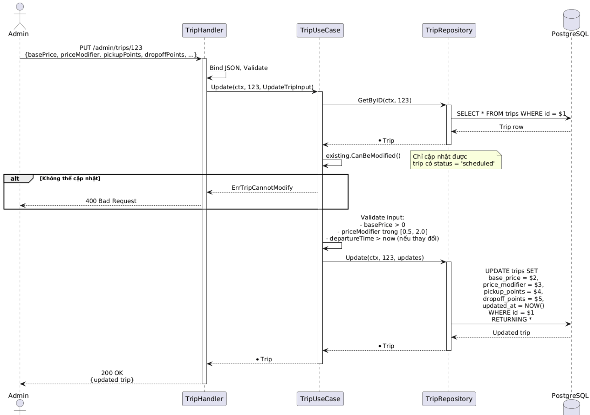
Sequence Diagram: Cập nhật Thông tin Chuyến xe
