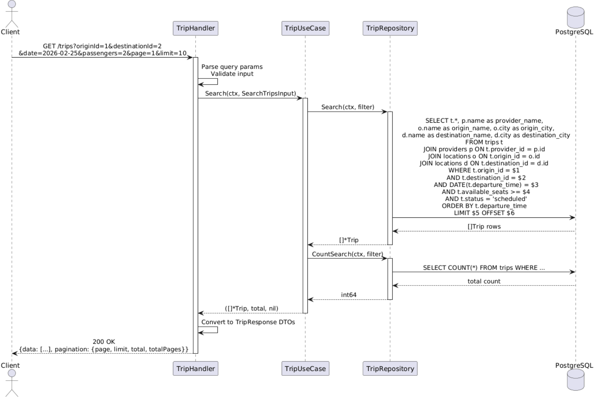
Sequence Diagram: Tìm kiếm Chuyến xe
