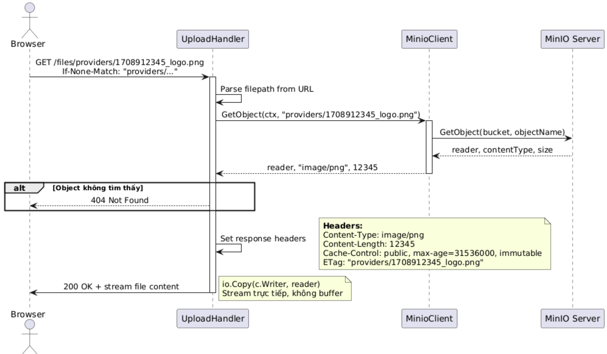
Sequence Diagram: Phục Vụ File
