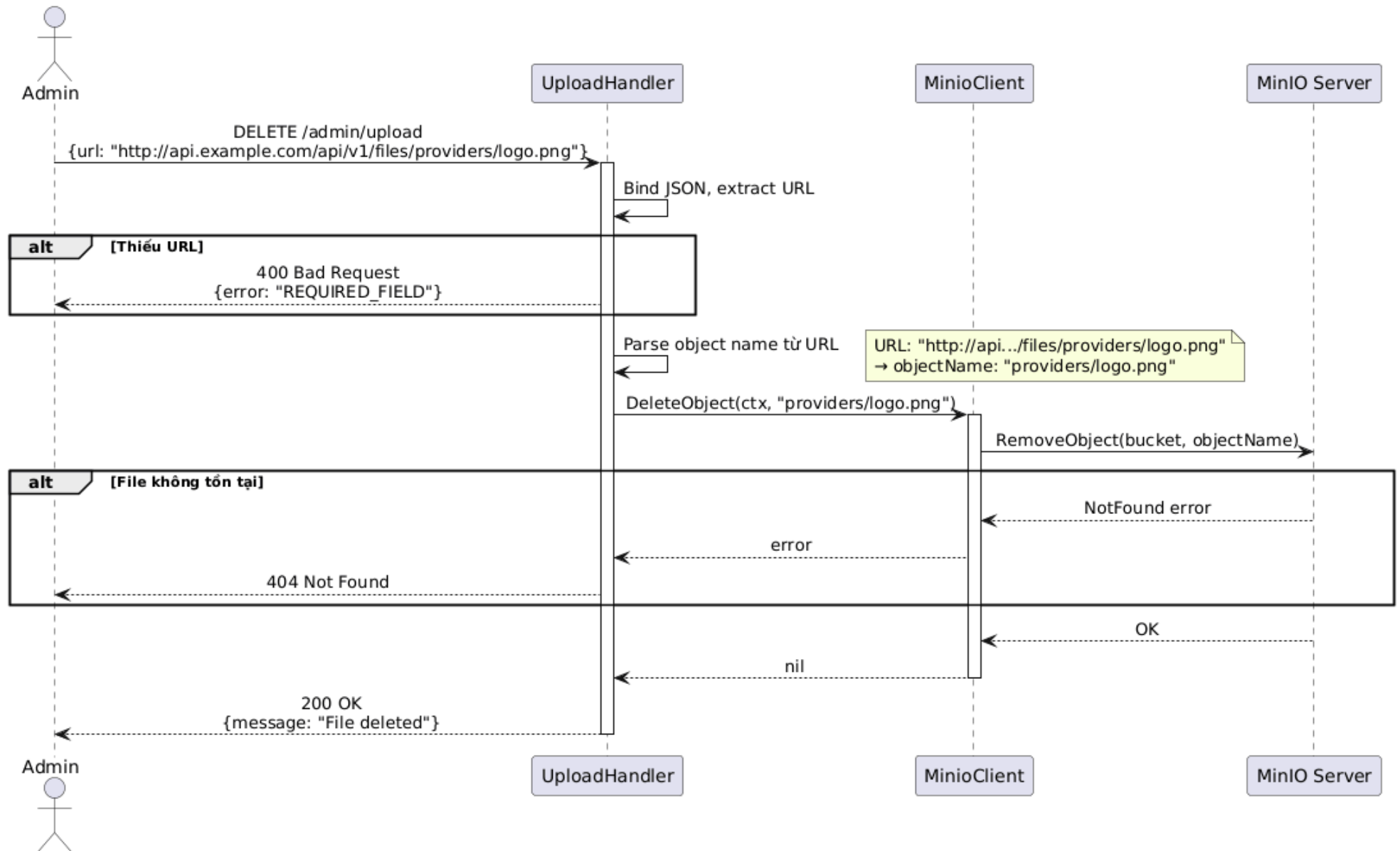
Sequence Diagram: Xóa Hình Ảnh
