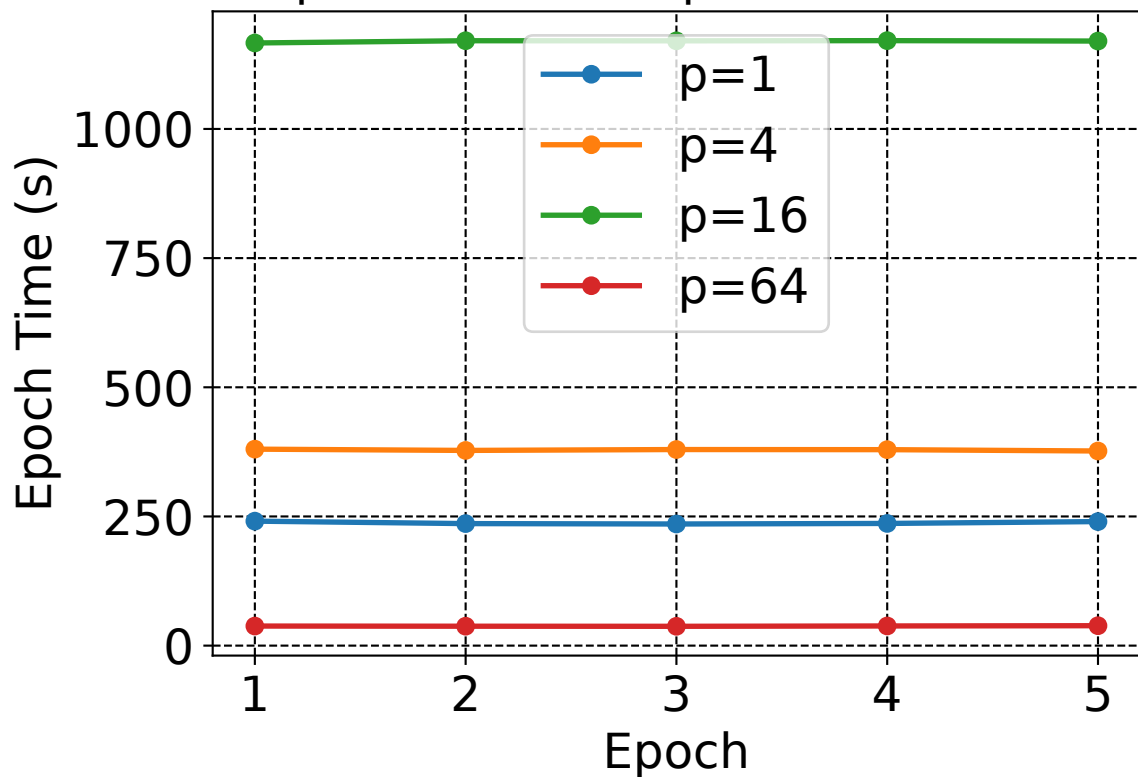
Epoch Time Per Epoch for h=4096
