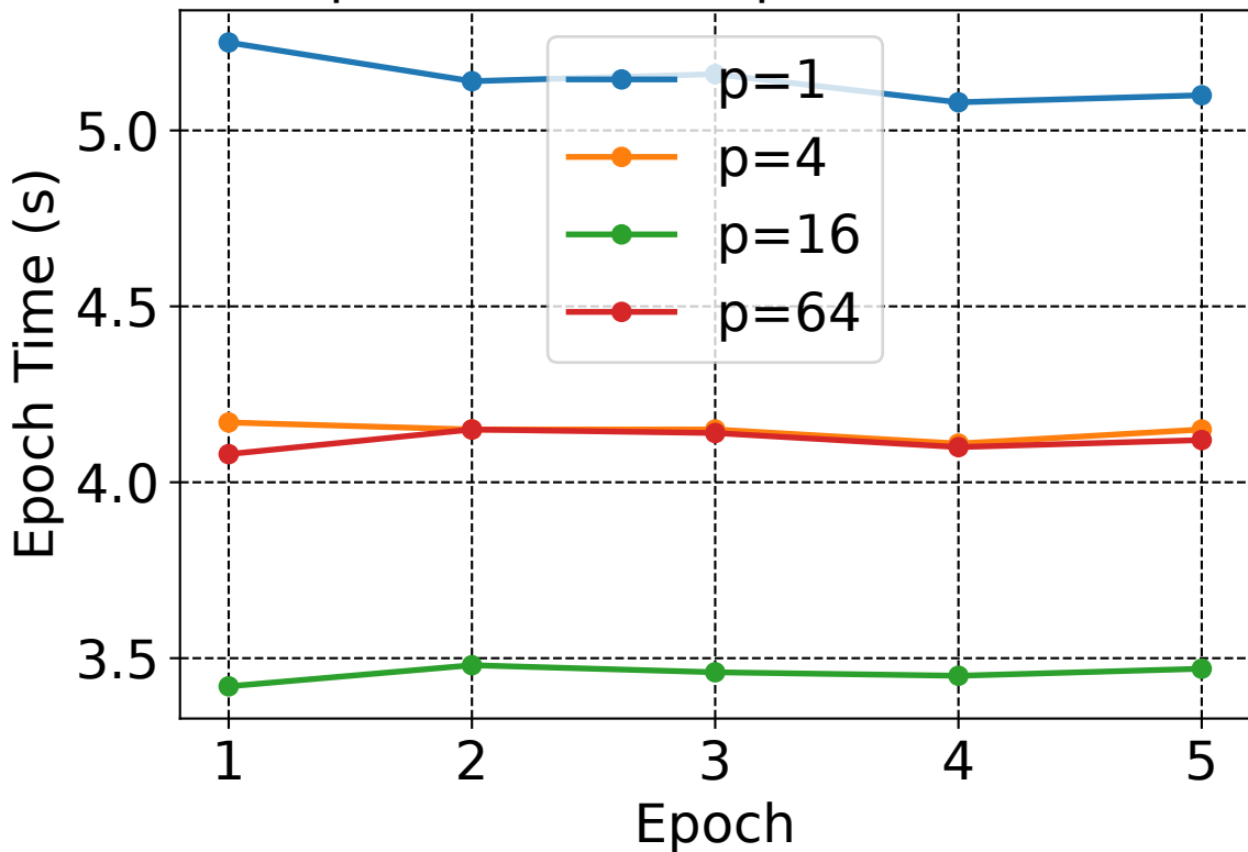
Epoch Time Per Epoch for h=64
