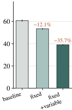
ClickBench
