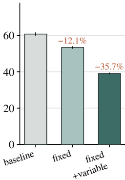
ClickBench 100M
