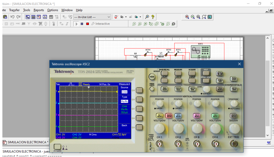
CORRIENTE POR EL INTERRUPTOR
