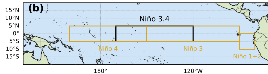
ENSO Region
