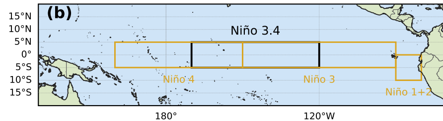
ENSO Region
