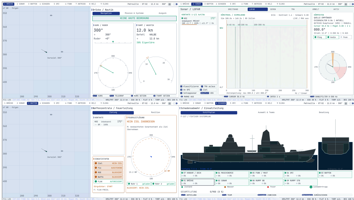
Fregatten-Stationen auf der uConsole: Brücke, Sonar, Waffen und Schadensabwehr
