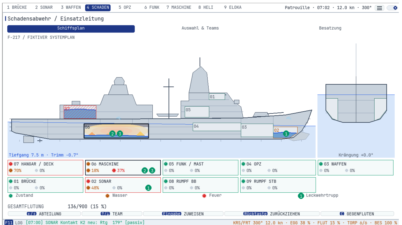
Schadensabwehr mit Wassereintrich und Feuer nach einem Treffer
