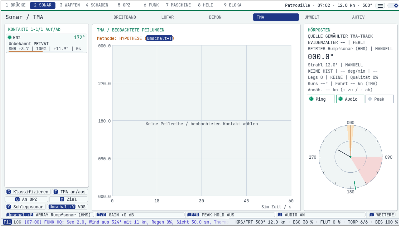
TMA-Seite
