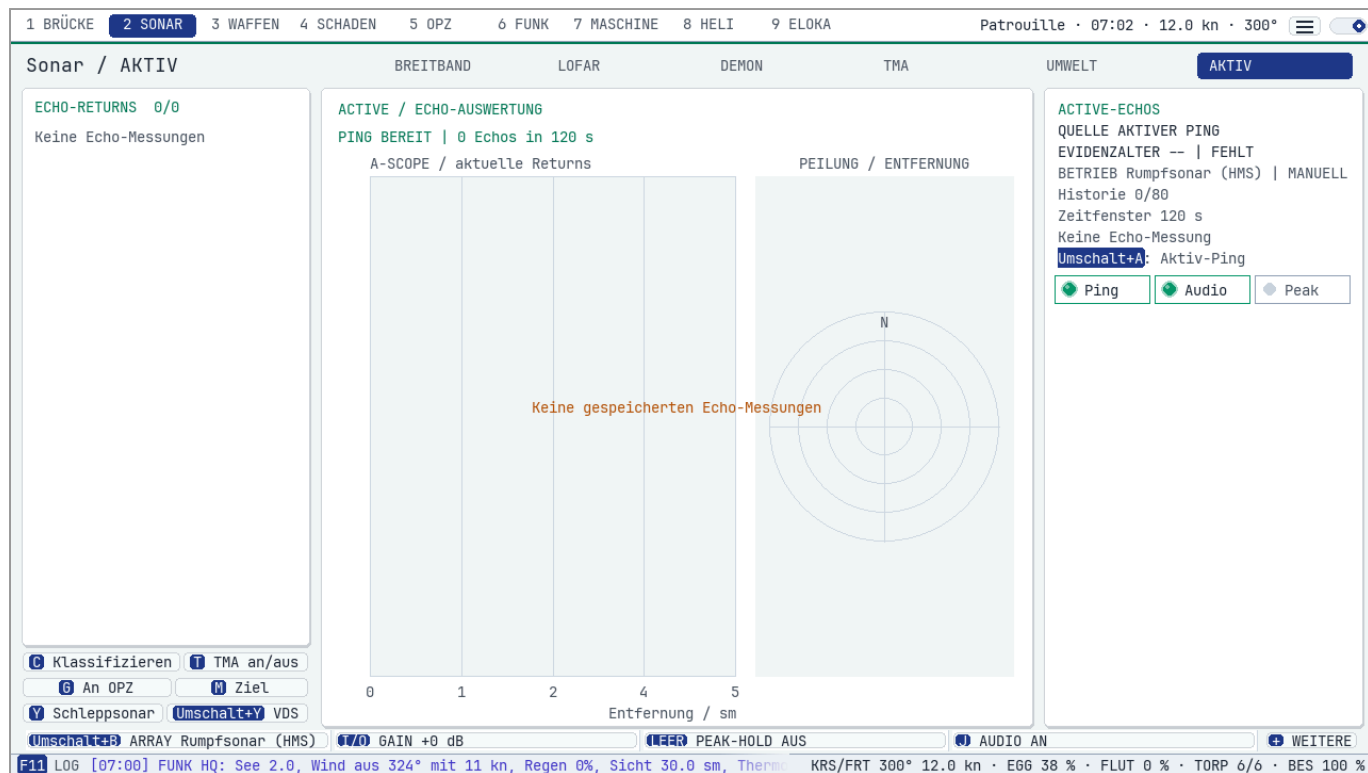
Aktiv-Seite
