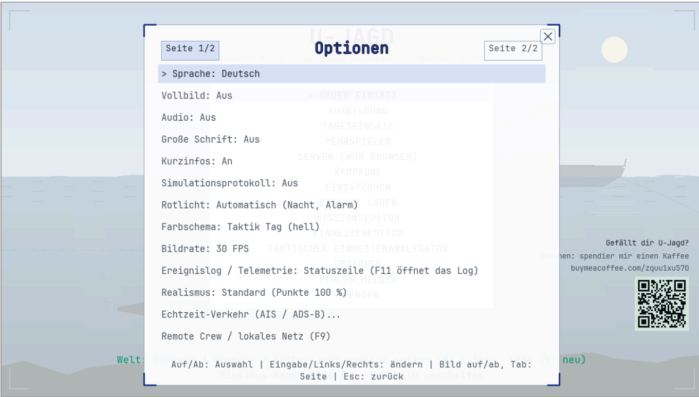
Optionen (F10)
