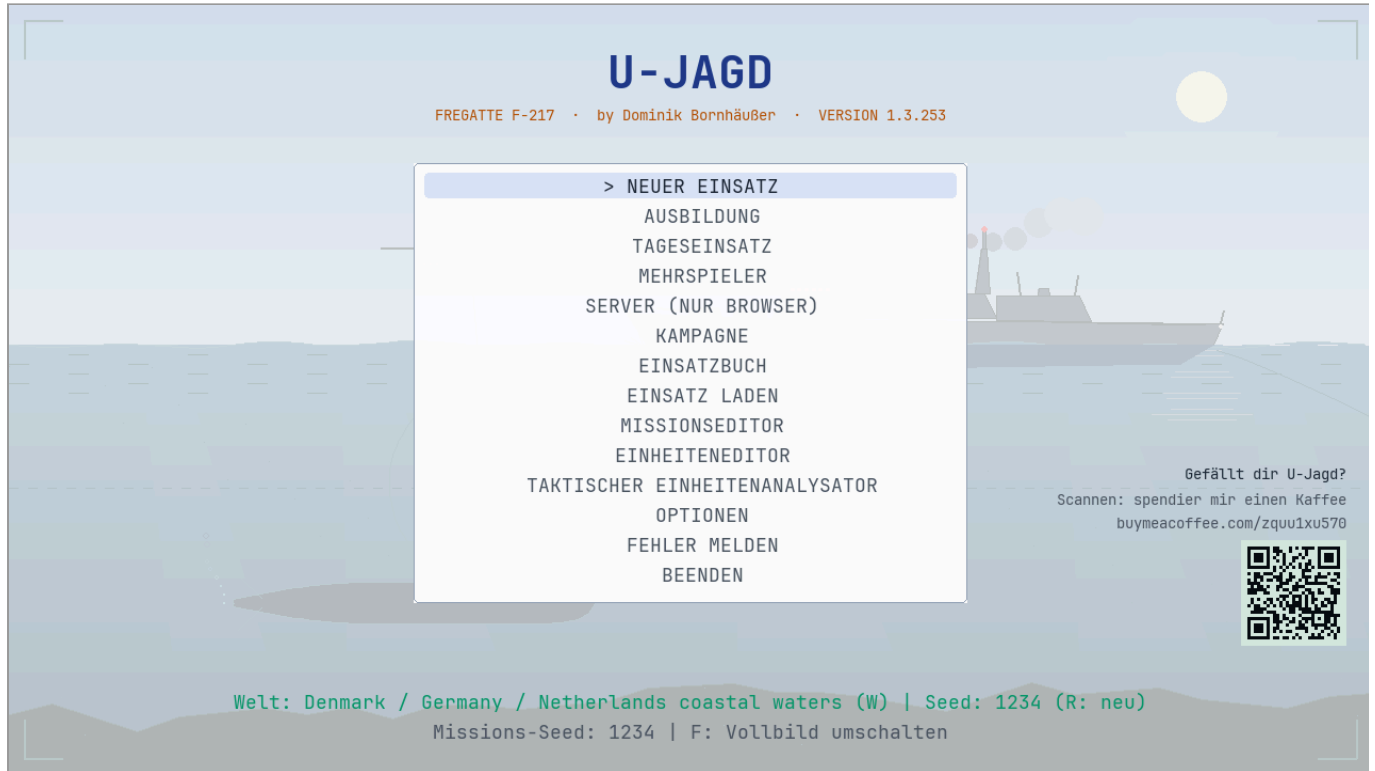
Hauptmenü
