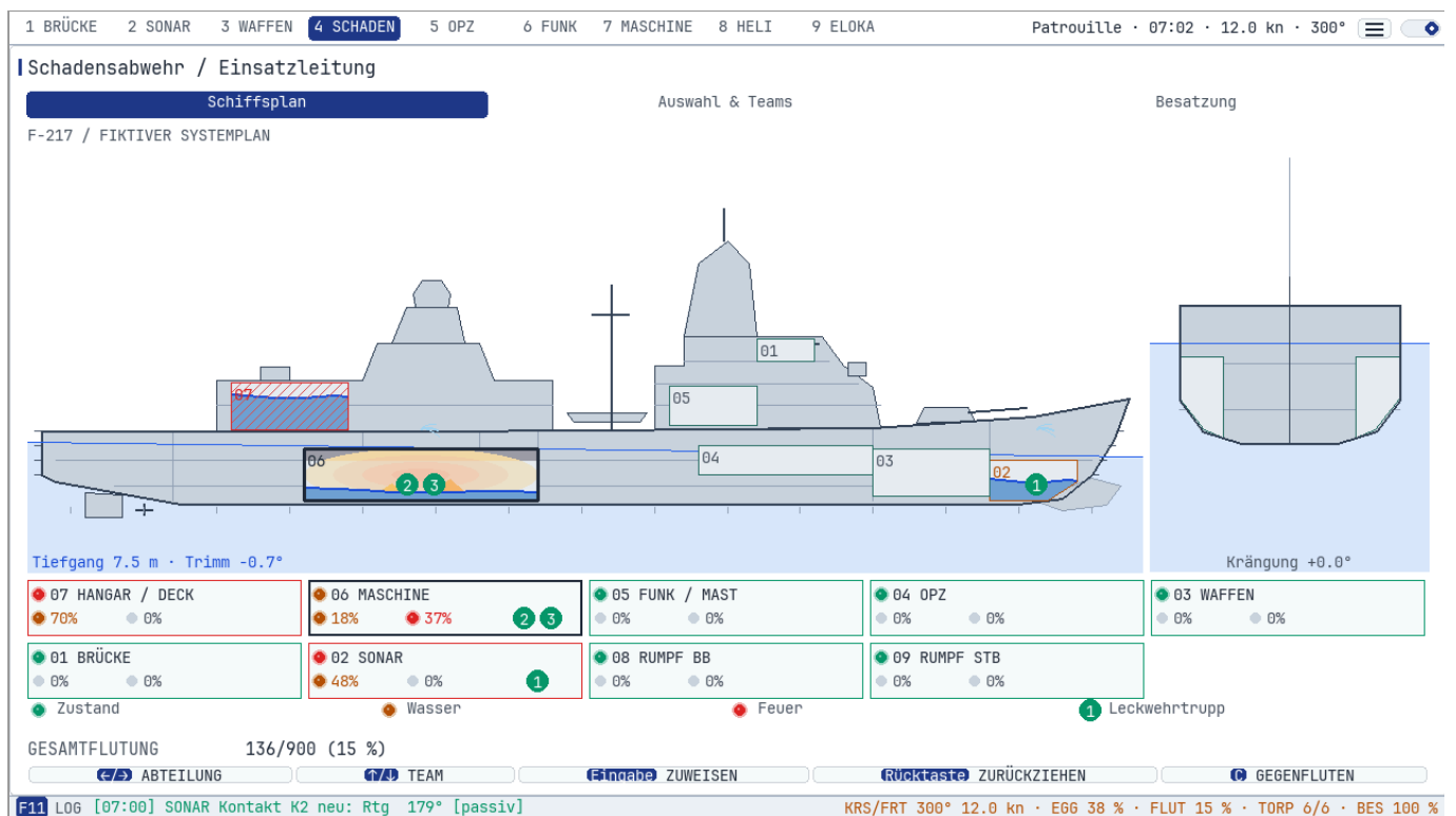
Schadensabwehr mit Wassereintritt und Feuer nach einem Treffer
