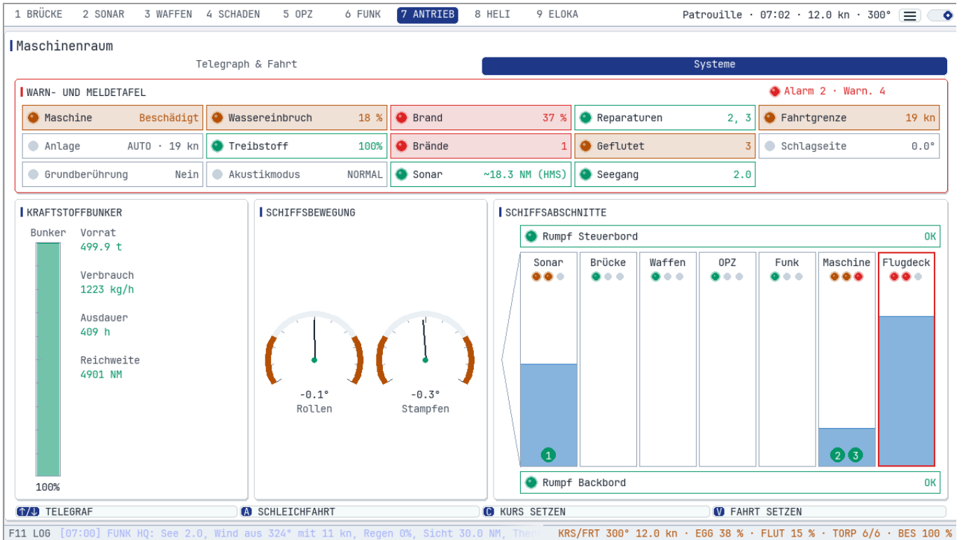
Antrieb, Systemseite
