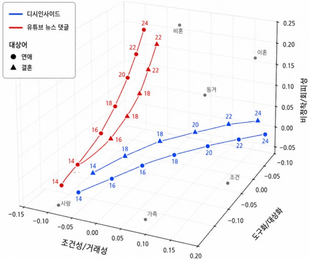
플랫폼별 3차원 의미 이동 경로 예측
