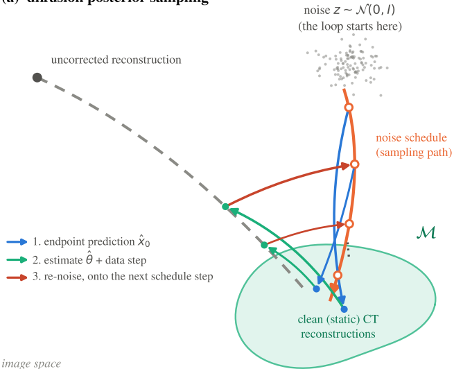
(a) diffusion posterior sampling
