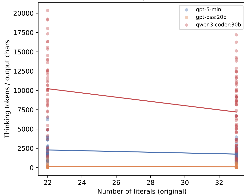
LLM Output Size
