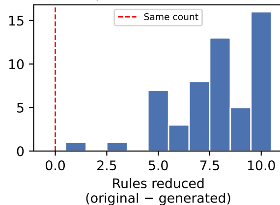
qwen3-coder:30b
