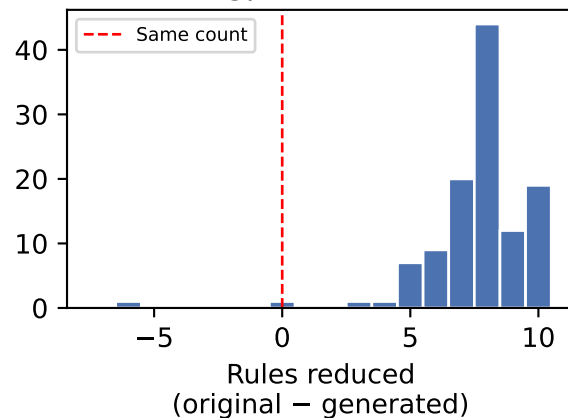
gpt-oss:20b
