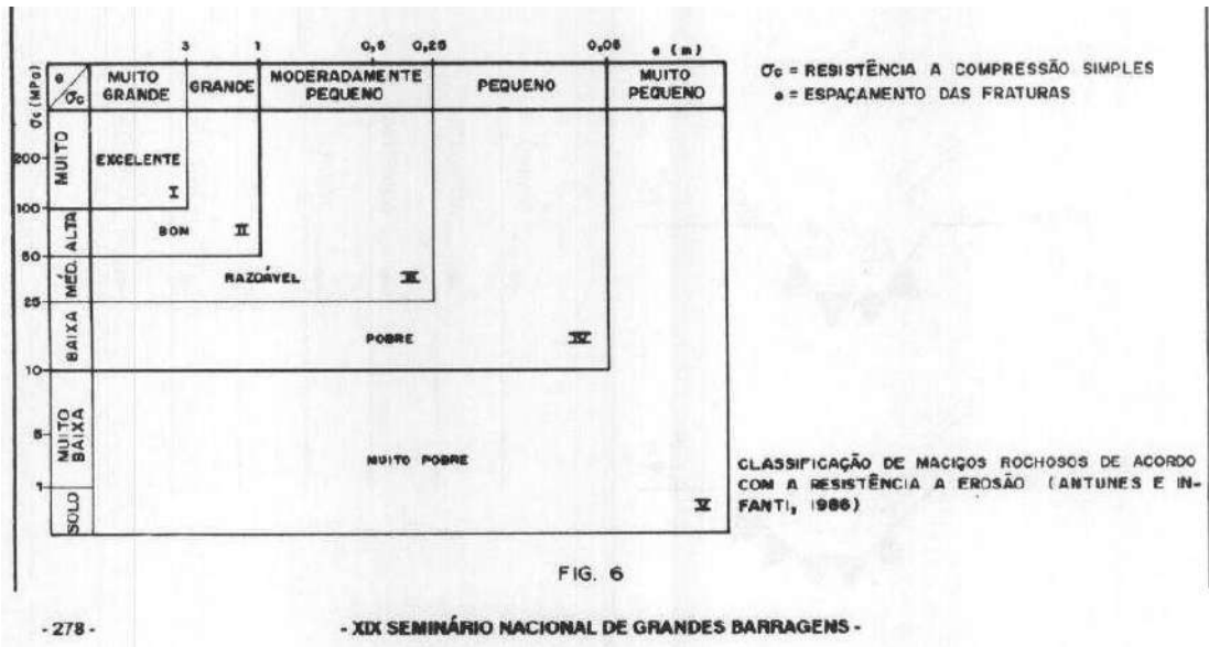
Figura 3.60 – Ábaco de classificação do maciço.
