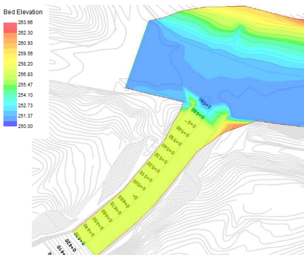
Figura 3.65 - Geometria simulada no modelo River2D: trecho final do canal de restituição da Barragem Norte.
