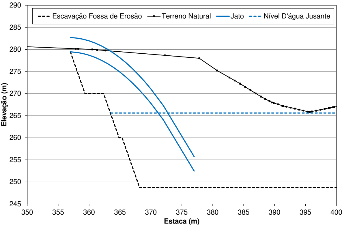
Figura 3.70 – Lançamento do jato na fossa de erosão.
