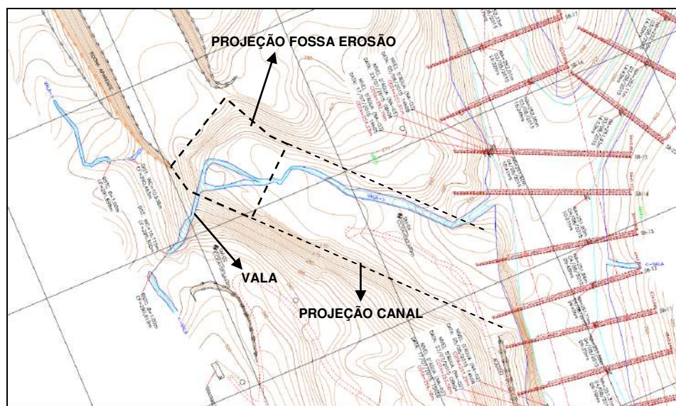
Figura 3.62 – Levantamento topográfico do curso d'água afluente ao canal.
