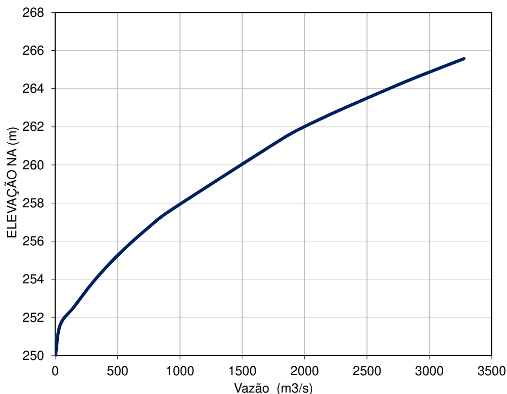
Figura 3.59 – Curva-chave na seção de saída do canal extravasor.
