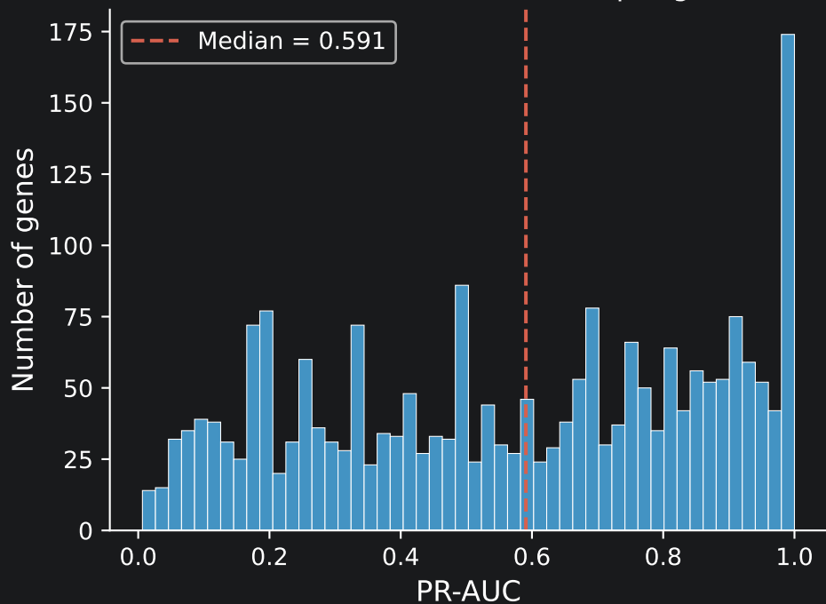
ESM-2 Delta-Norm — PR-AUC per gene
