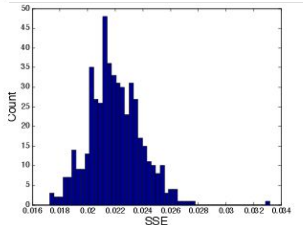
SSE en datos aleatorios
