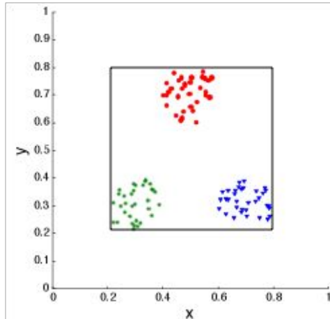
Nuestros datos: SSE = 0.005
