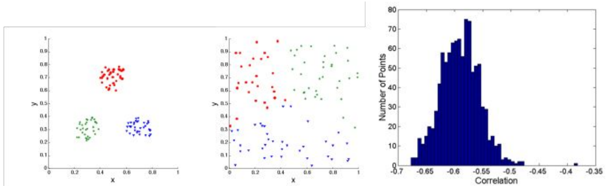
Nuestros datos: Corr= -0.9235
