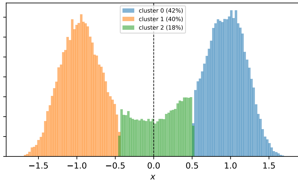
k -means on values
