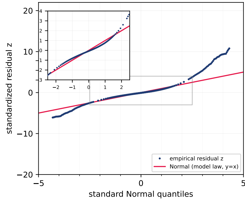
baseline (u+v), L2 ( R^2 N 0.929)
