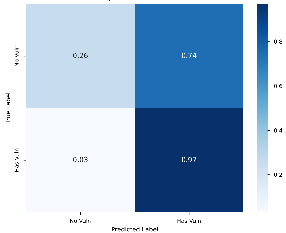
Mistral-7B
