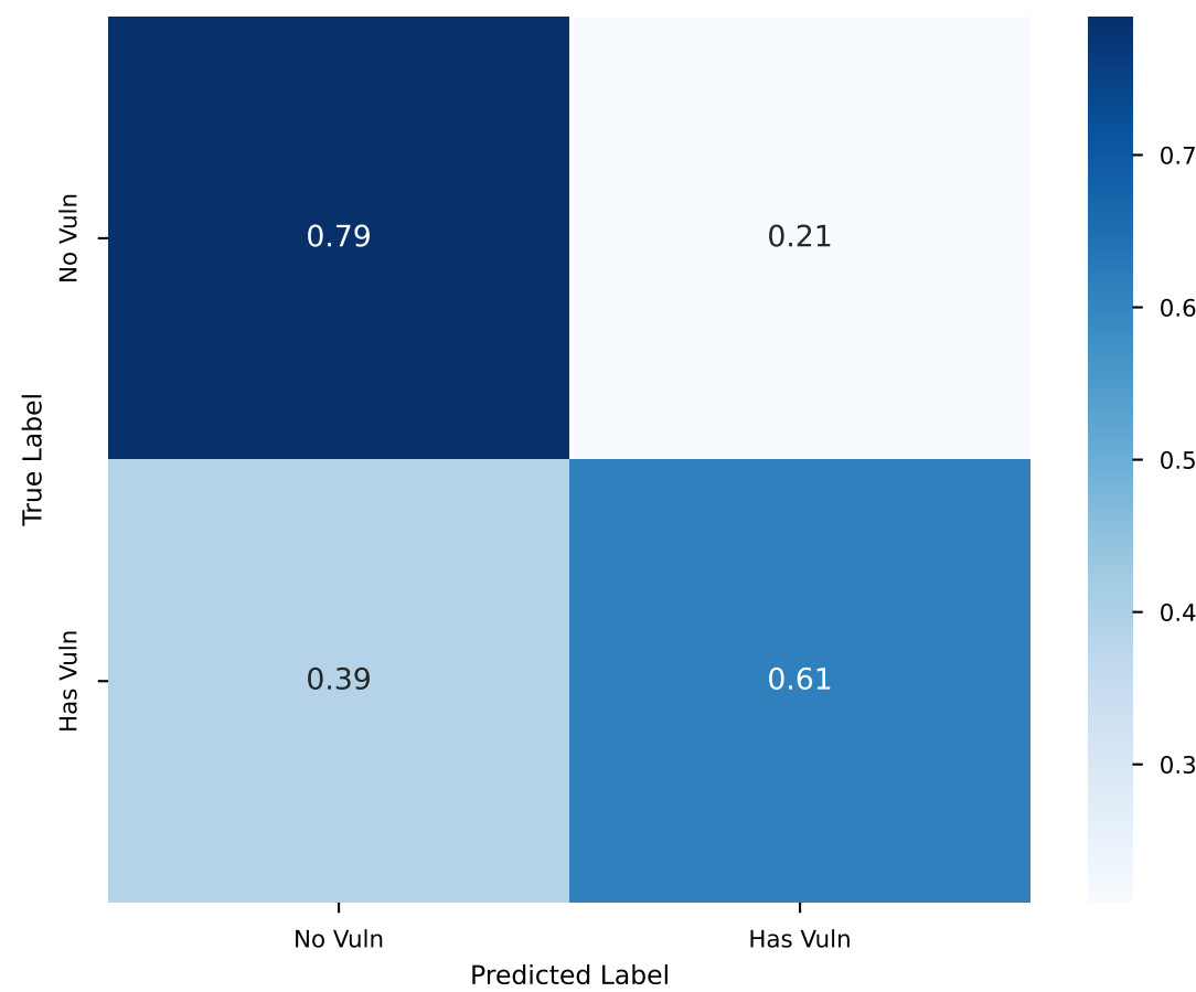
CodeLLaMA-7B
