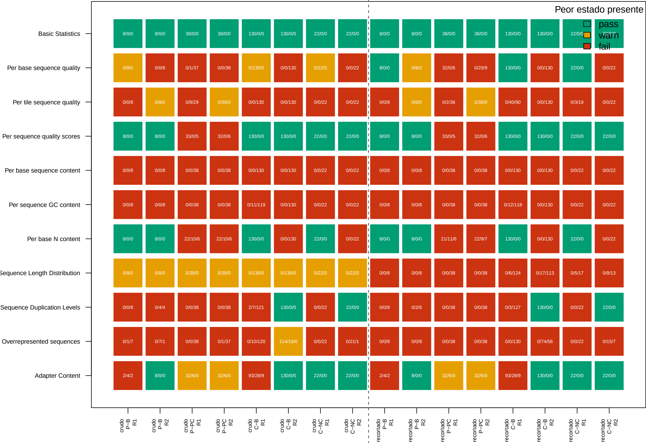
Estados FastQC por módulo (pass / warn / fail)
