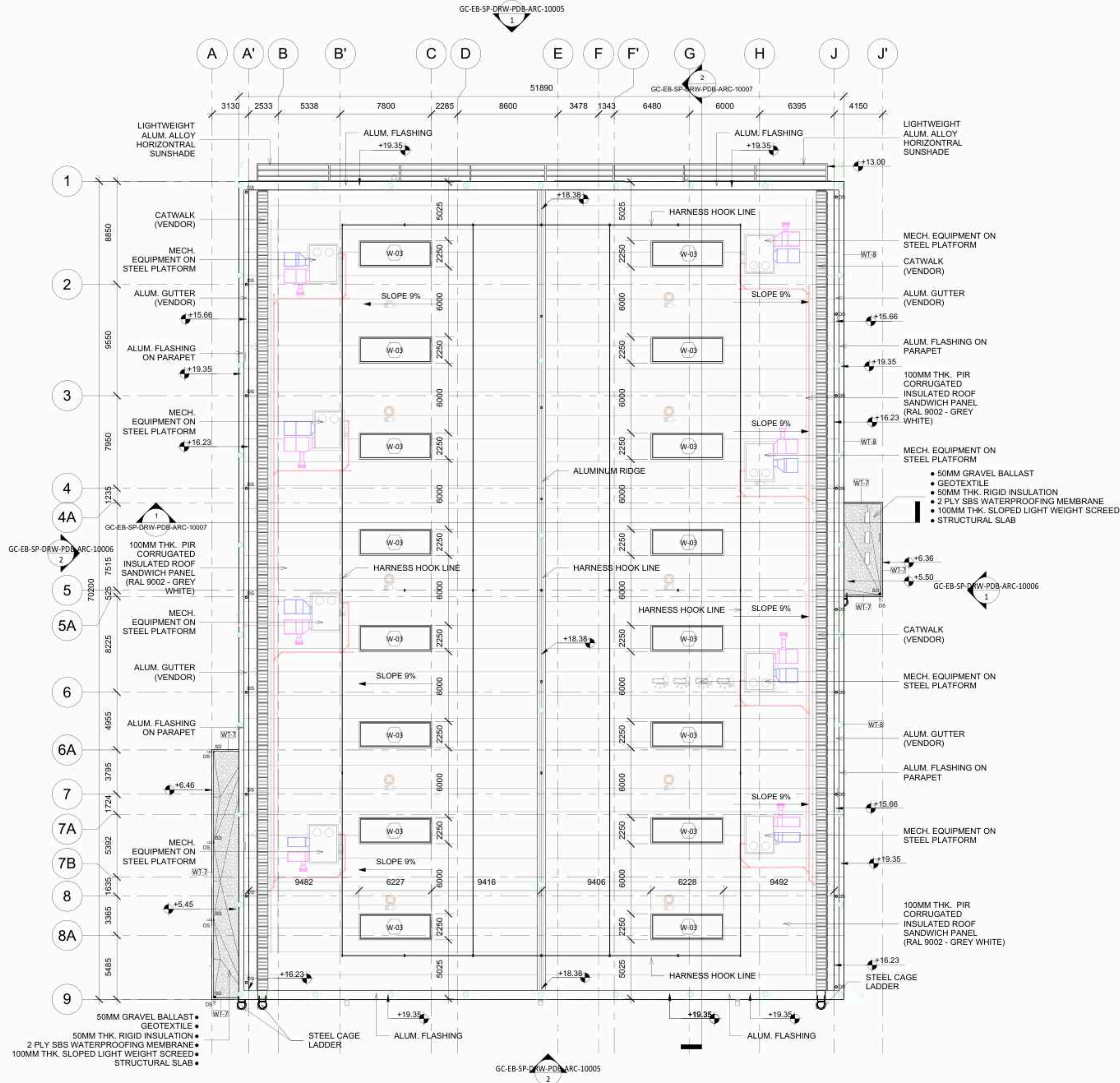
1 ROOF PLAN 1 : 200
