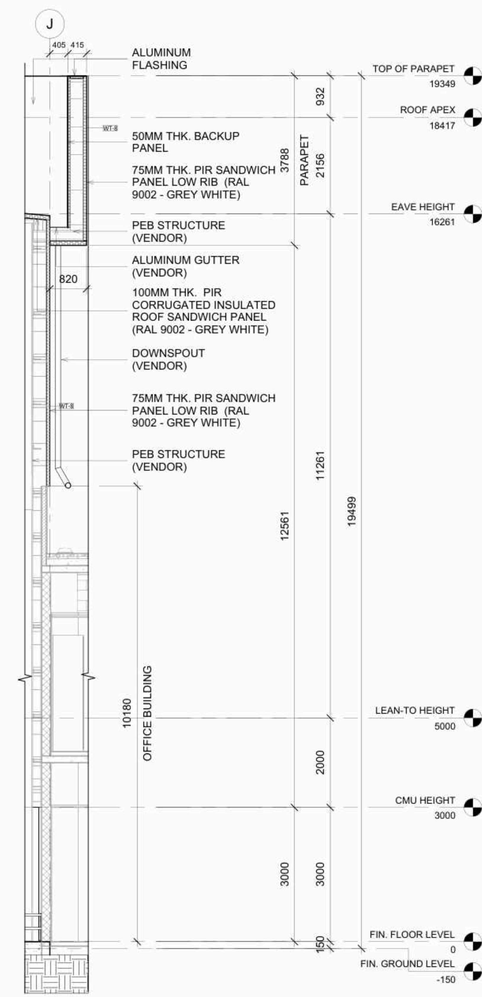
3 WALL SECTION 3 1 : 50
