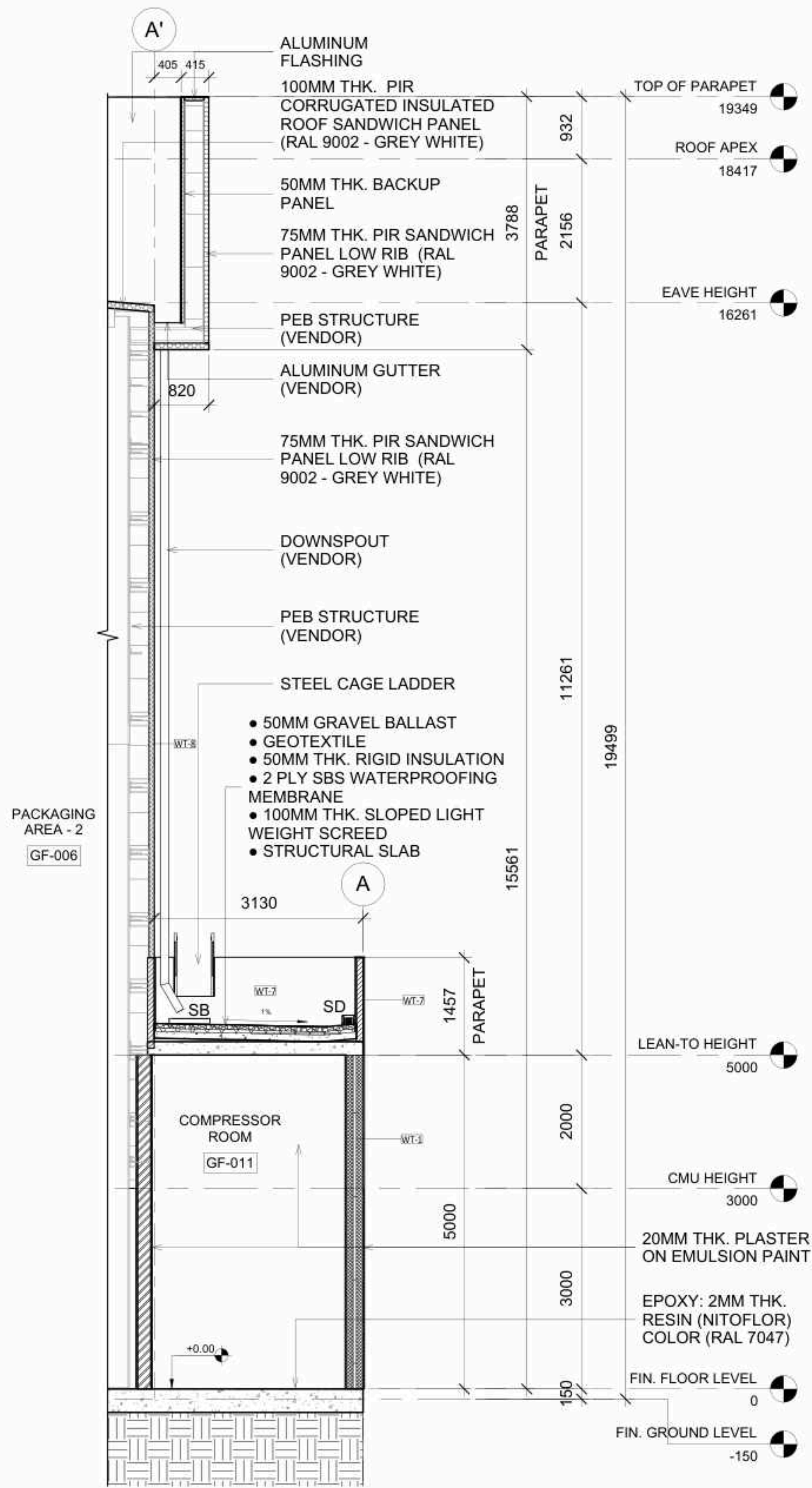
1 WALL SECTION 1 1 : 50
