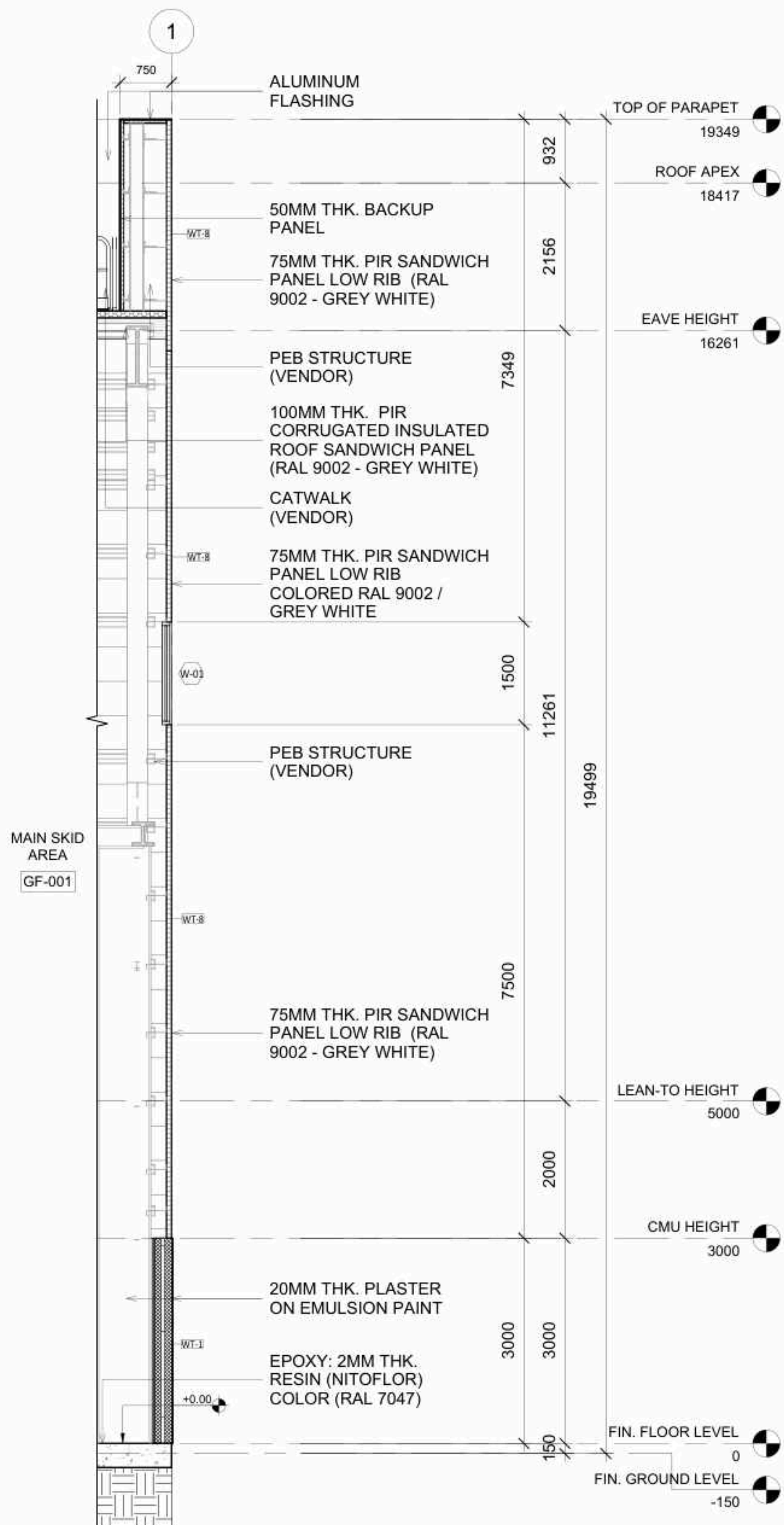
2 WALL SECTION 2 1 : 50
