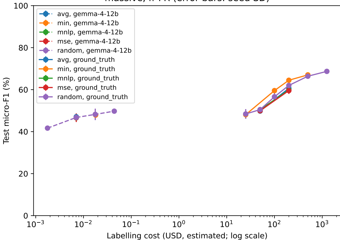
massive, fr-FR (error bars: seed SD)
